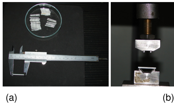
FIG. 63: Ensaio de flexão em quatro pontos, (a) Corpos-de-prova para ensaio e (b) Máquina universal de ensaios com adaptador para ensaio de flexão em quatro pontos. (IME).
