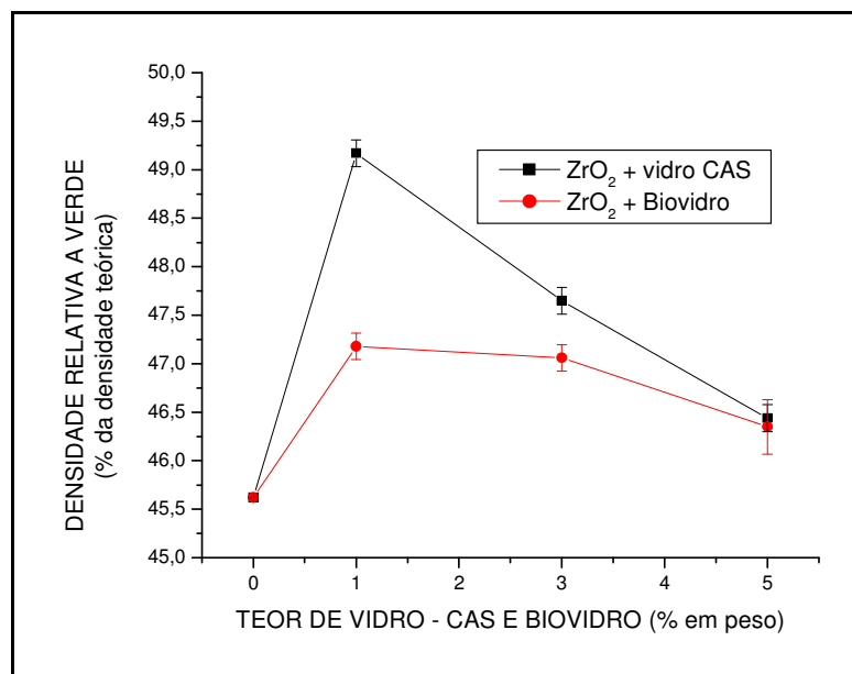
FIG. 76: Efeito da adição de vidro (CAS e Biovidro) na densidade a verde das amostras de zircônia.
