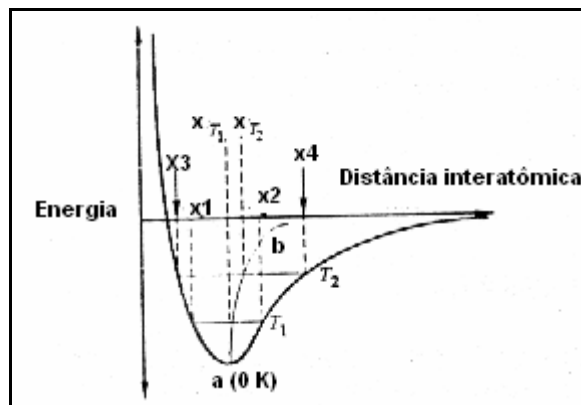
FIG. 50: Efeito do calor na distância interatômica entre os átomos. (BARSOU, 1997).
