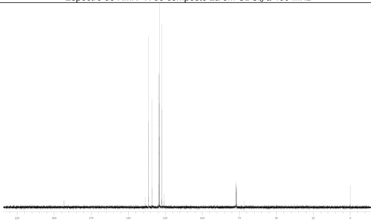
Espectro de RMN ^{13}\text{C} do composto 2a em \text{CDCl}_3 a 100 MHz
