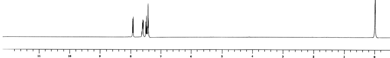
Espectro de RMN ^1\text{H} do composto 2a em \text{CDCl}_3 a 400 MHz
