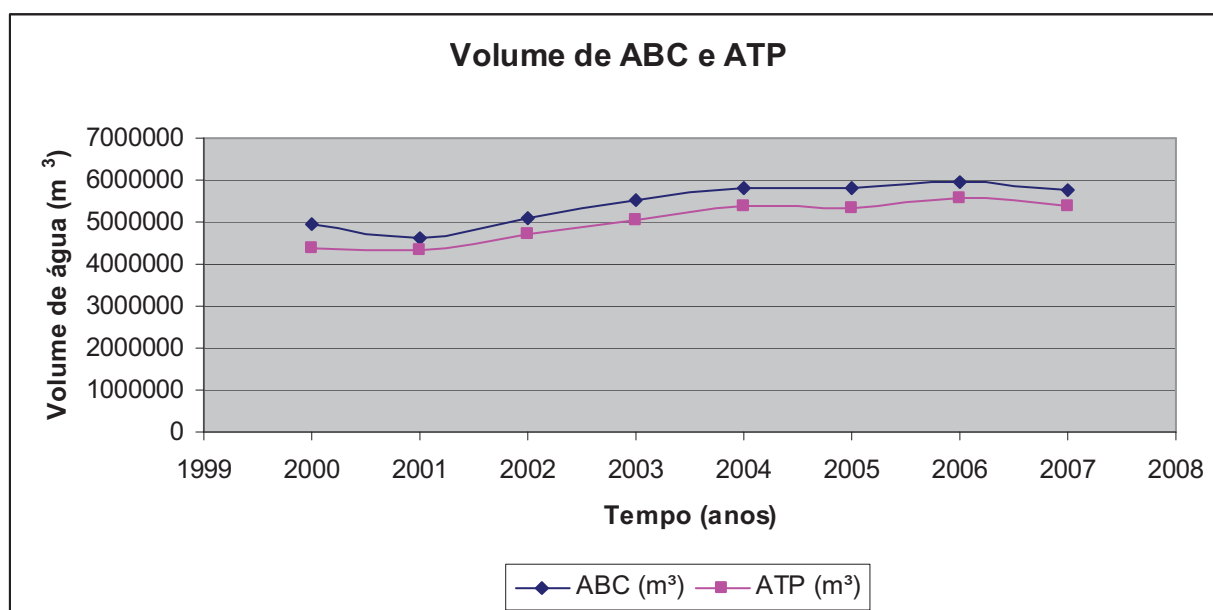
Gráfico 02 – Representação gráfica do volume anual da ABC e ATP do SAA da CORSAN de Lajeado/RS.
