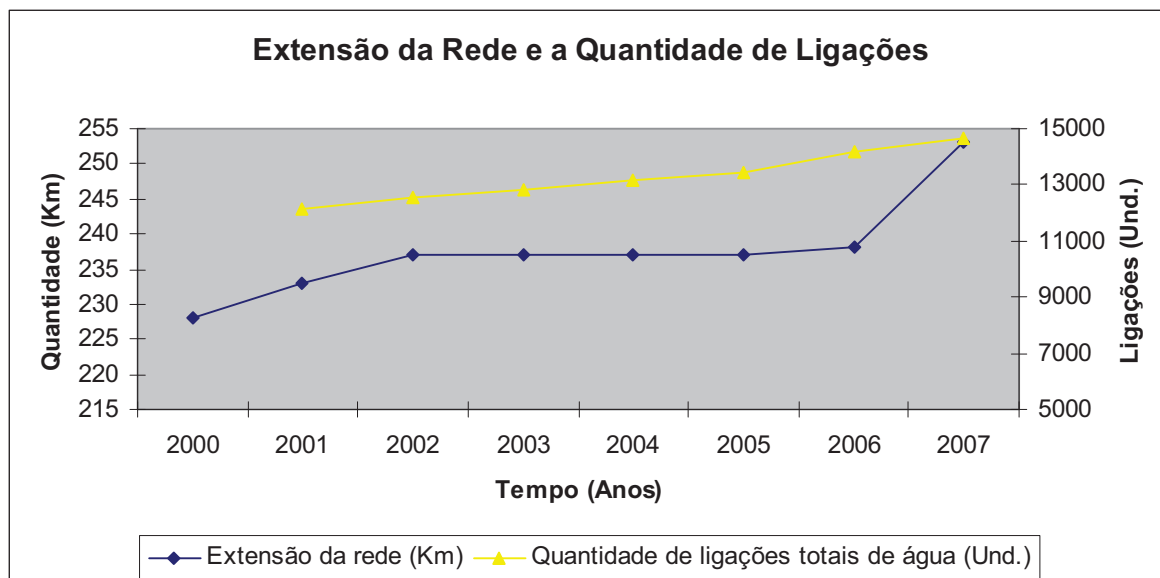
Gráfico 09 – Representação gráfica da extensão da rede de distribuição e da quantidade de ligações de água do SAA da CORSAN de Lajeado/RS.
