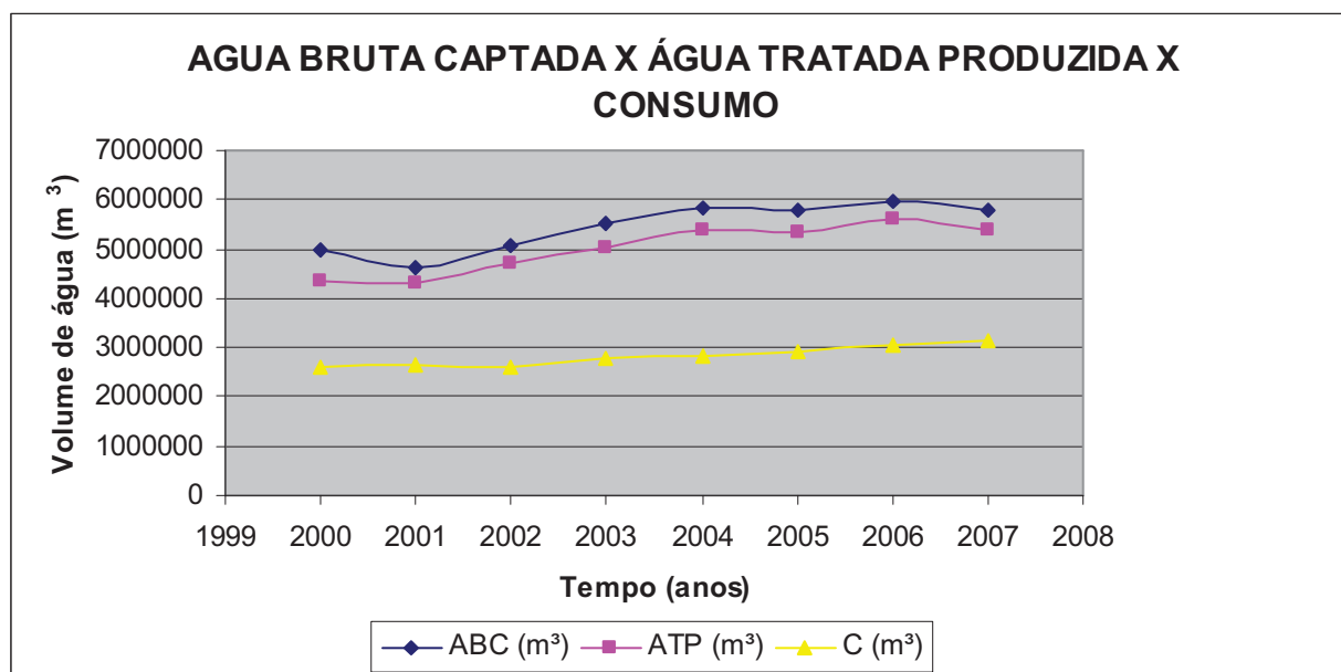
Gráfico 04 – Associação dos volumes de ABC, ATP e C do SAA da CORSAN de Lajeado/RS.
