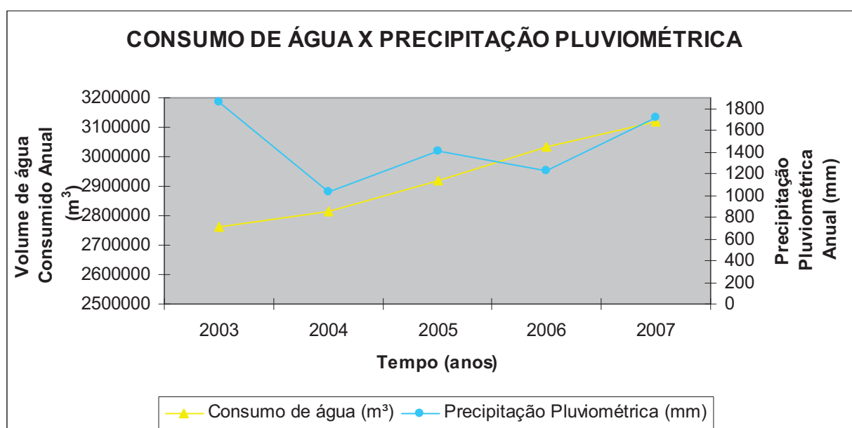
Gráfico 06 – Representação gráfica do volume de C do SAA da CORSAN de Lajeado/RS versus a precipitação pluviométrica total anual de Lajeado/RS.
