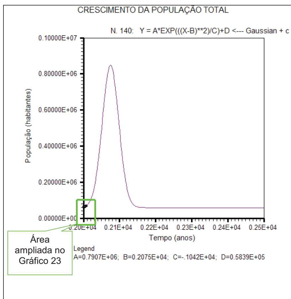
Gráfico 22 – Perfil da curva de ajuste da função número 140 do software LAB Fit Ajuste de Curvas utilizado para previsão do volume de ATP (m 3 ) em função do
