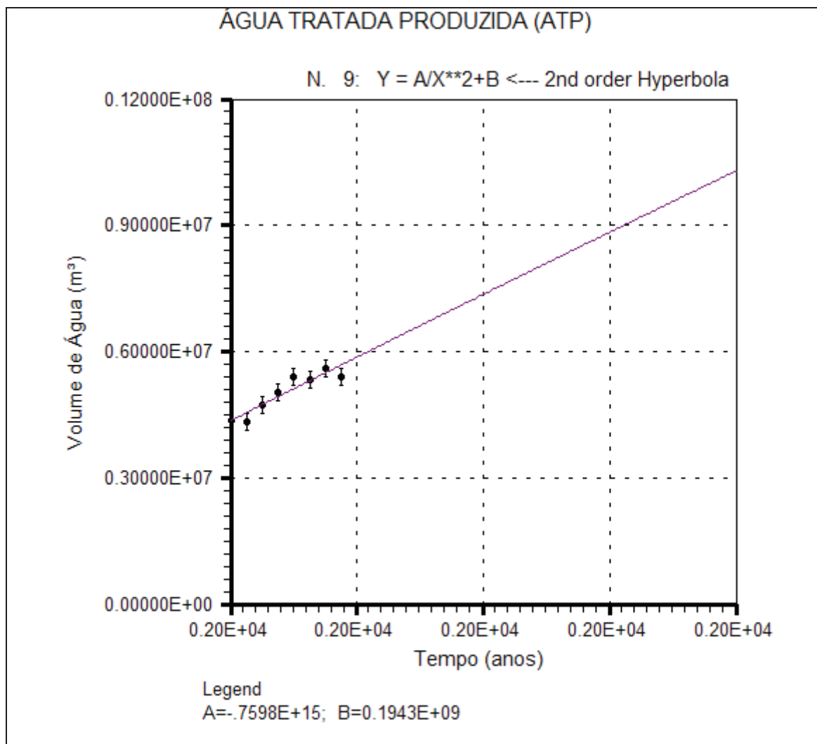
Gráfico 18 – Previsão do volume de ATP (m³) em função do Tempo (anos) através da função número 9 ( y = \frac{A}{X^2} + B ) do software LAB Fit Ajuste de Curvas, considerando-se a série temporal efetiva de 2000 e 2007, e a previsão a partir destes pontos efetivos a partir de 2008.
