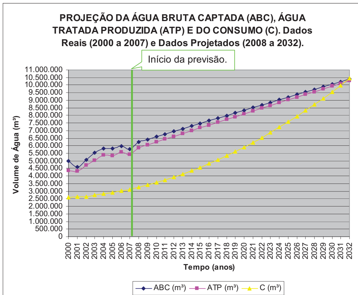
Gráfico 21 – Série temporal efetiva do volume de ABC, ATP e do C, entre 2000 e 2007, e a previsão da série temporal pela função de números 9 onde sua fórmula é
