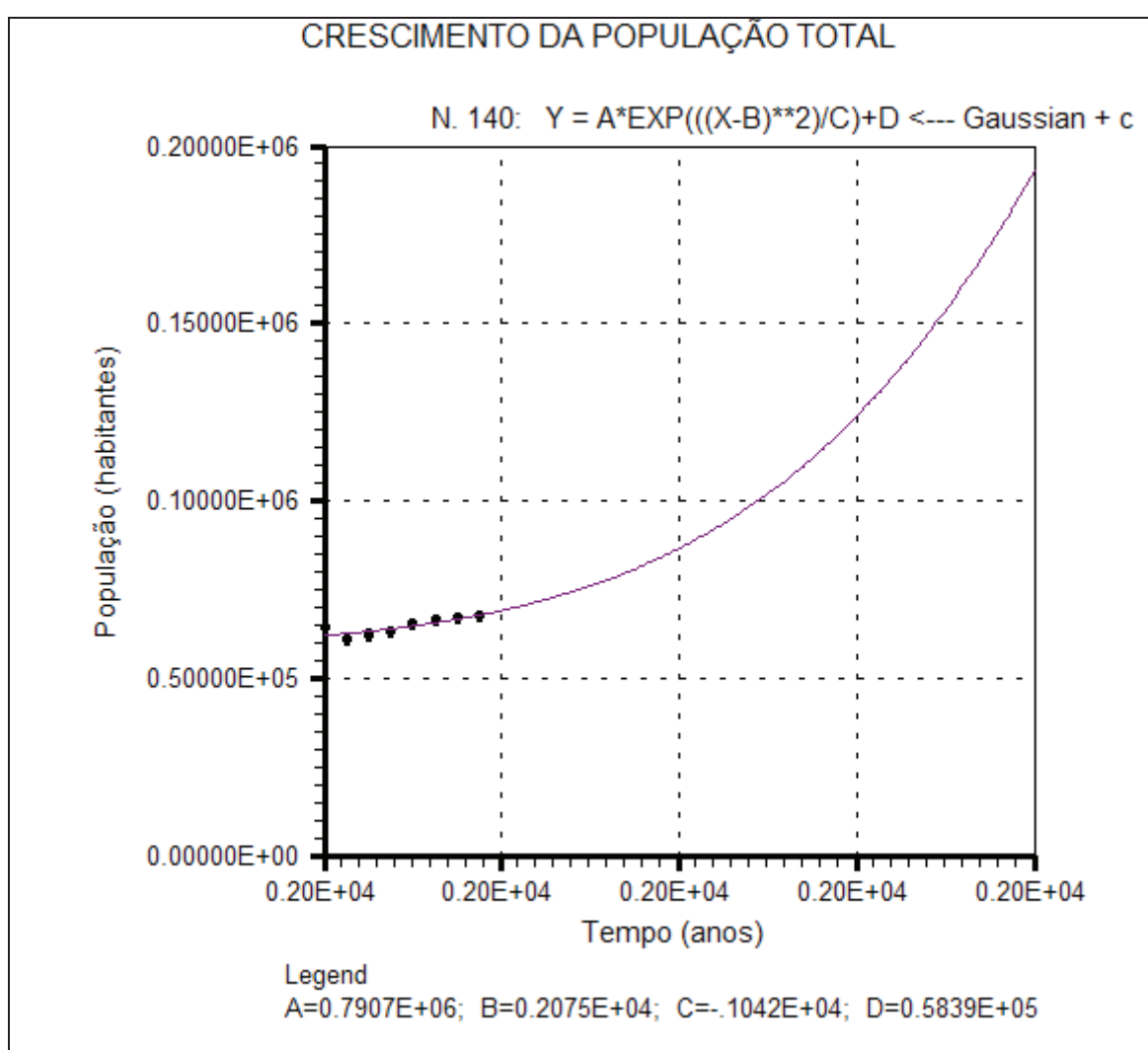
Gráfico 23 – Previsão da população total (habitantes) em função do tempo (anos) através do software LAB Fit Ajuste de Curvas onde a função é de número 140
