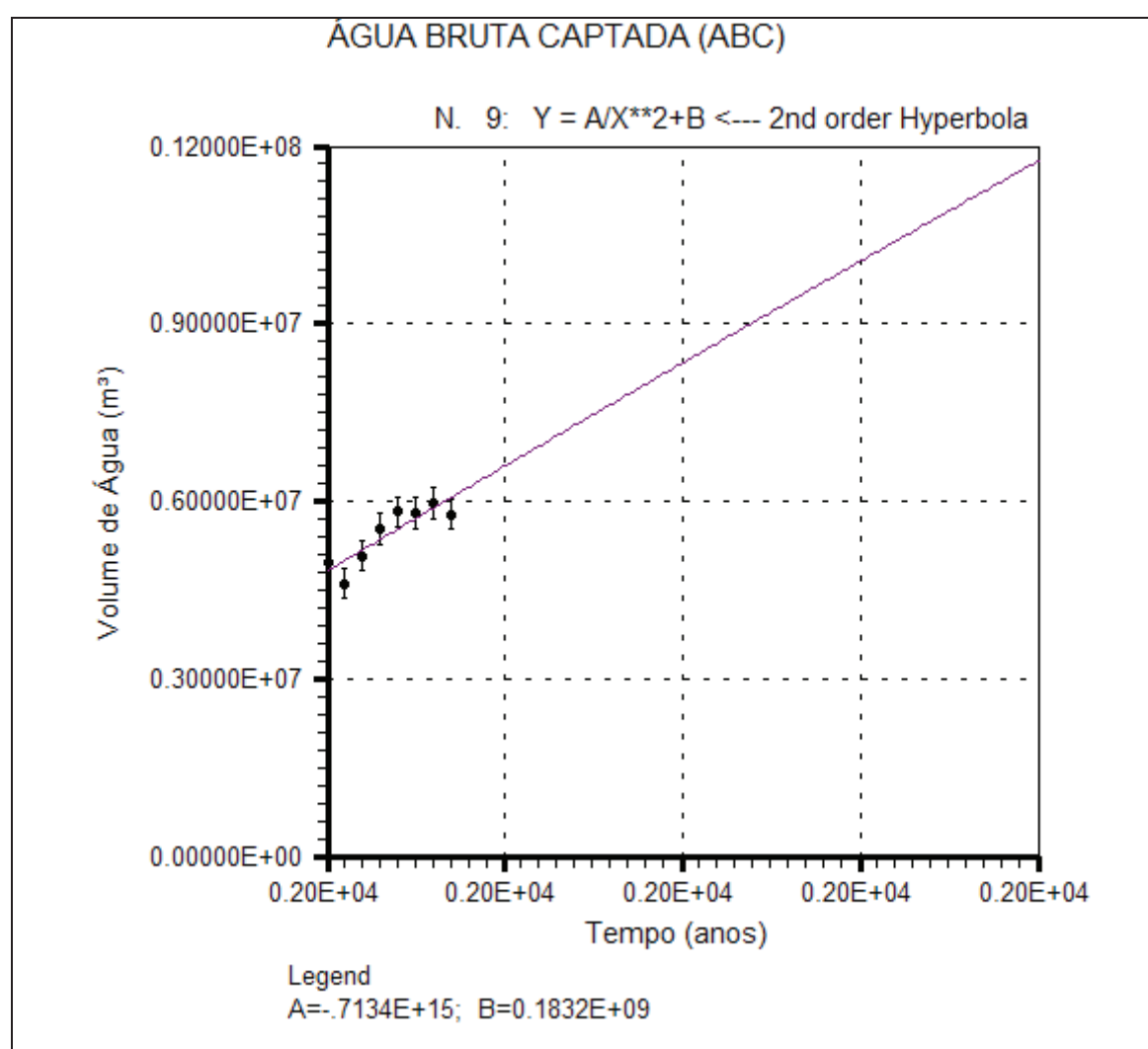
Gráfico 16 - Previsão do volume de ABC (m³) em função do tempo (anos) através da função número 9 onde sua fórmula é y = \frac{A}{X^2} + B do software LAB Fit Ajuste de Curvas, considerando-se a série temporal efetiva de 2000 e 2007, e a previsão a partir destes pontos efetivos a partir de 2008.
