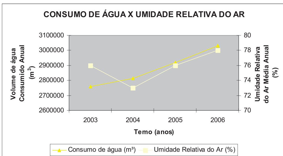
Gráfico 07 – Representação gráfica do volume de C do SAA da CORSAN de Lajeado/RS versus o percentual de umidade relativa do ar média anual de Lajeado/RS.
