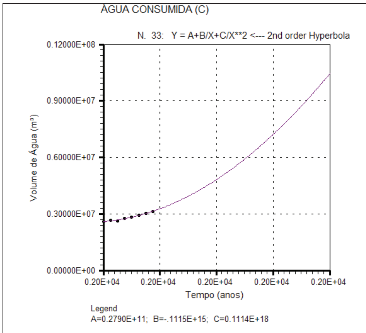
Gráfico 20 – Previsão do volume de C (m 3 ) em função do tempo (anos) através da função número 33 onde sua fórmula é y = A + \frac{B}{X} + \frac{C}{X^2} do software LAB Fit Ajuste de Curvas, considerando-se a série temporal efetiva de 2000 e 2007, e a linha de regressão entre 2008 e 2032.
