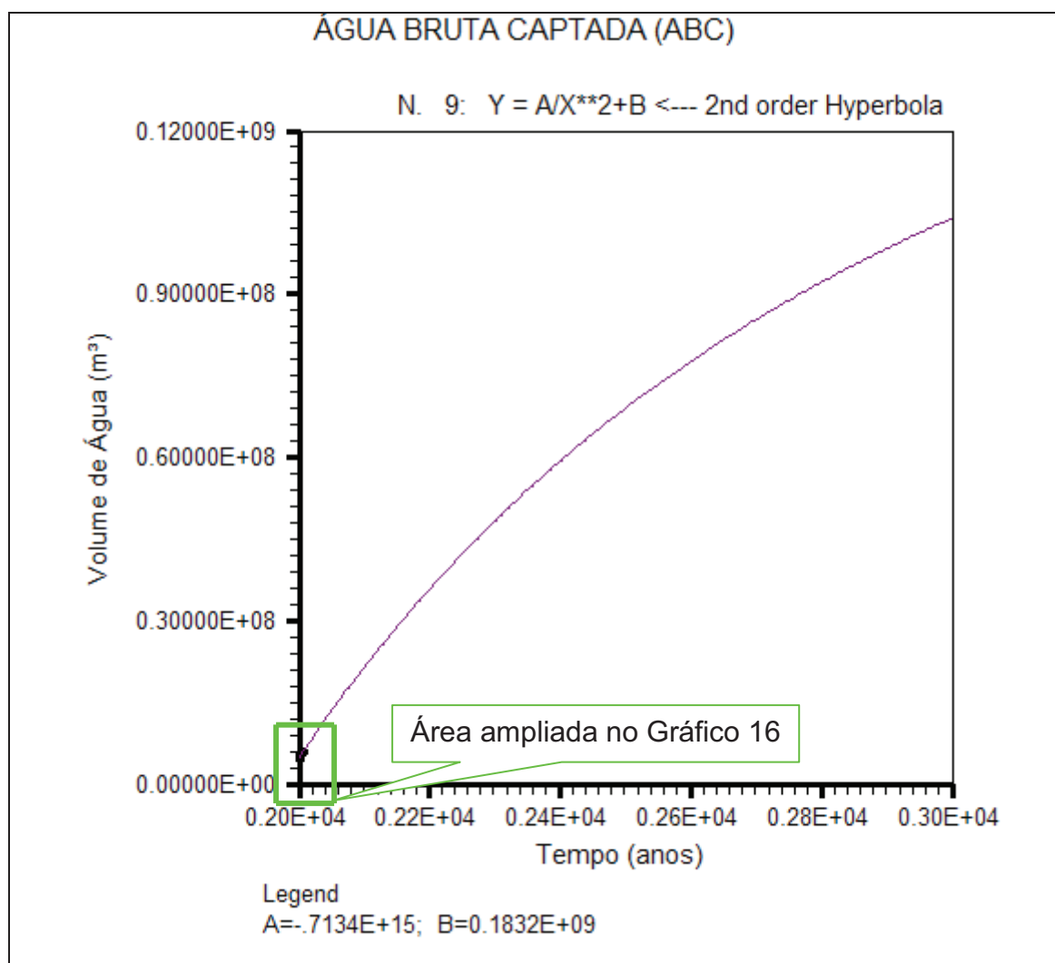
Gráfico 15 – Perfil da curva de ajuste da função número 9 do software LAB Fit Ajuste de Curvas utilizado para previsão do volume de ABC (m 3 ) em função do tempo (anos), onde sua fórmula é y = \frac{A}{X^2} + B e o valor de A = -.7134E+15 e de B = 0.1832E+09 .
