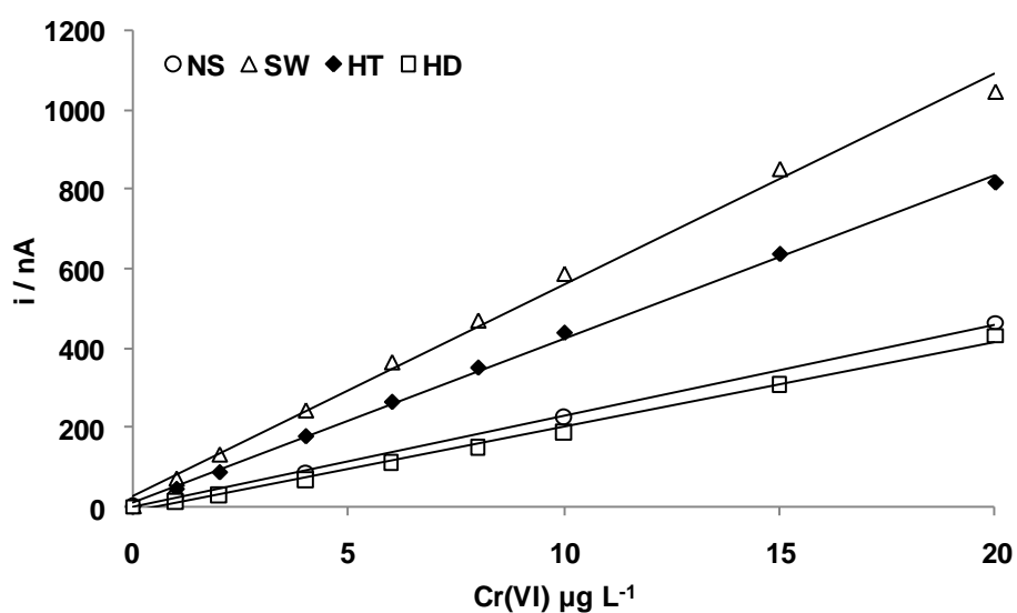
Figura 32 - Curvas de calibração para a faixa Cr(VI) 1,0 a 20,0 \mu\text{g L}^{-1} . Solução de medida: 10 mL solução-teste + 2,5 mL eletrólito (DTPA 0,05 mol \text{L}^{-1} , \text{NaNO}_3 2,5 mol \text{L}^{-1} e \text{CH}_3\text{COONa} 0,20 mol \text{L}^{-1} ). pH 6,2 \pm 0,1. AdSV. Tempo de deposição: 20 s. Amplitude de pulso: -50 mV (voltametria de pulso diferencial).
