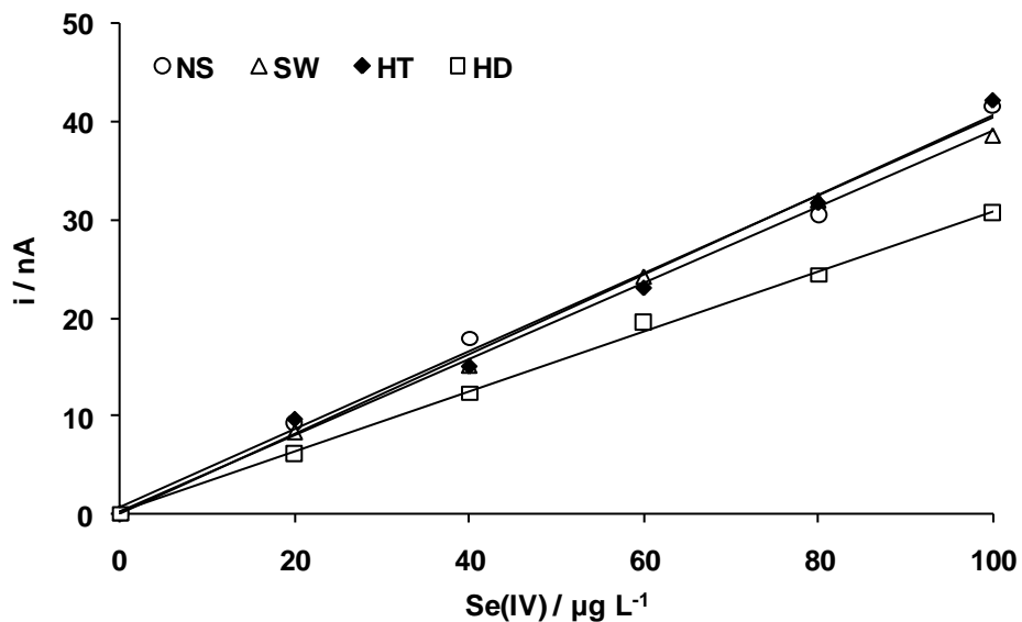
Figura 9 - Curvas de calibração para a faixa Se(IV) 20,0 a 100,0 \mu\text{g L}^{-1} . Solução de medida: 10 mL solução-teste + Cu(II) 1,0 \text{mg L}^{-1} + HCl 0,1 \text{mol L}^{-1} . Potencial de deposição: -300\text{ mV} . Tempo de deposição: 10 s. Amplitude de pulso: -50\text{ mV} (voltametria de pulso diferencial).
