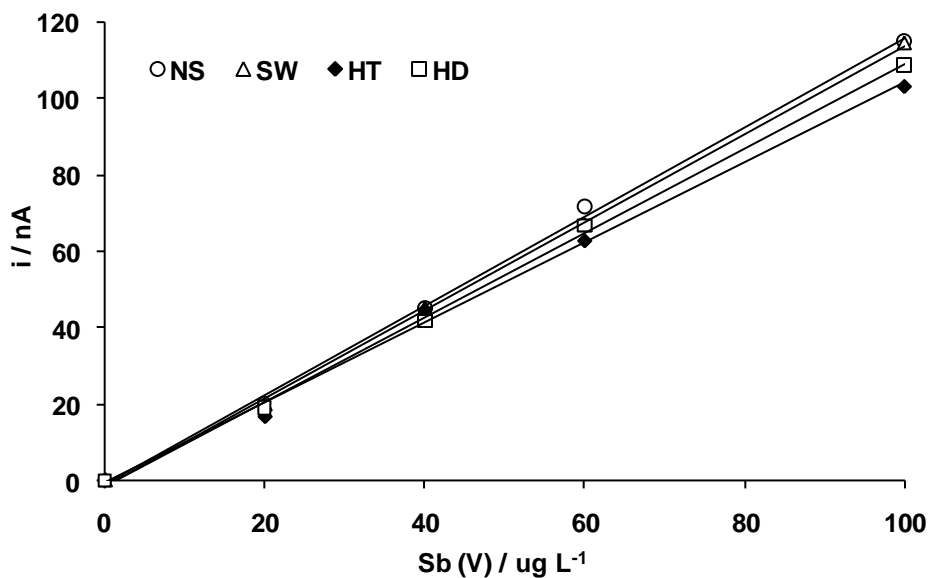
Figura 23 - Curvas de calibração para a faixa Sb(V) 20,0 a 100,0 \mu\text{g L}^{-1} . Solução de medida: 10 mL solução-teste + HCl 5,0 mol \text{L}^{-1} . ASV. Potencial de deposição: -400 mV. Tempo de deposição: 10-30 s. Amplitude de pulso: 25 mV (voltametria de pulso diferencial).
