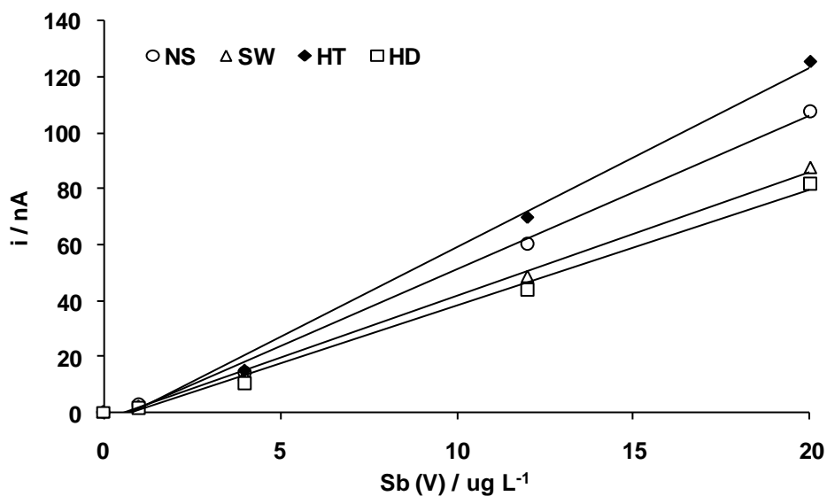
Figura 22 - Curvas de calibração para a faixa Sb(V) 1,0 a 20,0 \mu\text{g L}^{-1} . Solução de medida: 10 mL solução-teste + HCl 5,0 mol \text{L}^{-1} . ASV. Potencial de deposição: -400 mV. Tempo de deposição: 90-120 s. Amplitude de pulso: 25 mV (voltametria de pulso diferencial).
