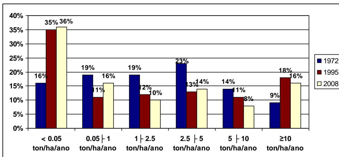
Gráfico 12 - A Variação da Distribuição das Classes de Perdas de Solo na Bacia do Ribeirão Alam Grei, em porcentagem (%), nos anos de 1972, 1995 e 2008.
