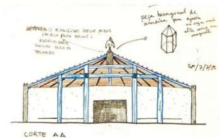
FIGURA 73 – Estudo da estrutura do telhado da capela.
