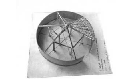
FIGURA 75 – Maquete da estrutura do telhado da capela.
