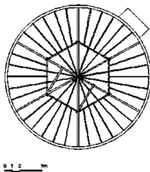
FIGURA 64 – Diagrama da cobertura.
