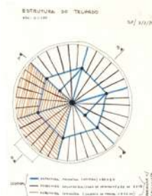
FIGURA 74 – Diagrama da estrutura do telhado da capela.
