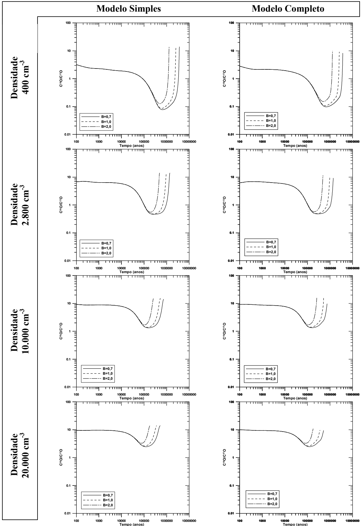
Figuras 5.3b: Comparação da razão C^{18}O/C^{17}O para os diferentes valores de B utilizados nos modelos simples e completo (colapso - sem grãos).
