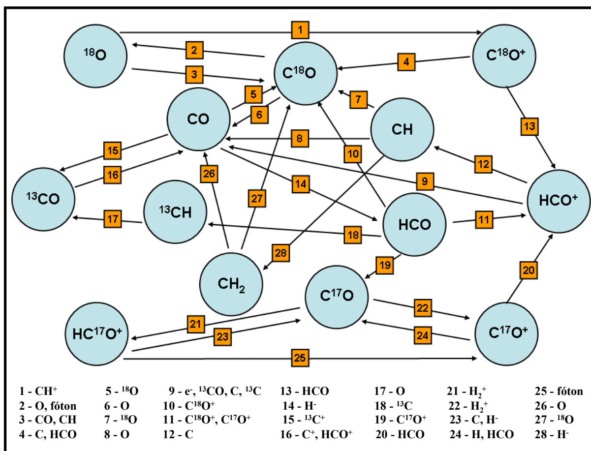
Figura 5.5: Diagrama esquemático das reações mais importantes dos modelos de colapso e puramente químico.
