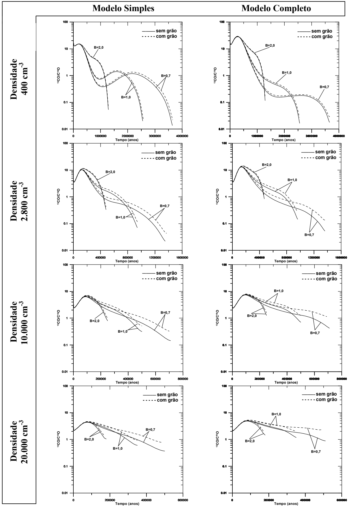
Figuras 5.4a: Razões ^{13}\text{CO}/^{18}\text{O} para os modelos simples e completo comparando-se os modelos de colapso sem e com grãos e para os diferentes valores de B utilizados.
