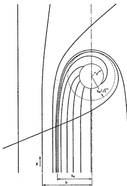
Figura B.1: Ilustração da colisão de um íon com uma molécula neutra. Fonte: GIOUMOUSIS; STEVENSON, 1958.
