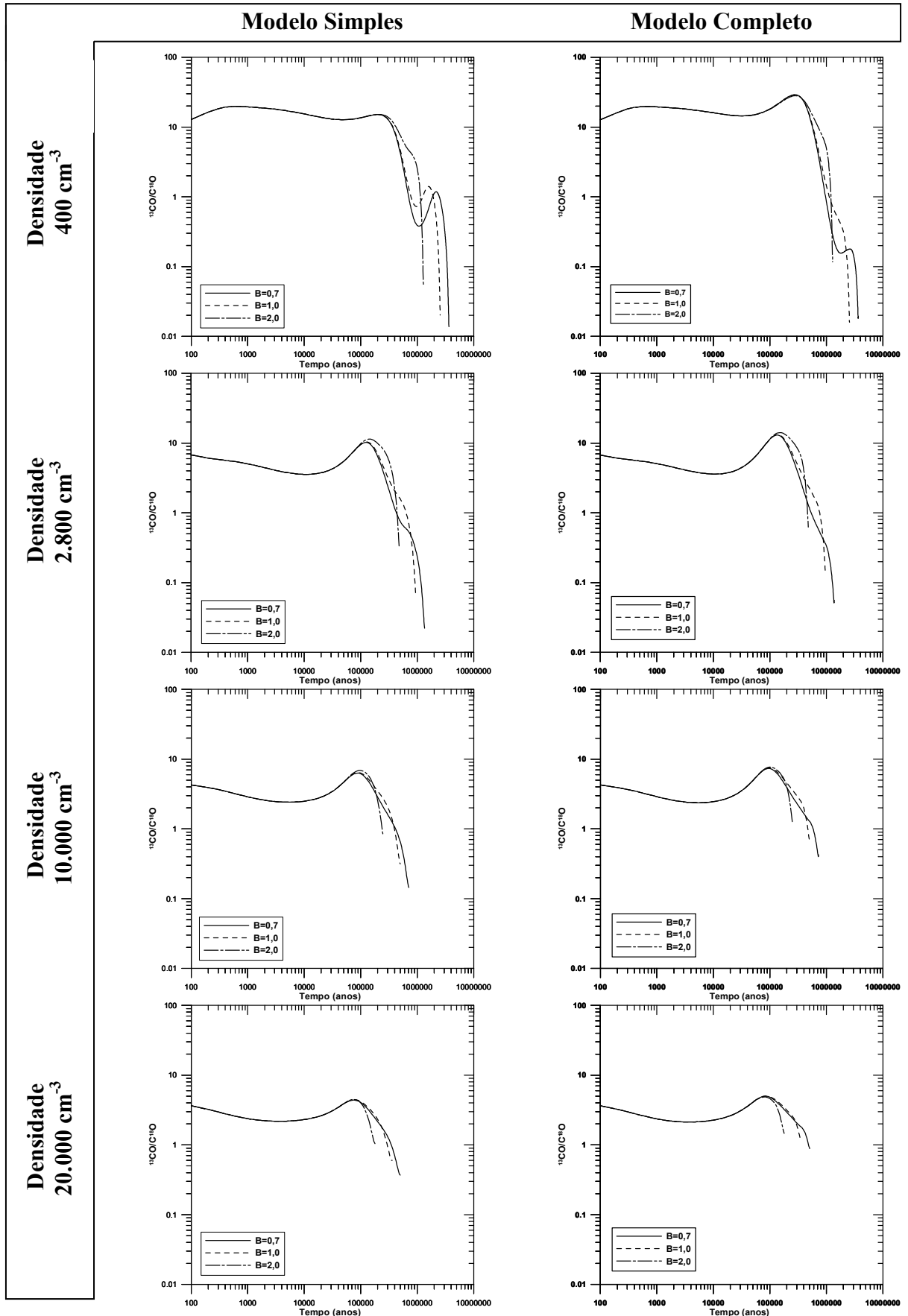
Figuras 5.3a: Comparação da razão ^{13}\text{CO}/^{18}\text{O} para os diferentes valores de B utilizados nos modelos simples e completo (colapso - sem grãos).
