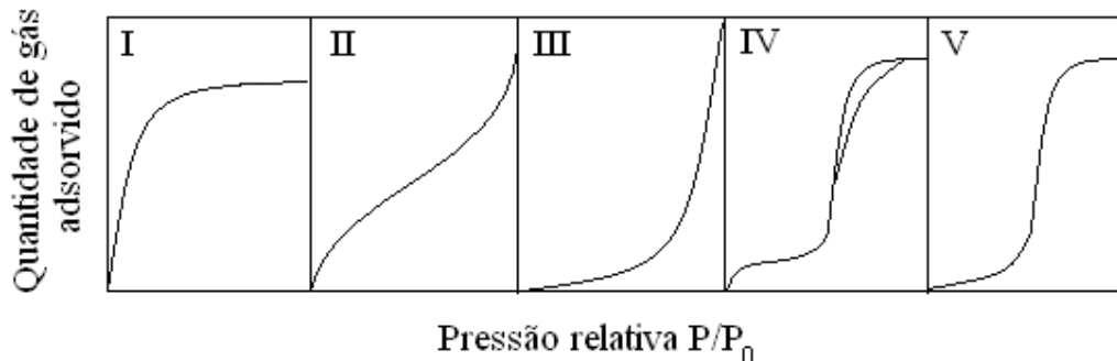
Figura III.8. Isotermas de adsorção segundo Brunauer, Emmet e Teller (BET)
