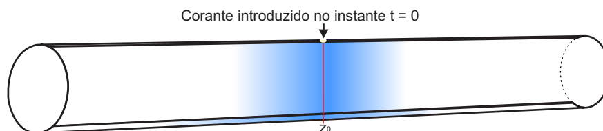
Figura 1.1: Um tubo estreito de comprimento infinito com água, onde foi introduzida uma quantidade de corante em uma posição z_0 .
