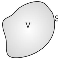
Figura 1.3: Volume V delimitado por uma superfície S .
