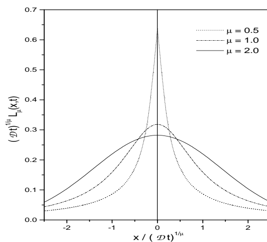
Figura 2.2: Comportamento de (Dt)^{1/\mu} L_\mu(x, t) versus x / (Dt)^{1/\mu} , para valores típicos de \mu . A derivada fracionária na variável espacial caracteriza um processo superdifusivo do tipo Lévy.
