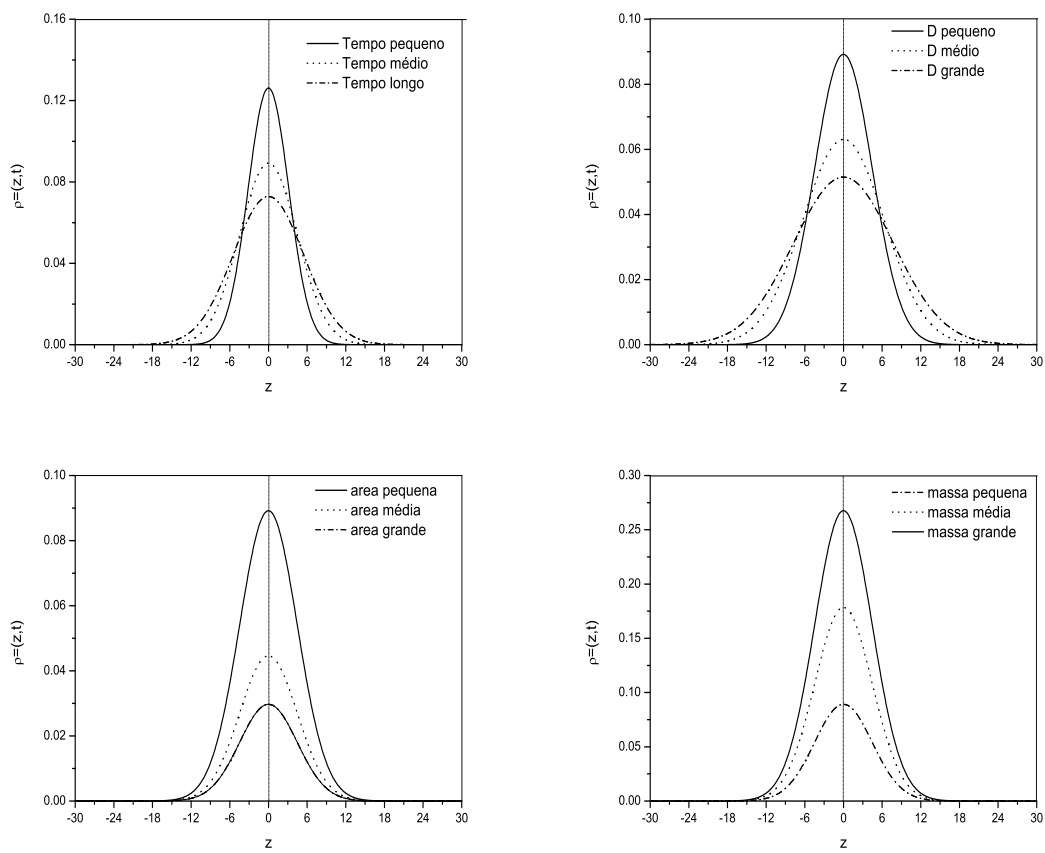
Figura 1.2: As curvas mostram a evolução temporal da distribuição \rho(z, t) no regime difusivo unidimensional. (a) a distribuição para diferentes intervalos de tempos; (b) para valor diferentes do coeficiente de difusão; (c) é a área que está variando; (d) para diferentes valores de massa.
