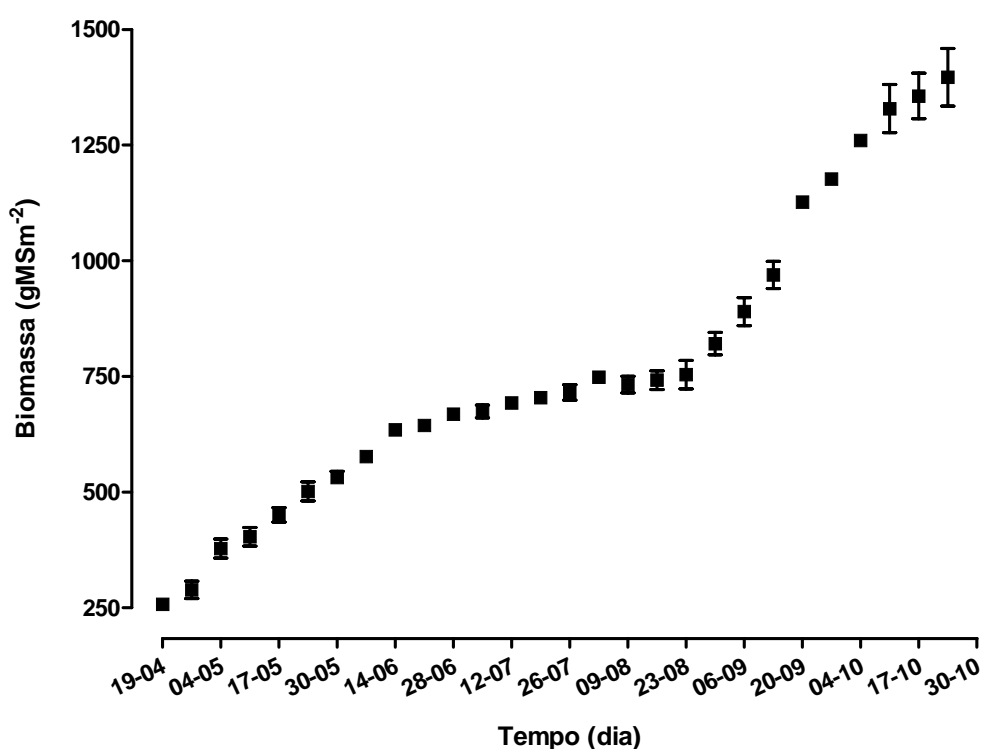
Figura 1. Curva de crescimento de Eichhornia crassipes ao longo do experimento.
