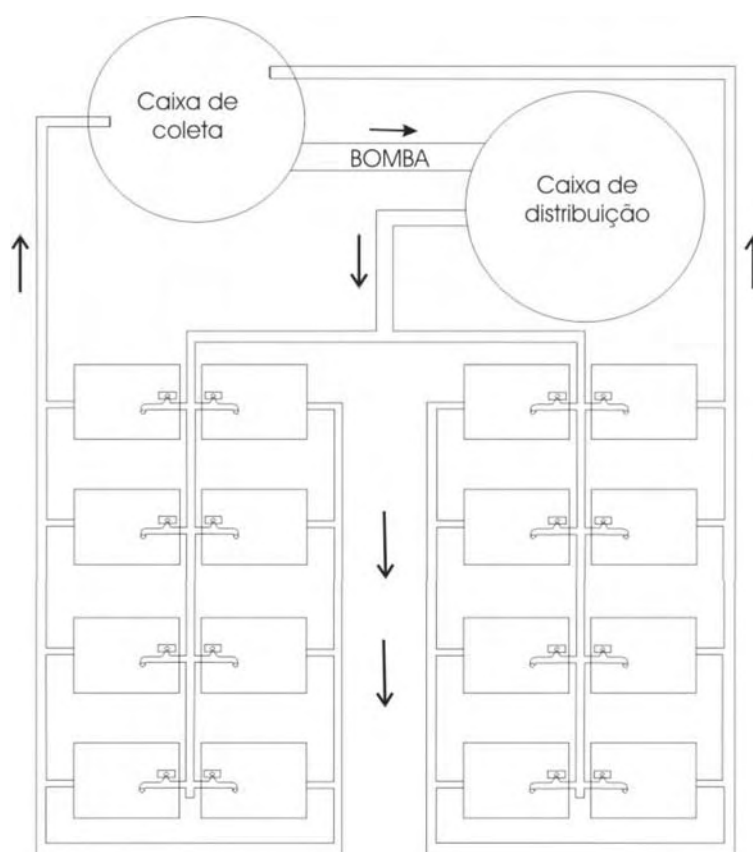
Figura 1. Esquema do sistema de recirculação de água.
