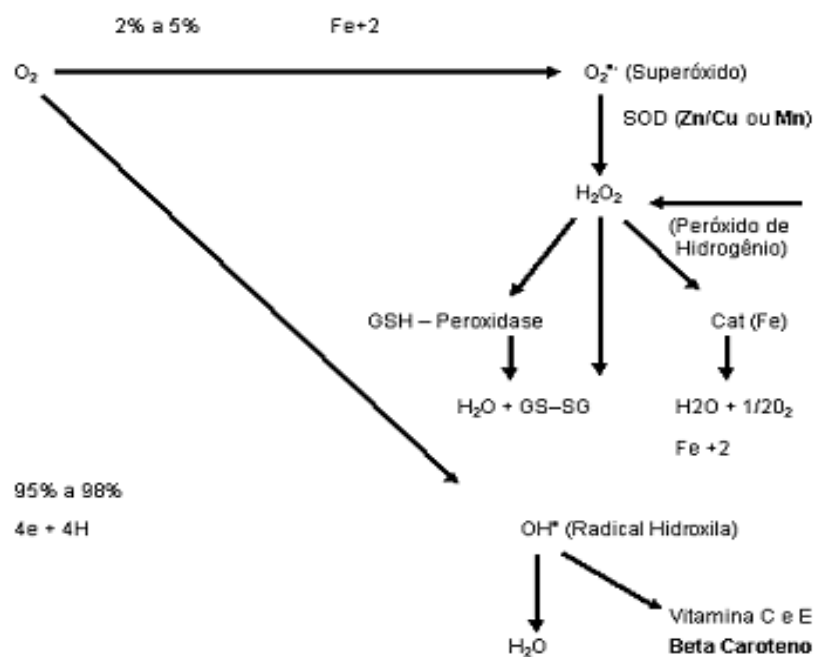
FIGURA 3. Cadeia de reações para formação das ERO.
