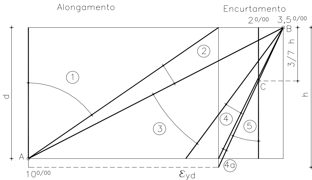
Figura 4.6 – Deformação para Estado Limite Último – ABNT NBR6118:2003
