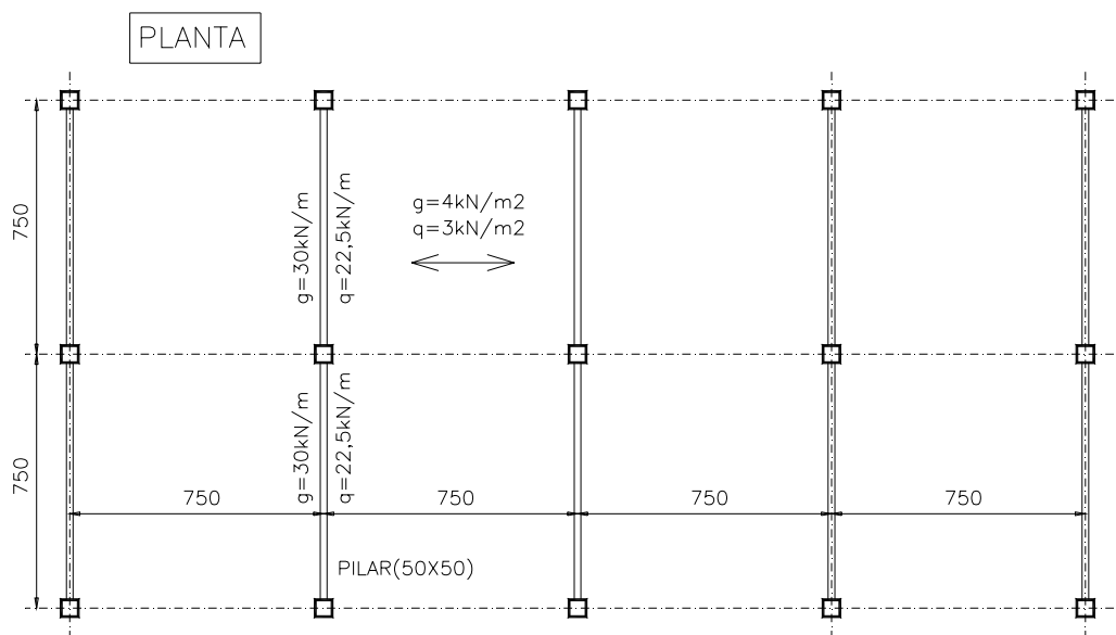
Figura 6.16 – Planta da estrutura analisada.
