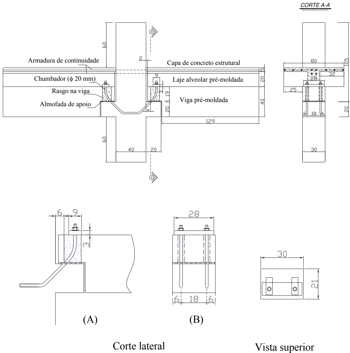
Figura 2.19 – Esquema da ligação ensaiada por BALDISSERA (2006).
