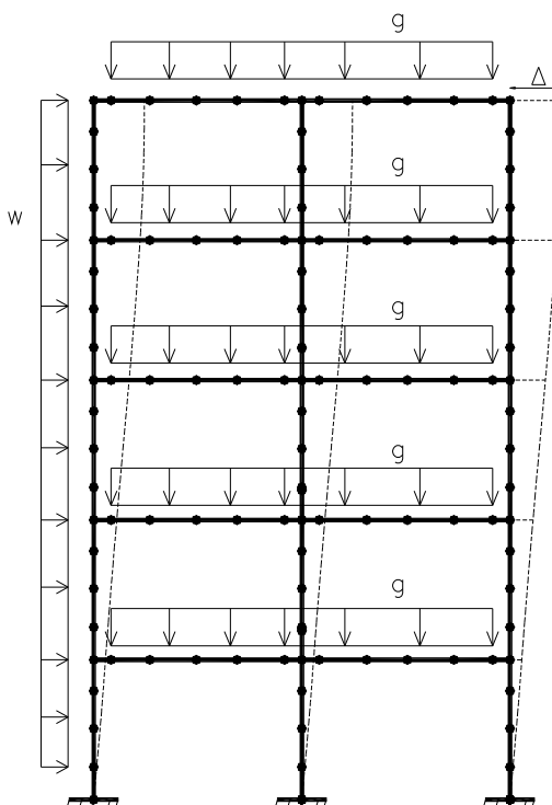
Figura 3.1 – Modelo de pórtico plano para análise não-linear geométrica.
