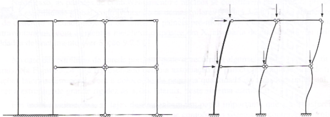
Figura 1.5 – Pórtico articulado ligado a uma parede de contraventamento.
