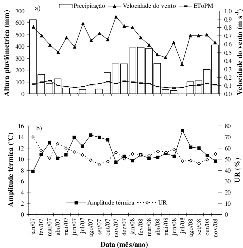
FIGURA 12. Média mensal, a) de precipitação, ETo de Penman-Monteith-FAO e velocidade do vento; b) Variação da amplitude térmica e umidade relativa do ar, durante os anos de 2007 e 2008, na bacia hidrográfica do ribeirão Lavrinha, região da Serra da Mantiqueira, MG.
