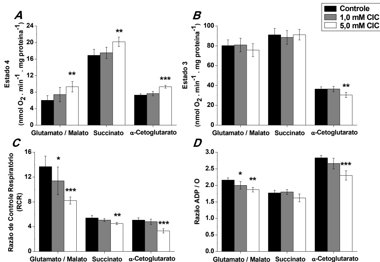
Figura 6. Efeito in vitro do ácido \alpha -cetoglutarato (CIC) sobre o consumo de oxigênio em mitocôndrias não estimuladas (estado 4) (A) e estimuladas por ADP (estado 3) (B) e sobre as razões de controle respiratório (RCR) (C) e ADP/O (D), utilizando glutamato/malato, succinato ou \alpha -cetoglutarato como substratos. Diferentes concentrações de CIC (1,0 - 5,0 mM) foram adicionadas ao meio de incubação contendo preparações mitocondriais (0,5 mg proteína . mL -1 ). Os valores representam média \pm desvio padrão (N = 4 -5) e os estados 3 e 4 da respiração mitocondrial são expressos como nmol O 2 . min -1 . mg proteína -1 . A diferença entre as médias foi calculada por análise de variância de uma via (ANOVA) seguida do teste de Duncan (* P <0,05; ** P <0,01; *** P <0,001, comparados ao controle).
