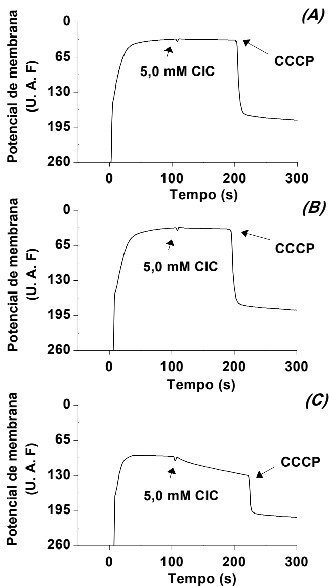
Figure 15. Efeito in vitro do ácido \alpha -cetoisocapróico (CIC) sobre o potencial de membrana mitocondrial utilizando glutamato/malato (A), succinato (B) ou \alpha -cetoglutarato (C) como substratos respiratórios. Após cem segundos o CIC foi adicionado na concentração de 5,0 mM ao meio de reação contendo a preparação mitocondrial (0,5 mg proteína . mL -1 ). CCCP (1 \mu M) foi adicionado no final das medições. Os traços são representativos de quatro experimentos independentes e expressos como unidades arbitrárias de fluorescência (U.A.F.).
