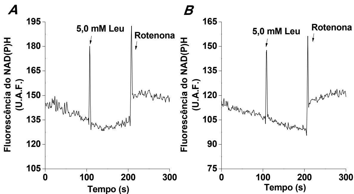
Figure 20. Efeito in vitro da leucina (Leu) sobre o conteúdo de NAD(P)H em preparações mitocondriais utilizando glutamato/malato (A) e \alpha -cetoglutarato (B) como substratos respiratórios. Após cem segundos a Leu foi adicionada na concentração de 5,0 mM ao meio de reação contendo a preparação mitocondrial ( 0,5 \text{ mg proteína} \cdot \text{mL}^{-1} ). Rotenona ( 4 \mu\text{M} ) foi adicionada no final das medições. Os traços são representativos de quarto experimentos independentes e foram expressos como unidades arbitrárias de fluorescência (U.A.F.).
