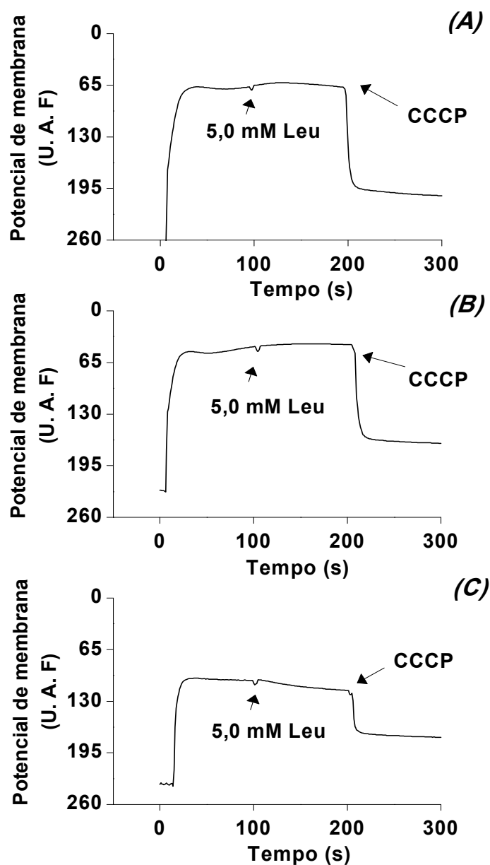
Figure 17. Efeito in vitro da leucina (Leu) sobre o potencial de membrana mitocondrial utilizando glutamato/malato (A), succinato (B) ou \alpha -cetoglutarato (C) como substratos respiratórios. Após cem segundos a Leu foi adicionada na concentração de 5,0 mM ao meio de reação contendo a preparação mitocondrial (0,5 mg proteína . mL -1 ). CCCP (1 \mu M) foi adicionado no final das medições. Os traços são representativos de quatro experimentos independentes e foram expressos como unidades arbitrárias de fluorescência (U.A.F.).
