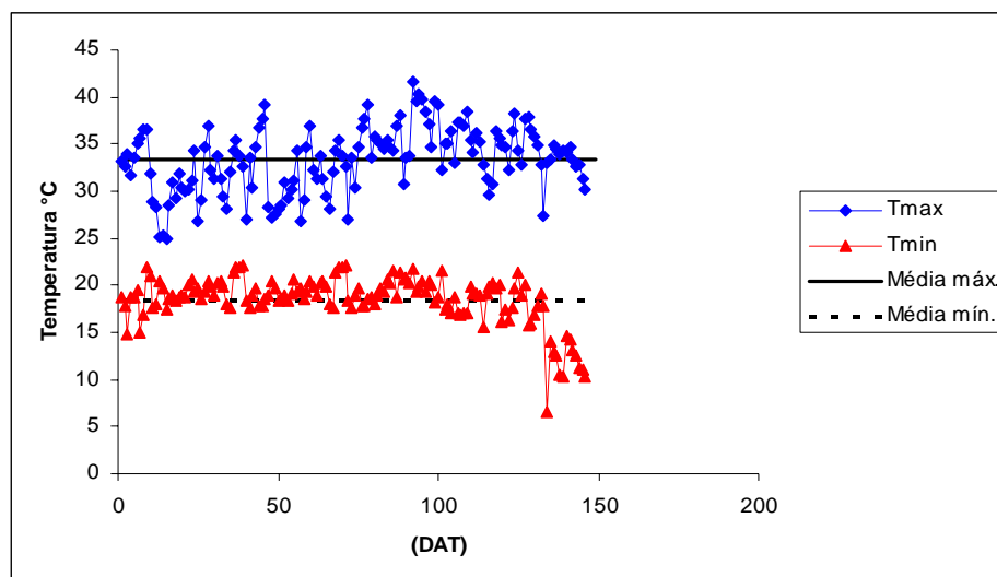
FIGURA 10 Temperatura (° C) máxima e mínima e suas respectivas médias máximas e mínimas, dentro da casa de vegetação.
