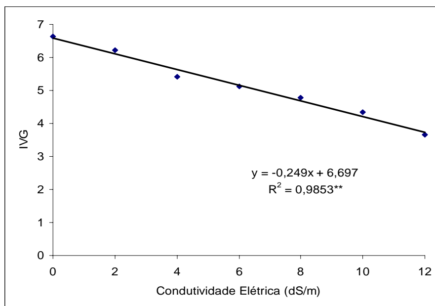
FIGURA 8 Índice de velocidade de germinação de plântulas de pinhão-mansão, em função de diferentes níveis de salinidade testados.
