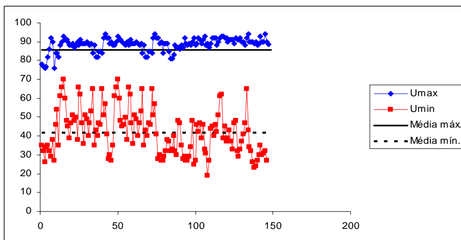
FIGURA 11 Umidade relativa do ar (%) máxima e mínima e suas respectivas médias máximas e mínimas, dentro da casa de vegetação.
