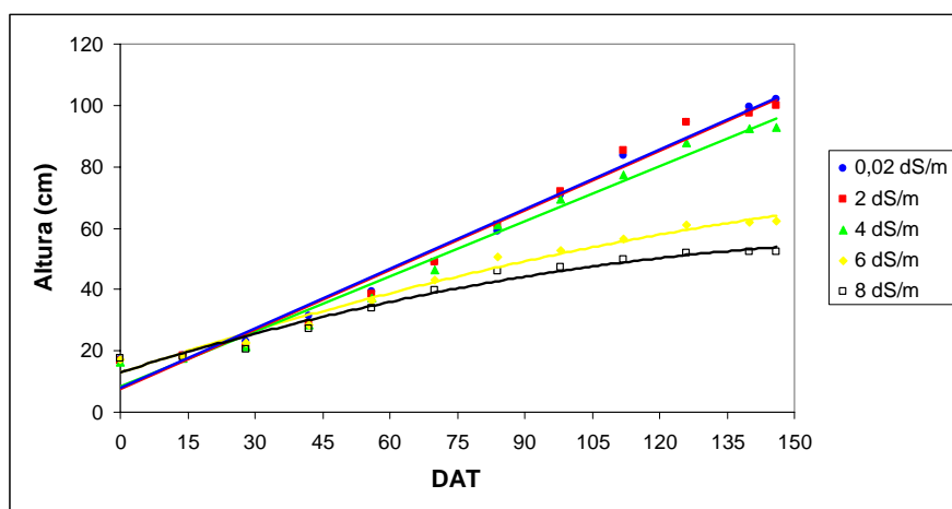
FIGURA 13 Dados de altura da planta (cm), em função de DAT e curvas de regressão para os diversos tratamentos.
