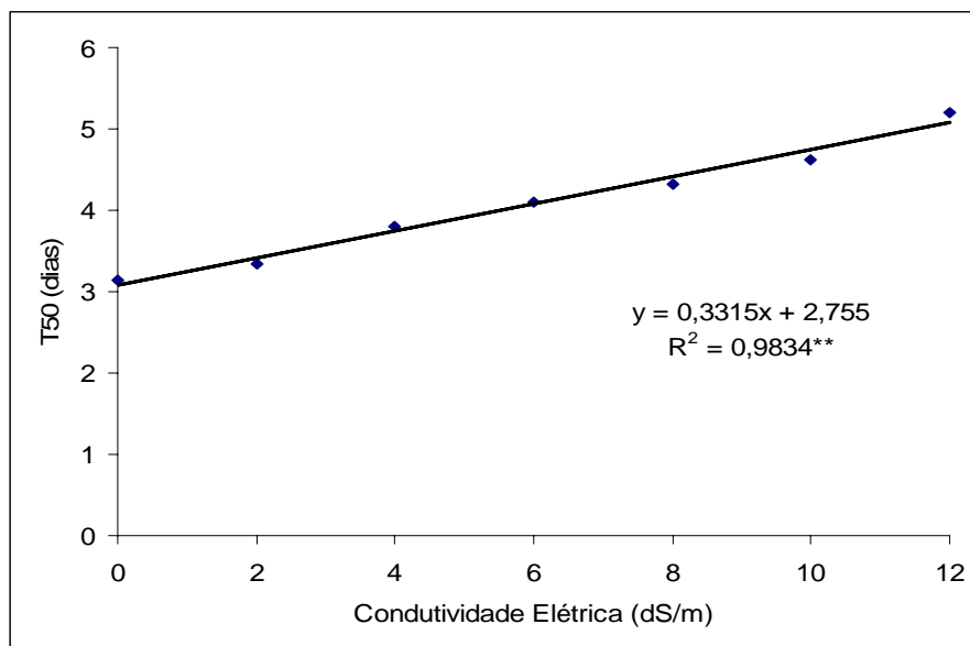
FIGURA 9 Tempo necessário para germinação de 50% de sementes de pinhão-mansão, em função dos diferentes níveis de salinidade estudados.
