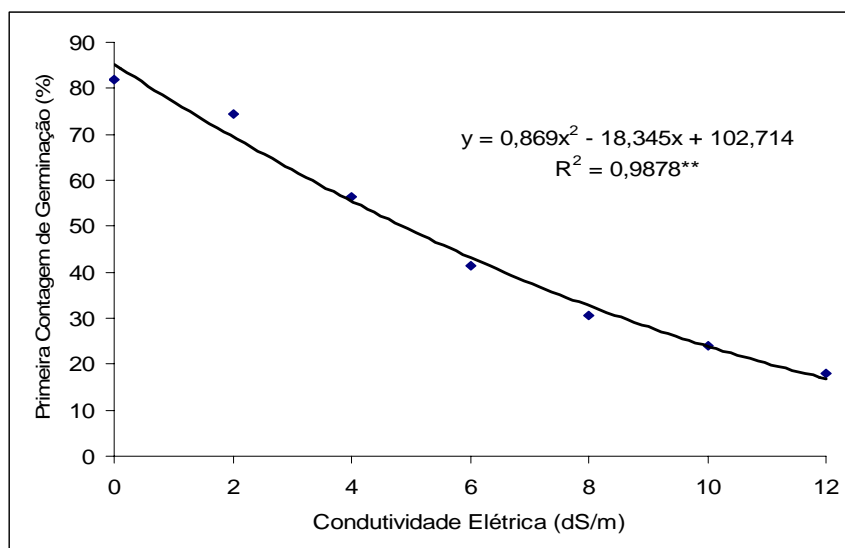
FIGURA 7 Percentagem de germinação de plântulas de pinhão-mansão na primeira contagem, em função de diferentes níveis de salinidade testados.
