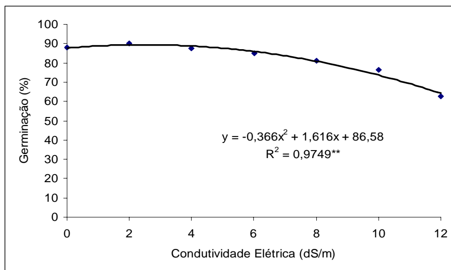
FIGURA 6 Percentagem de germinação de plântulas de pinhão-mansó em função de diferentes níveis de salinidade testados.
