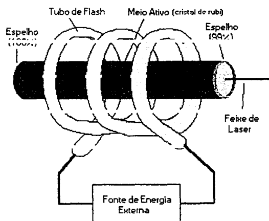
Figura1 esquematiza o LASER de rubi desenvolvido em 1960
