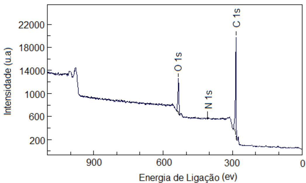
FIGURA 16 – ESPECTRO DE XPS PARA O CARVÃO ORGÂNICO MODIFICADO COM HNO 3 .
