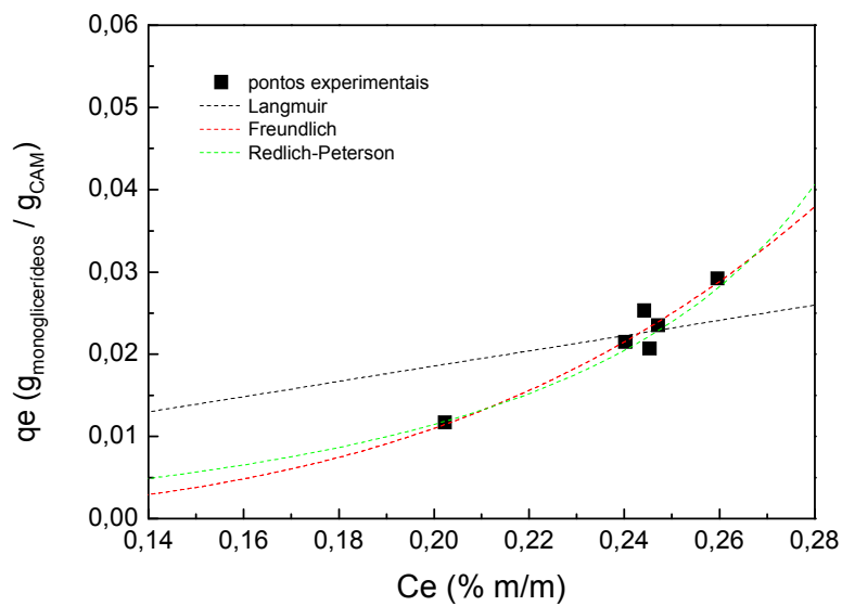
FIGURA 28 – ISOTERMA DE ADSORÇÃO DOS MONOGLICERÍDEOS A 20 °C.
