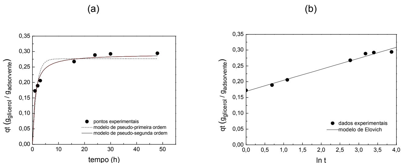
FIGURA 21 – MODELAGEM DOS DADOS EXPERIMENTAIS DA CINÉTICA DE ADSORÇÃO DO GLICEROL UTILIZANDO CAM. (a) MODELO DE PSEUDO-PRIMEIRA E PSEUDO-SEGUNDA ORDEM. (b) MODELO DE ELOVICH.
