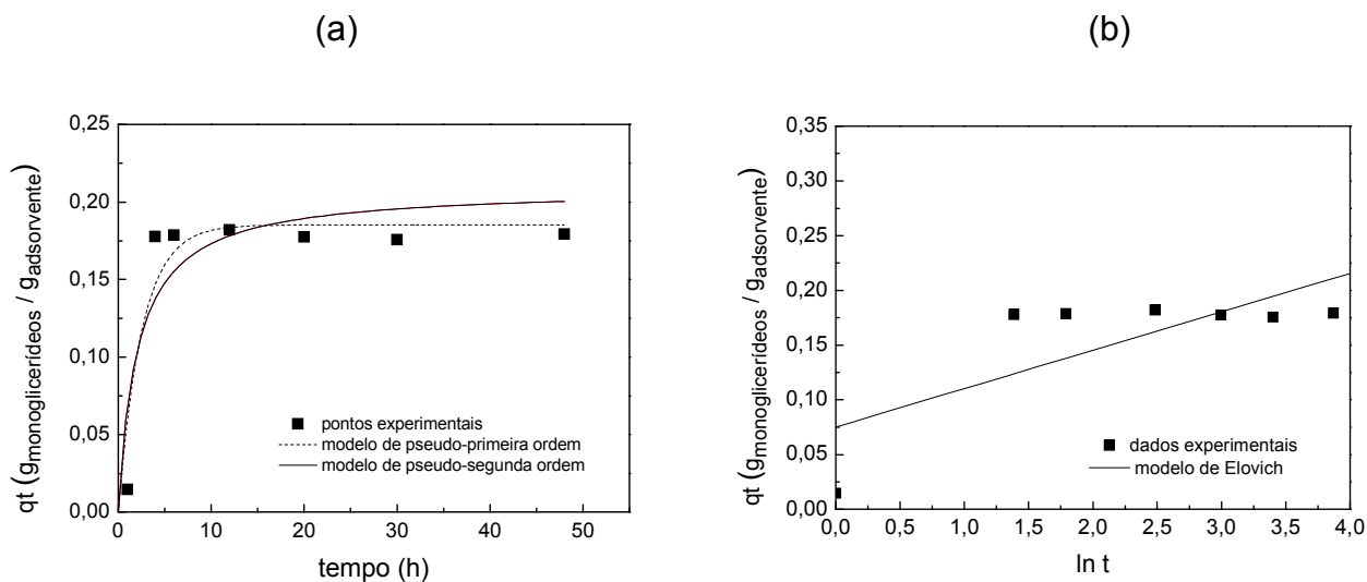
FIGURA 22 – MODELAGEM DOS DADOS EXPERIMENTAIS DA CINÉTICA DE ADSORÇÃO DO MONOGLICERÍDEO UTILIZANDO CAM. (a) MODELO DE PSEUDO-PRIMEIRA E PSEUDO-SEGUNDA ORDEM. (b) MODELO DE ELOVICH.
