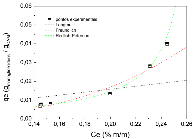
FIGURA 29 – ISOTERMA DE ADSORÇÃO DOS MONOGLICERÍDEOS A 40 °C.
