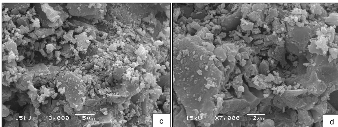
FIGURA 14 – MICROSCOPIA ELETRÔNICA DO CAM. (c) AUMENTO DE 3000X, (d) AUMENTO DE 7000X.
