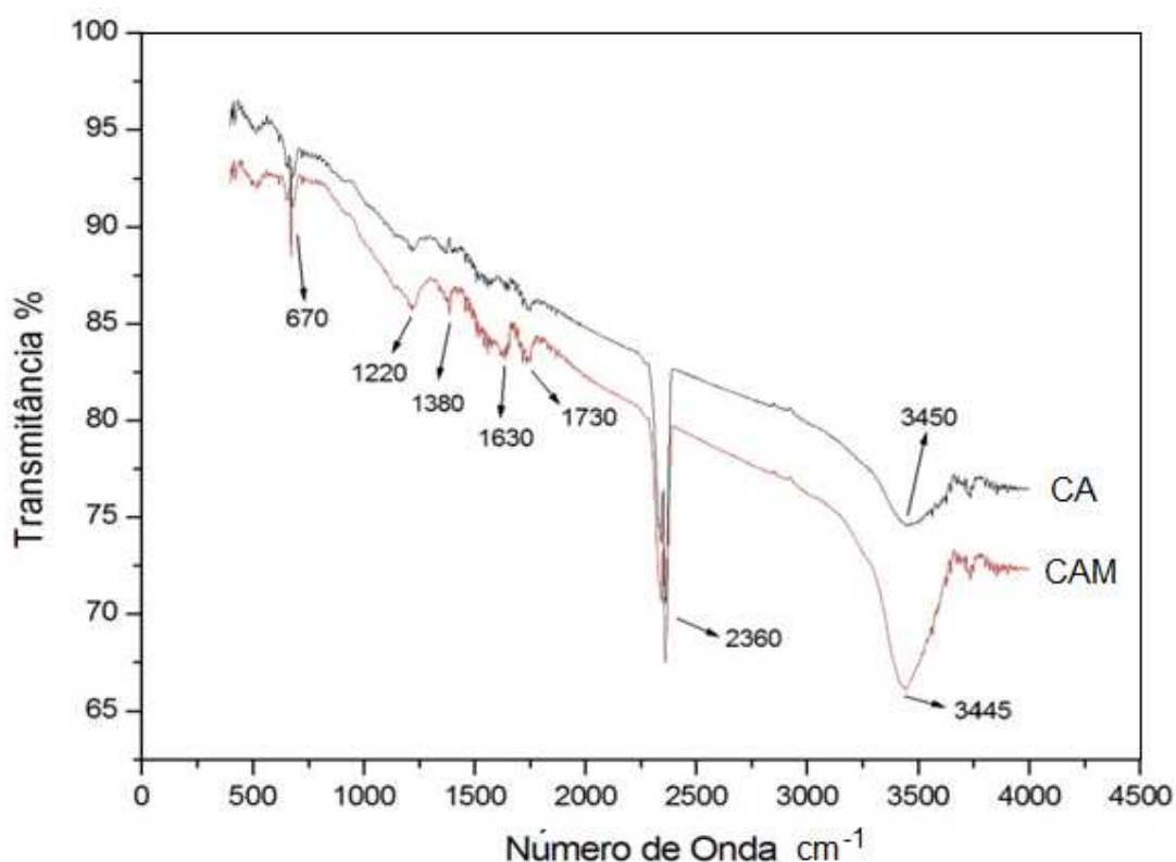
FIGURA 17 – ESPECTRO FTIR DO CA E CAM.
