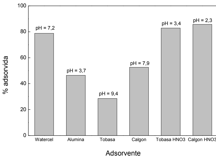
FIGURA 12 – AVALIAÇÃO DA REMOÇÃO DO GLICEROL REMANESCENTE NO BIODIESEL UTILIZANDO DIFERENTES ADSORVENTES. T = 50 °C; t = 24 h.
