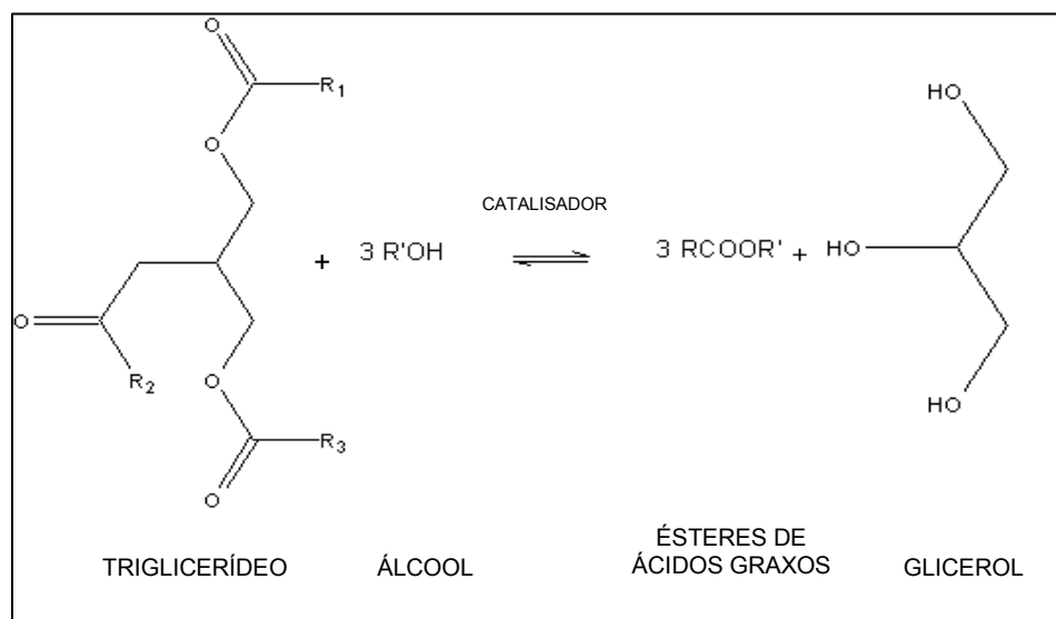
FIGURA 2 – TRANSESTERIFICAÇÃO DE TRIGLICERÍDEOS COM ÁLCOOL, PRODUZINDO ÉSTERES DE ÁCIDOS GRAXOS E GLICEROL.
