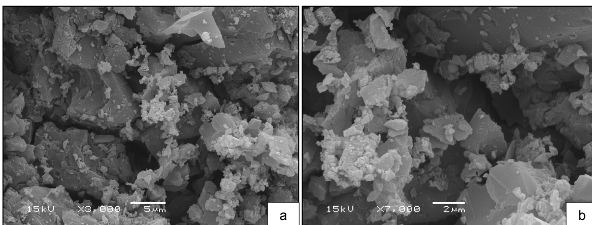
FIGURA 13 – MICROSCOPIA ELETRÔNICA DO CA. (a) AUMENTO DE 3000X, (b) AUMENTO DE 7000X.
