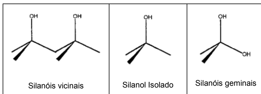
FIGURA 3 – TIPOS DE GRUPOS SILANÓIS NORMALMENTE ENCONTRADOS NA SUPERFÍCIE DA SÓLICA GEL. O ÁTOMO CENTRAL É O SILÍCIO, LIGADO AOS GRUPOS SILANÓIS.
