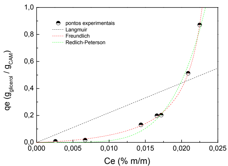
FIGURA 26 – ISOTERMA DE ADSORÇÃO DO GLICEROL A 30 °C.
