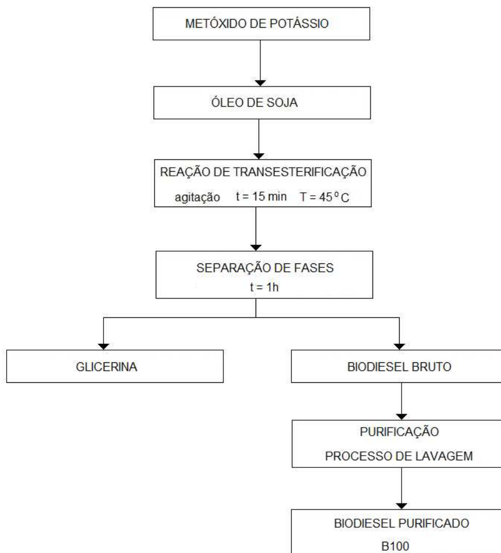
FIGURA 7 – DIAGRAMA ESQUEMÁTICO DA PRODUÇÃO DO BODIESEL.
