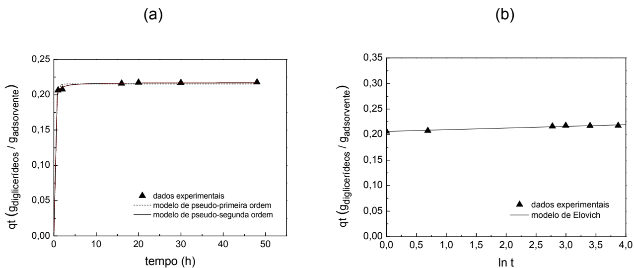
FIGURA 23 – MODELAGEM DOS DADOS EXPERIMENTAIS DA CINÉTICA DE ADSORÇÃO DOS DIGLICERÍDEOS UTILIZANDO CAM. (a) MODELO DE PSEUDO-PRIMEIRA E PSEUDO-SEGUNDA ORDEM E (b) MODELO DE ELOVICH.
