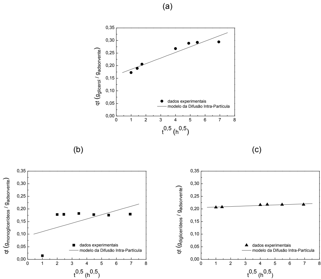
FIGURA 24 – MODELAGEM DA DIFUSÃO INTRA-PARTÍCULA. (a) GLICEROL, (b) MONOGLICÉRIDES E (c) DIGLICÉRIDES UTILIZANDO CAM.
