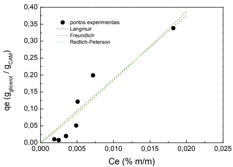
FIGURA 25 – ISOTERMA DE ADSORÇÃO DO GLICEROL A 20 °C.
