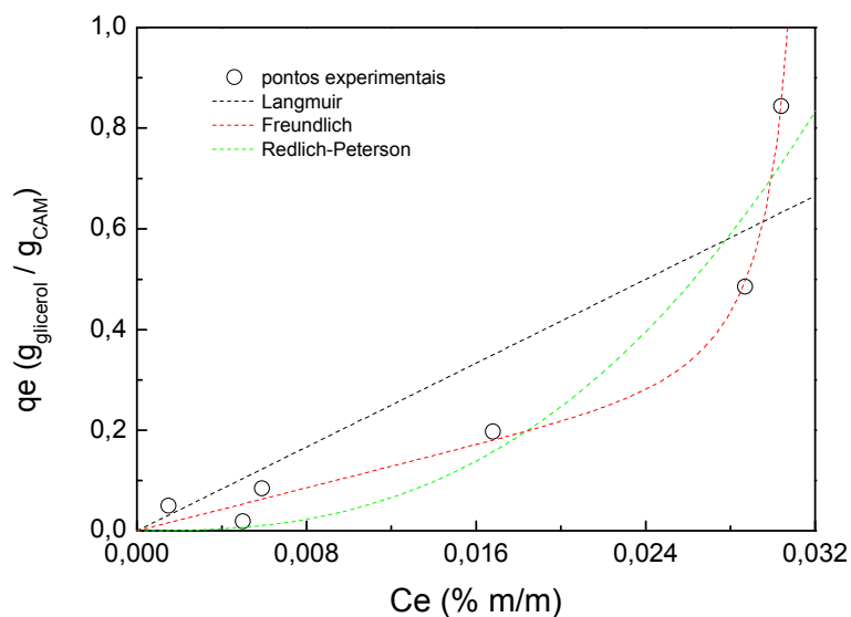
FIGURA 27 – ISOTERMA DE ADSORÇÃO DO GLICEROL A 40 °C.
