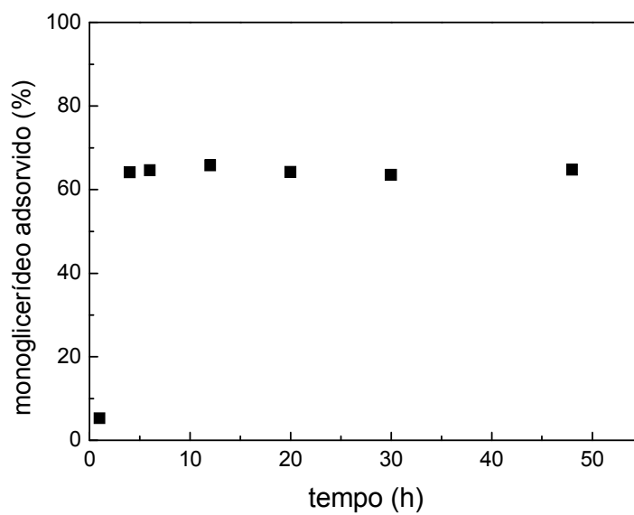
FIGURA 19 – CINÉTICA DE ADSORÇÃO DO MONOGLICERÍDEO PRESENTE NO BODIESEL BRUTO UTILIZANDO CAM. C_0 = 0,3860 \text{ \% (M/M)} ; V = 150 \text{ RPM} ; T = 30 \text{ }^\circ\text{C} .
