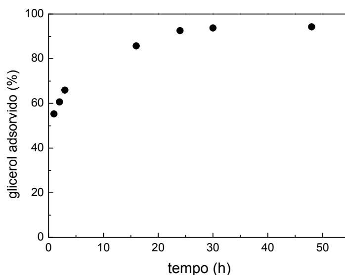
FIGURA 18 – CINÉTICA DE ADSORÇÃO DO GLICEROL PRESENTE NO BIODIESEL BRUTO UTILIZANDO CAM. C_0 = 0,4354 \text{ \% (m/m)} ; V = 150\text{RPM} ; T = 30 \text{ }^\circ\text{C} .
