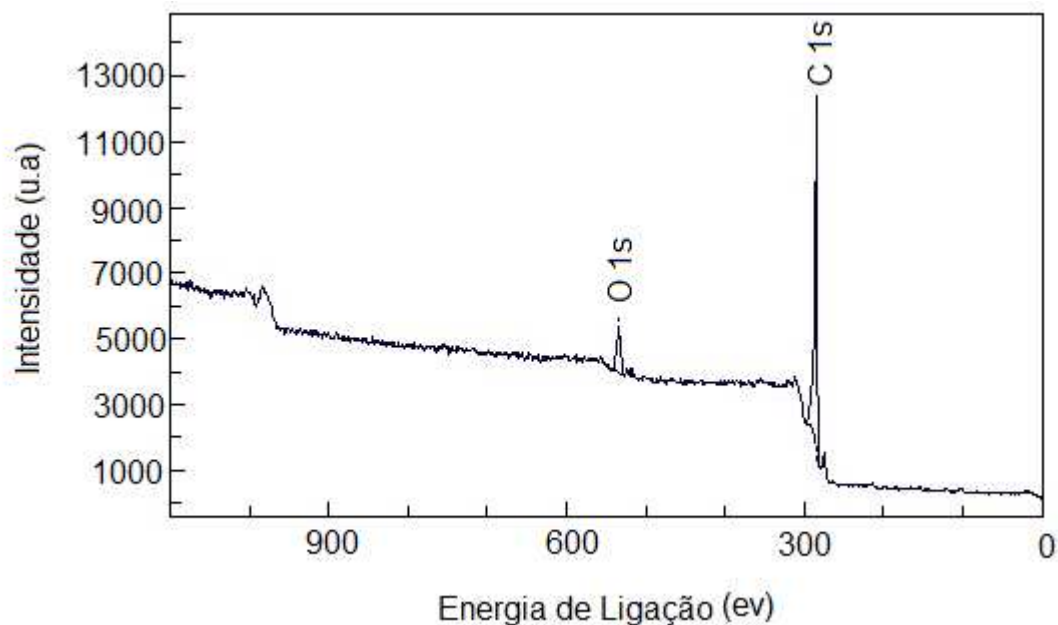
FIGURA 15 – ESPECTRO DE XPS PARA O CARVÃO ORGÂNICO ORIGINAL.
