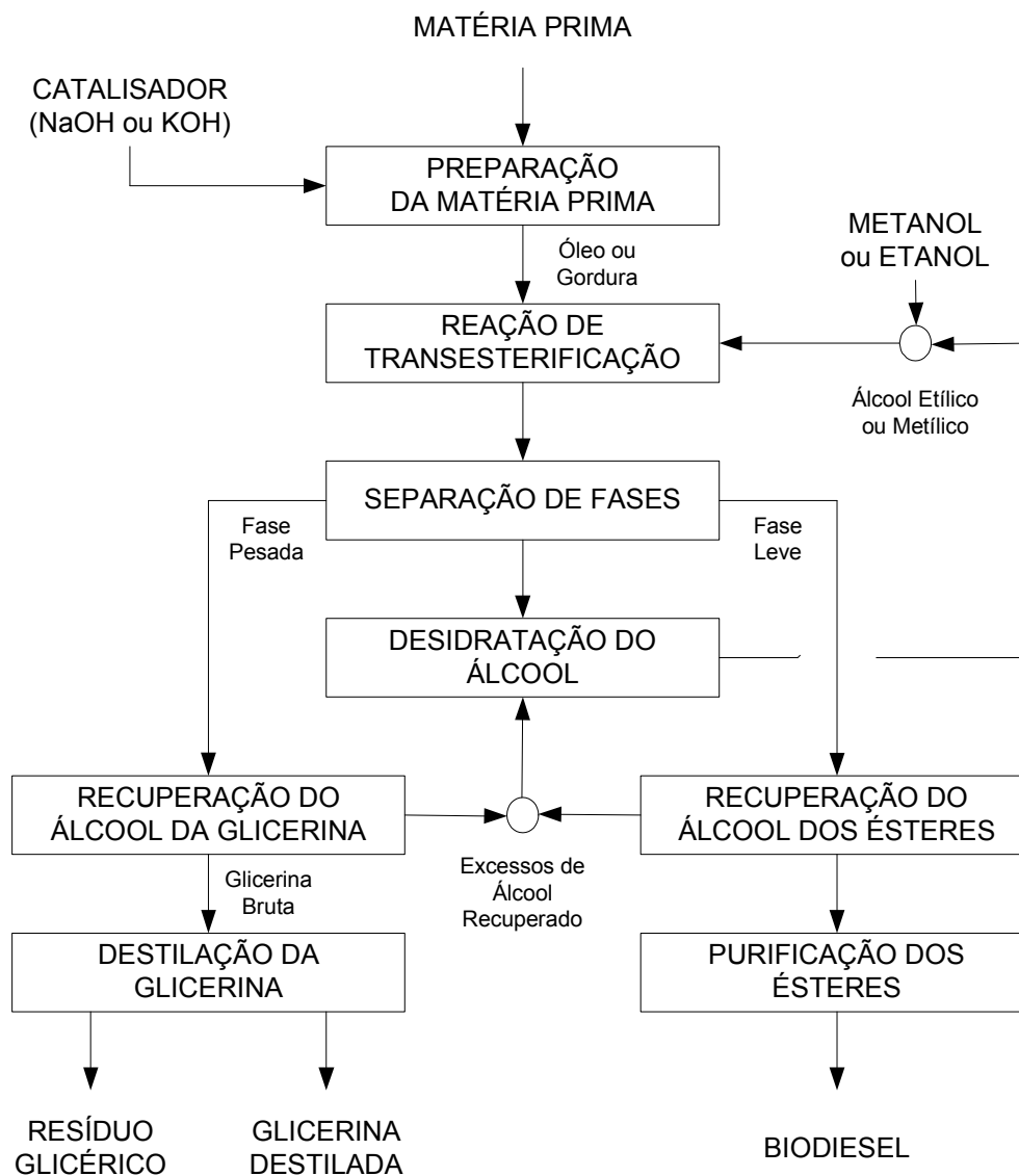
FIGURA 1 – FLUXOGRAMA DO PROCESSO DE PRODUÇÃO DO BODIESEL. FONTE: PARENTE, 2003.
