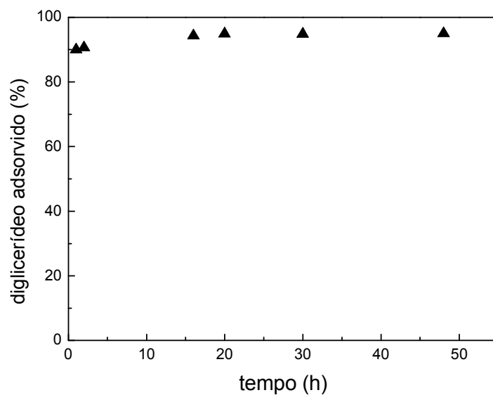
FIGURA 20 – CINÉTICA DE ADSORÇÃO DO DIGLICERÍDEO PRESENTE NO BODIESEL BRUTO UTILIZANDO CAM. C_0 = 0,0320 \text{ \% (M/M)} ; V = 150 \text{ RPM} ; T = 30 \text{ }^\circ\text{C} .
