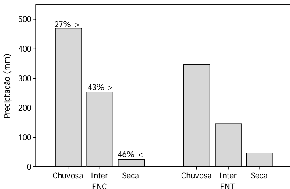
Figura 4 – Comparação entre os volumes médios de precipitação na Floresta Nacional de Caxiuanã (F.N.C.) e Floresta Nacional do Tapajós (F.N.T.) durante o período de amostragem
