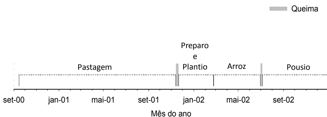
Figura 11 – Caracterização da mudança no uso do solo na área agrícola no período entre setembro/2000 e dezembro/2002
