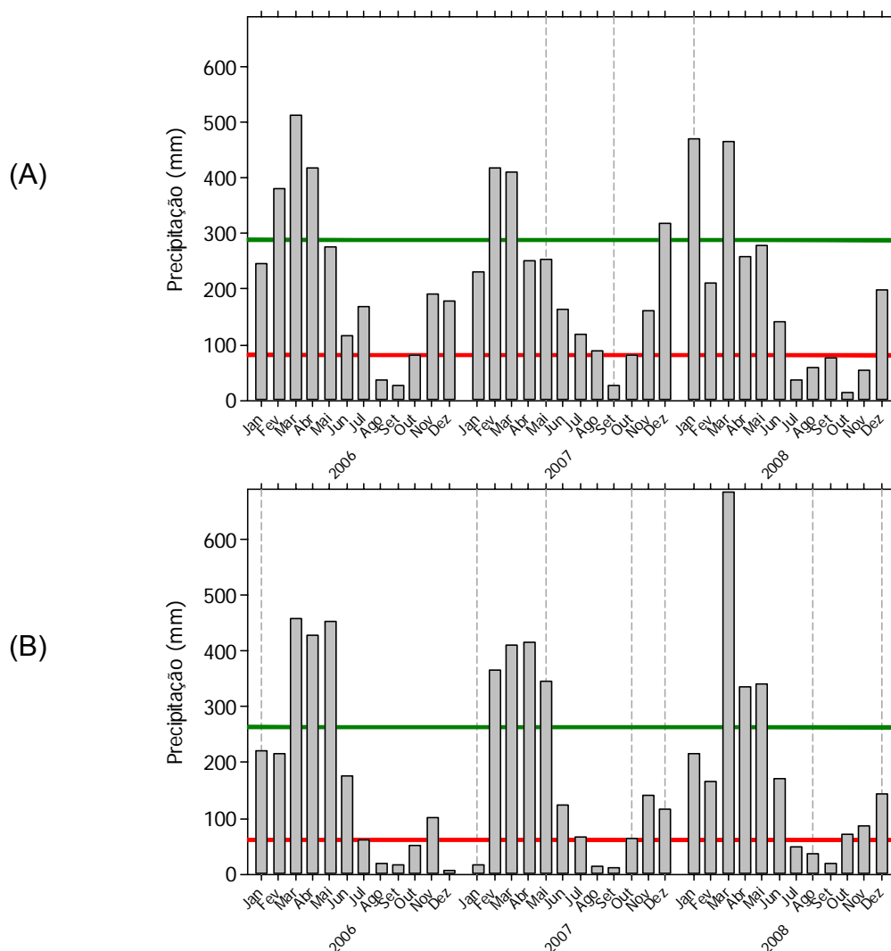
Figura 3 - Média mensal de precipitação nos municípios de Breves-PA (A) e em Belterra-PA (B) 19 . As linhas verticais tracejadas indicam o período de cada coleta. As linhas horizontais vermelhas indicam o limite entre as estações seca e intermediária e as linhas verdes indicam o limite entre a estação intermediária e chuvosa 20
