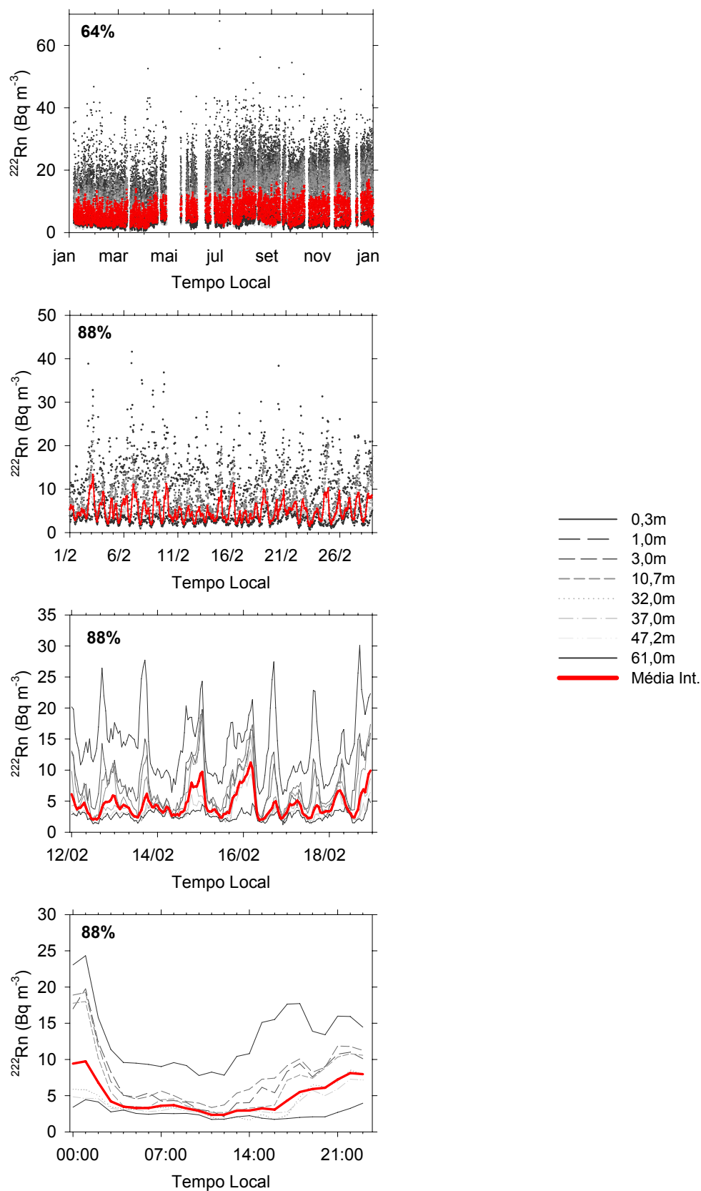
Figura 15 – Exemplos do inventário da atividade de ^{222}\text{Rn} medida ao longo do tempo (ano de 2001) no perfil vertical da floresta em diferentes alturas. A cobertura dos dados para cada período está expressa em percentagem no canto superior esquerdo de cada gráfico. O gráfico inferior refere-se ao dia 15 de fevereiro de 2001
