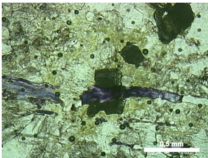
Figura 18 - Veio de fluorita cortando grão de zircão a luz natural.
