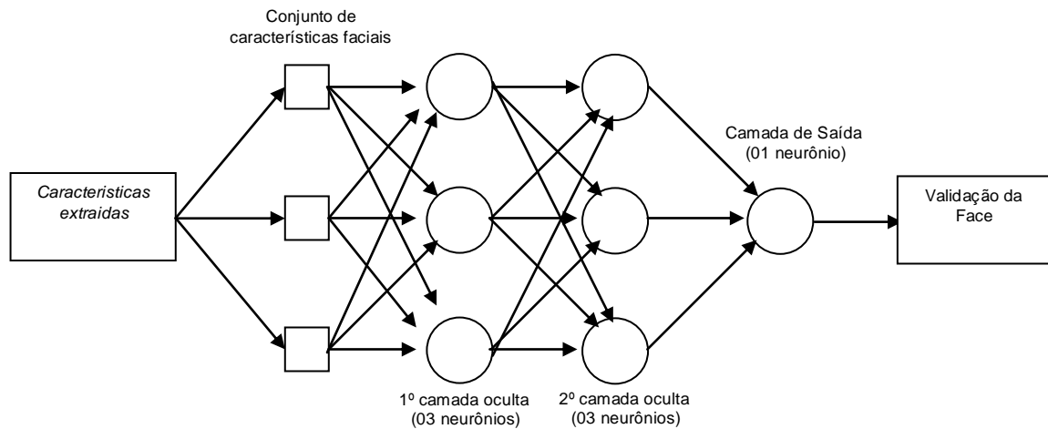
Figura 41 – Topologia da Rede Neural proposta para a detecção de face
