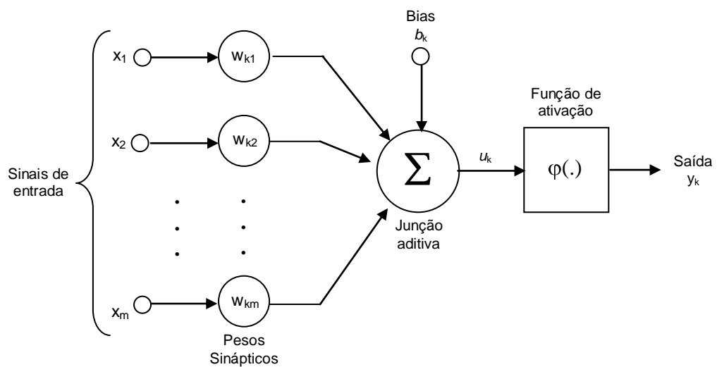
Figura 19 - Modelo não-linear de um neurônio (HAYKIN, 2001)
