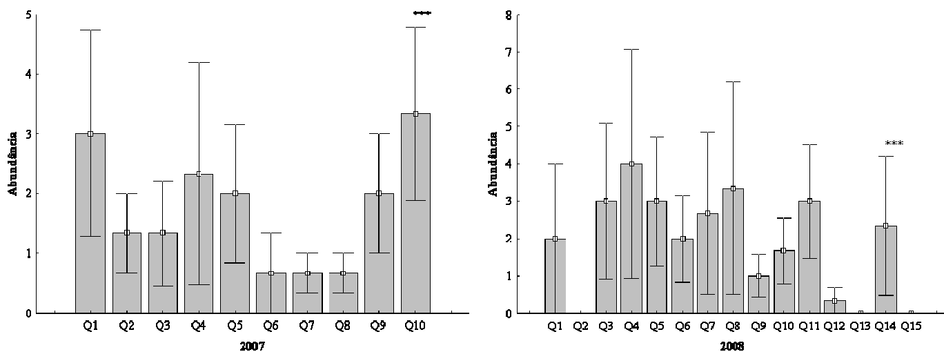
Figura 11 – Abundância de ninhos de formigas do gênero Ectatomma presentes nos quadrantes amostrados em área de cerrado nos anos de 2007 e 2008. ***indica diferença significativa ( p < 0.0001 ) entre as áreas (ANOVA para medidas repetidas).
