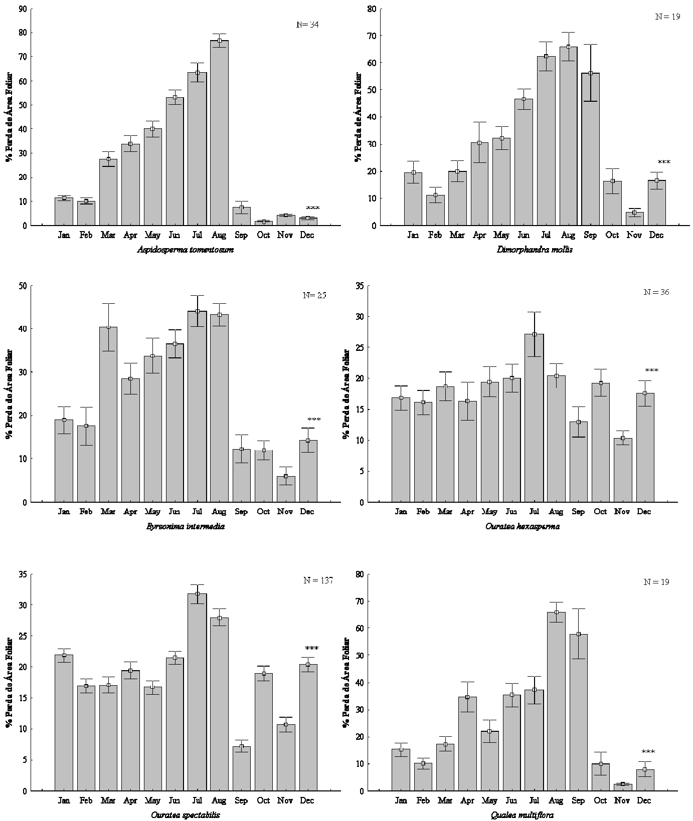
Figura 7 – Perda de área foliar ( X \pm 1 erro padrão) em plantas arbóreas com alta abundância ( N \geq 19 ) e presentes em mais de 50% dos quadrantes amostrados em área de cerrado. *** indica diferença significativa ( p < 0,0001 ) entre os meses (ANOVA para medidas repetidas).
