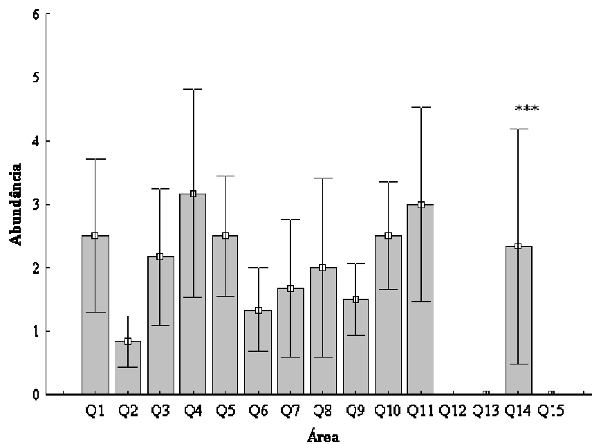
Figura 10 – Abundância de ninhos de formigas do gênero Ectatomma presentes nos quadrantes amostrados em área de cerrado. ***indica diferença significativa ( p < 0.0001 ) entre as áreas (ANOVA para medidas repetidas).
