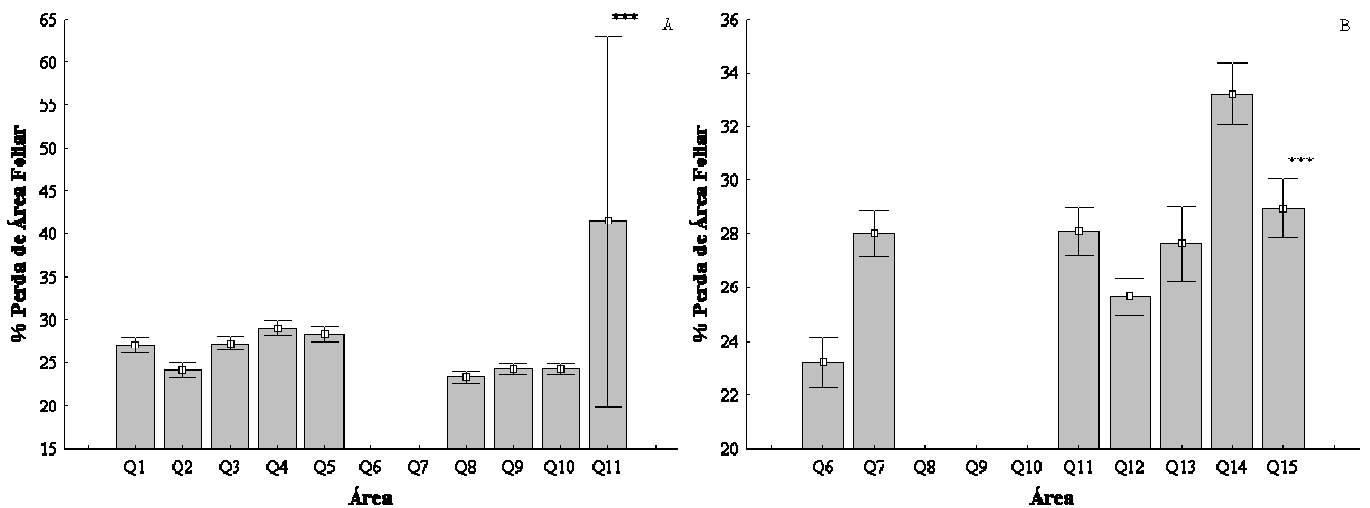
Figura 13 – Perda de área foliar ( X \pm 1 erro padrão) em áreas com (A) e sem (B) a presença de ninhos de formigas do gênero Ectatomma em área de cerrado. ***indica diferença significativa ( p < 0.0001 ) (ANOVA para medidas repetidas).
