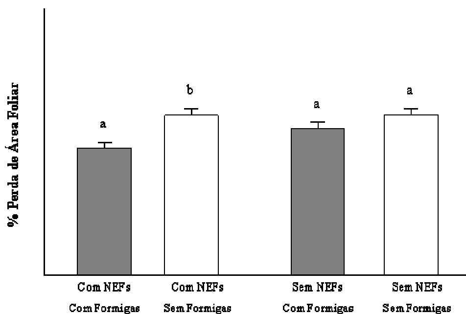
Figura 15 – Perda de área foliar ( X \pm 1 erro padrão) em plantas com e sem a presença de nectários extraflorais (NEFs) e com e sem formigas do gênero Ectatomma amostradas em área de cerrado nos anos de 2007 e 2008 respectivamente. Letras diferentes indicam diferença significativa ( p < 0.0001 ) entre as áreas (Mann-Whitney U teste).
