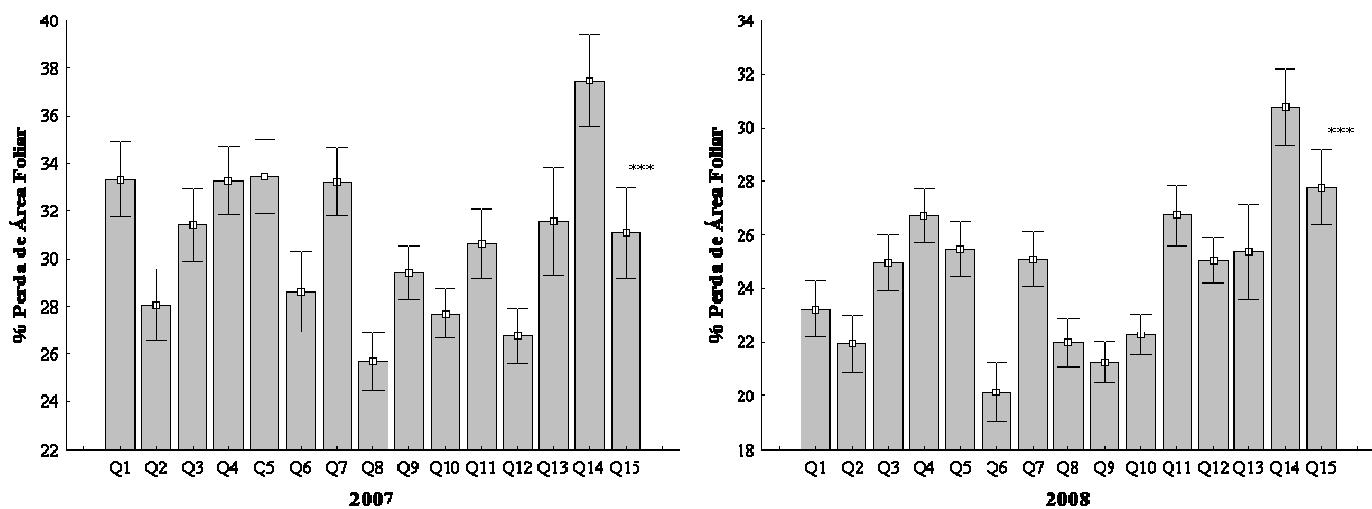
Figura 9 – Perda de área foliar ( X \pm 1 erro padrão) de acordo com a área (15 quadrantes de 10 x 10 m) de uma comunidade de plantas de cerrado sensu stricto em 2007 e 2008. *** indica diferença significativa ( p < 0.0001 ) (ANOVA para medidas repetidas).
