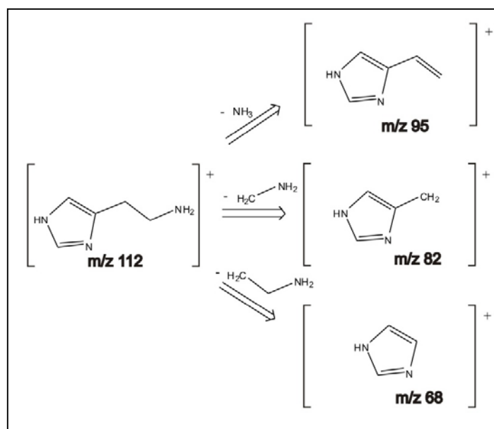
Esquema 1- Representação da fragmentação da Histamina.
