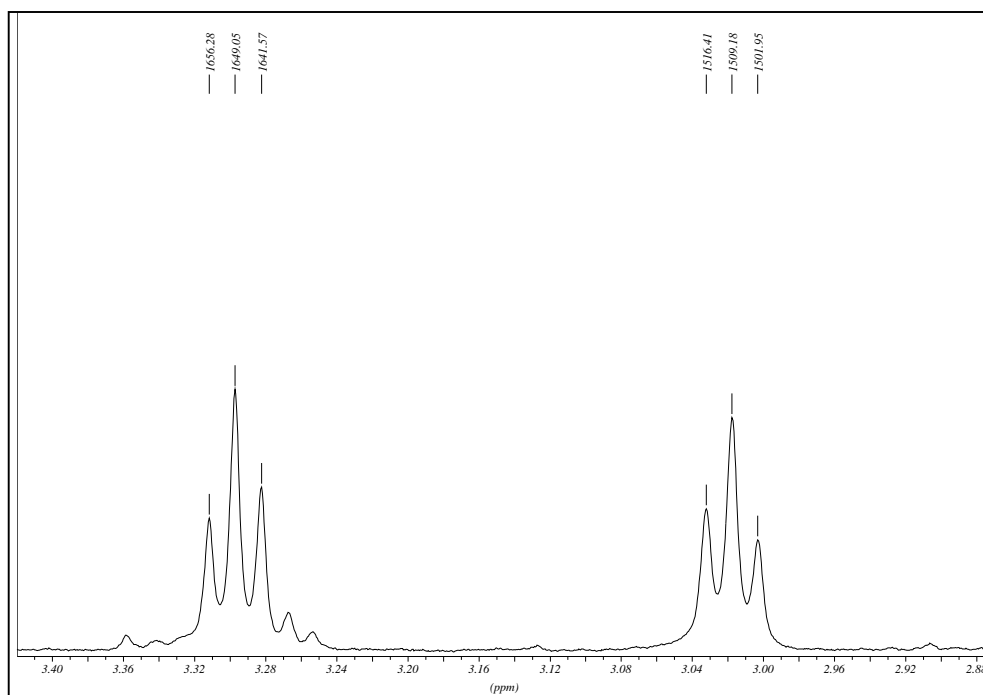
Figura 43- Ampliação do espectro de RMN- ^1\text{H} mostrando dois tripletos em 3,02 e 3,3 ppm
