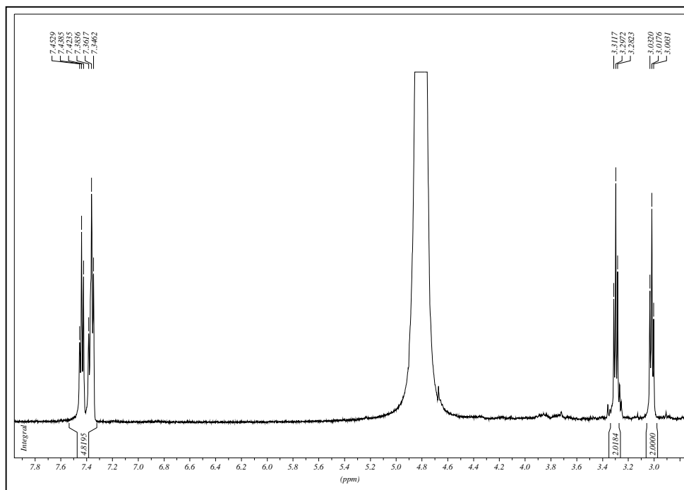
Figura 42- Espectro de RMN- ^1\text{H} em \text{D}_2\text{O} da fração 5 do veneno da vespa social Poybia paulista
