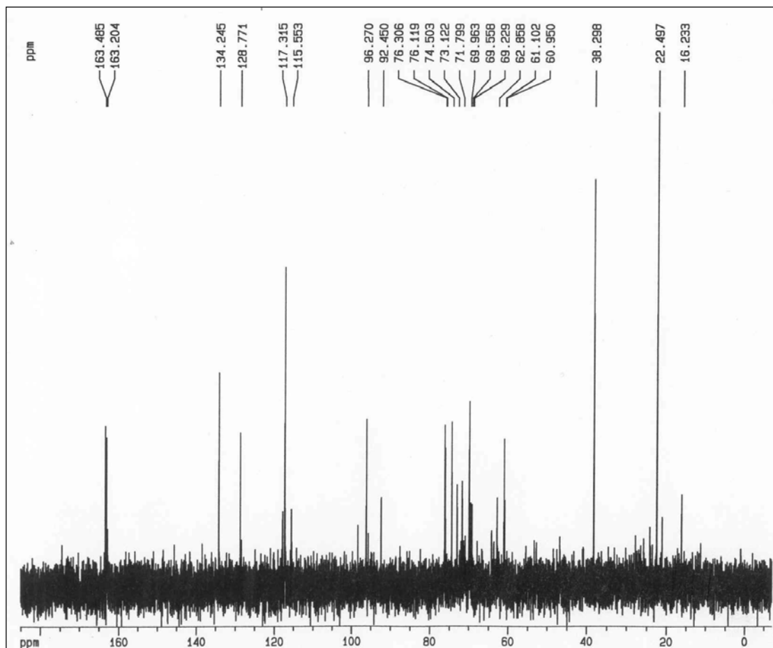
Figura 21- Espectro de RMN de ^{13}\text{C} a 125 MHz em \text{D}_2\text{O} do composto presente na fração 1A do veneno da vespa social Polybia paulista .
