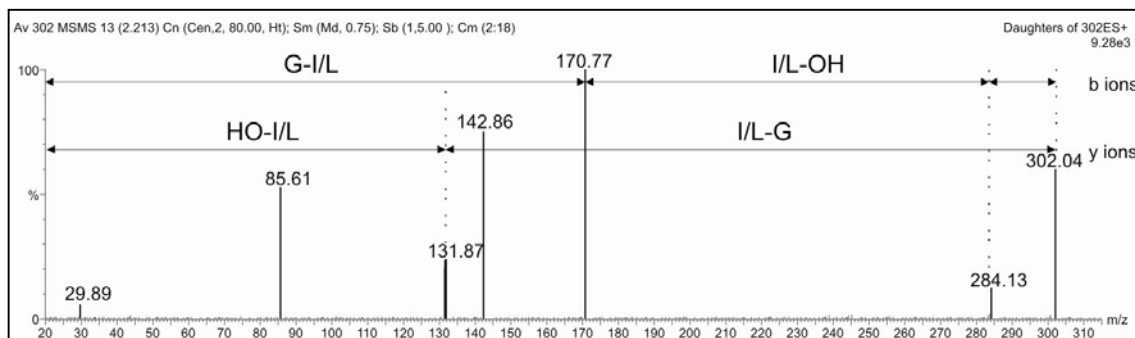
Figura 16- Espectro de ESI-MS/MS no modo positivo, do composto isolado da fração 7 do veneno da vespa Agelaia vicina , mostrando um padrão de fragmentação de um peptídeo com uma seqüência de resíduos aminoácidos G-I/L-I/L-OH.
