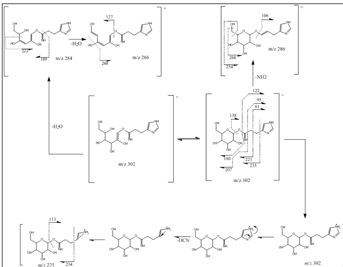
Esquema 3- Esquema de fragmentação para o Polybiosídeo mostrada na figura 23.
