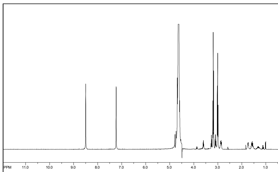
Figura A2- Espectro de 1 H-RMN em D 2 O da fração 1, isolada da vespa A. vicina , com sua possível interpretação.
