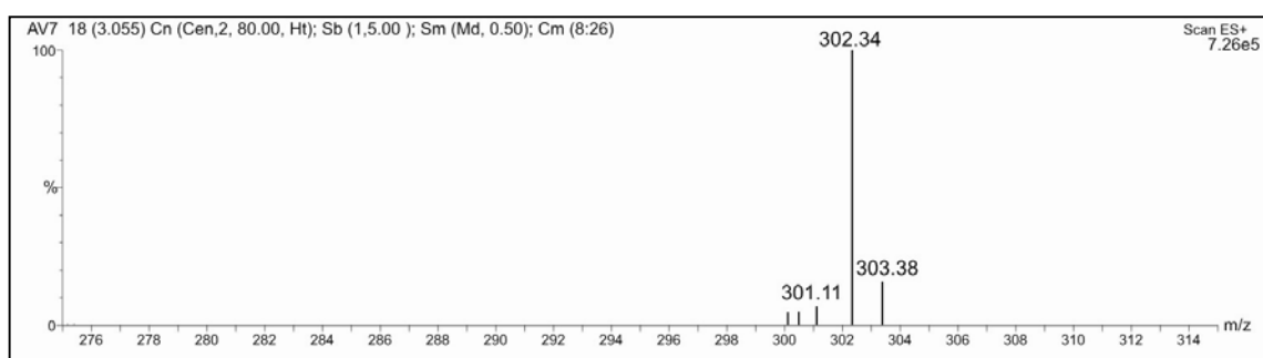
Figura 15- Espectro de ESI-MS/MS no modo positivo, do composto isolado da fração 7 do veneno da vespa Agelaia vicina .
