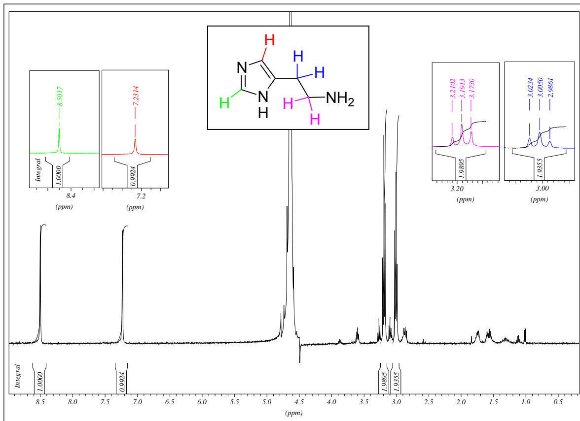
Figura 7: Espectro de 1 H-RMN em D 2 O da fração 1-4, isolada da vespa Agelaia pallipes pallipes , com sua possível interpretação.
