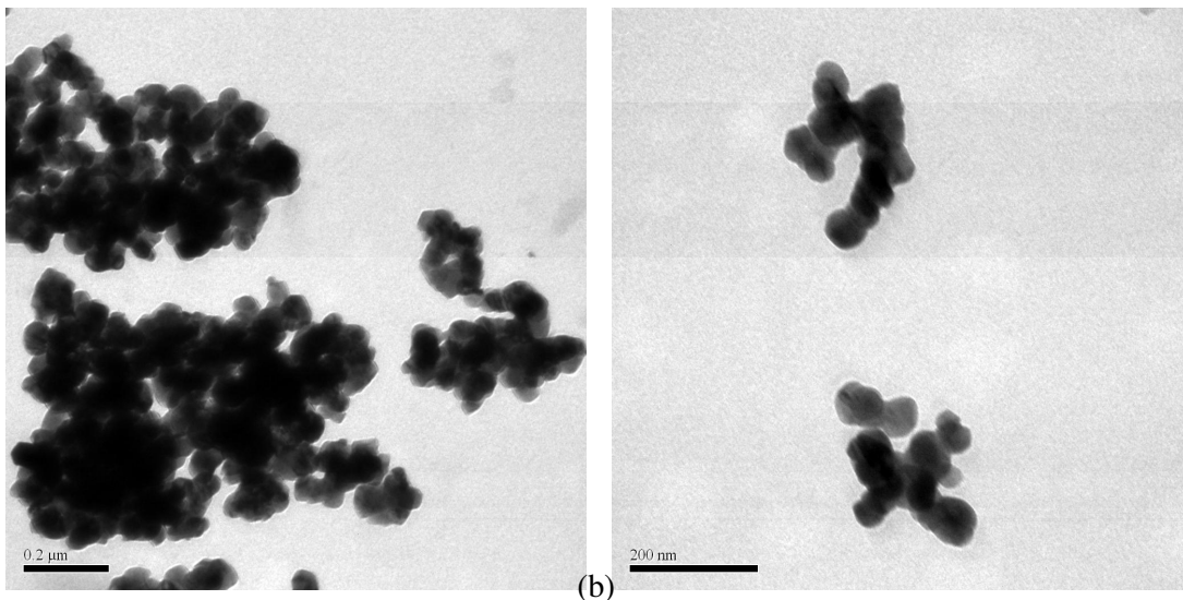
Figura 4.9. (a) Distribuição granulométrica do pó de zircônia comercial, (b) Micrografias obtidas por microscopia eletrônica de transmissão do pó \text{ZrO}_2 : 3% Mol de \text{Y}_2\text{O}_3 comercial utilizado com aumento de 80000X.
