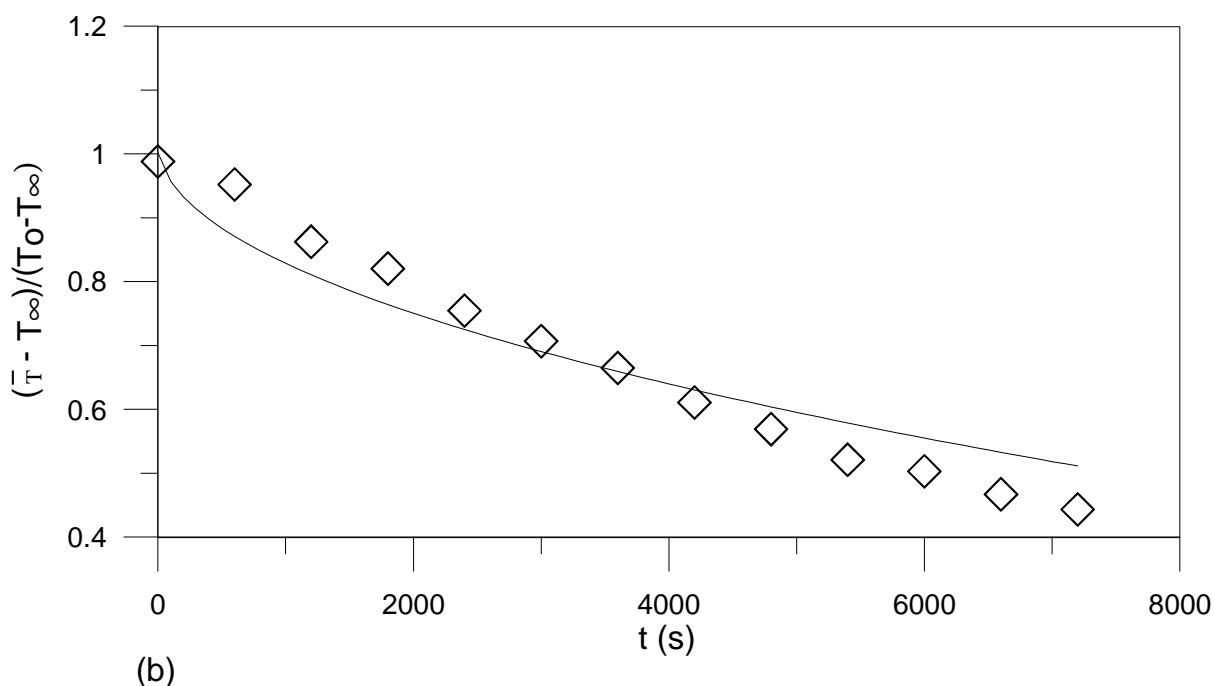
Figura 4.18 – Temperatura adimensional experimental (símbolos) e calculada (linhas) do cilindro de farinha de resíduos (descrito no capítulo de materiais e métodos) ao longo do tempo de ensaio. (a) umidade=3,7% (base úmida); (b) umidade=61,2% (base úmida).
