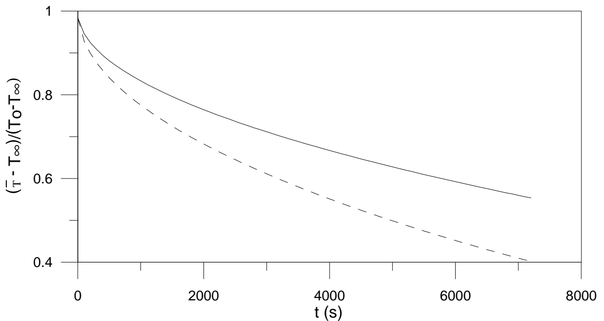
Figura 4.21 – Perfil de temperatura média adimensional ao longo do tempo de amostras de farinha de resíduos com diferentes frações mássicas de gordura. Linha contínua (1%) e linha tracejada (99%)
