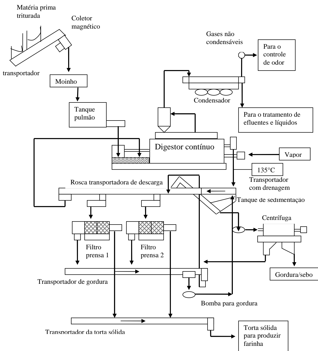
Figura 2.2 – Fluxograma do processamento contínuo da farinha de resíduos.
