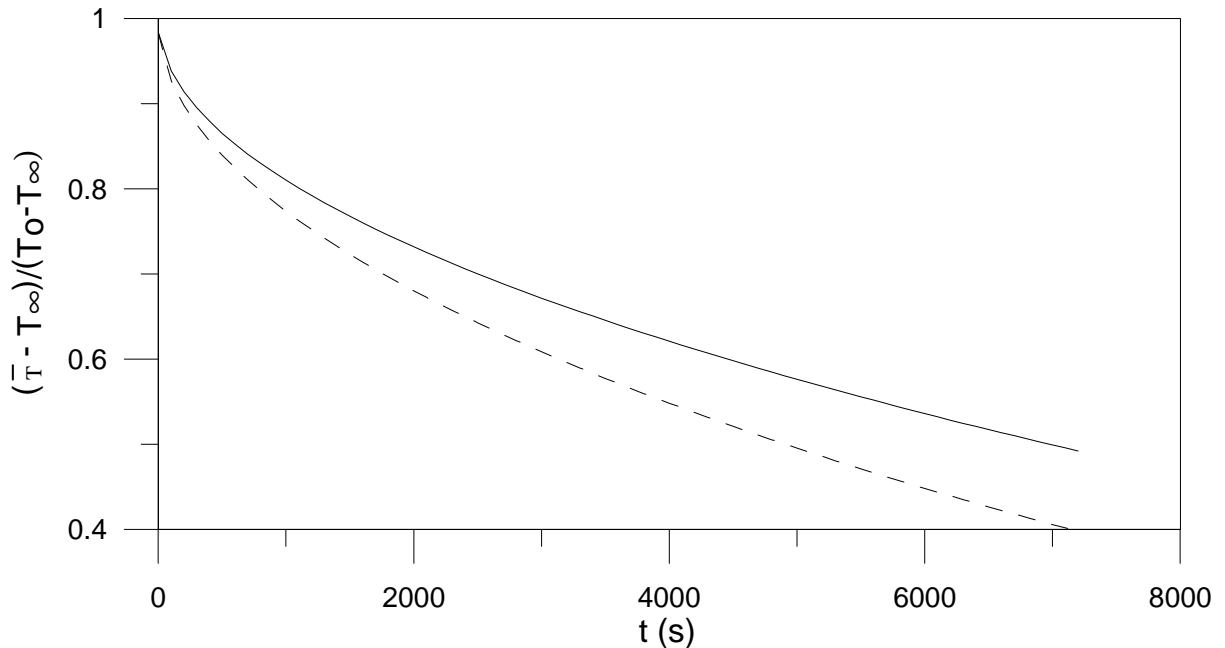
Figura 4.19 – Temperatura média adimensional ao longo do tempo de amostras de farinha de resíduos com diferentes umidades. Linha contínua (1%) e linha tracejada (99%)
