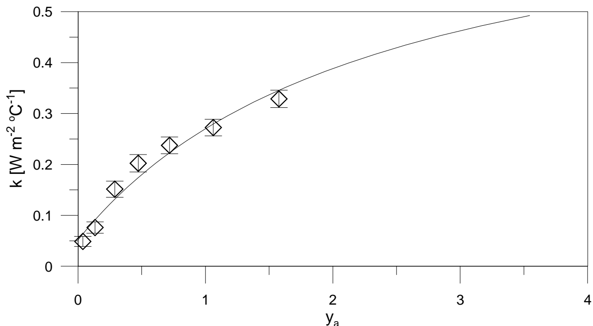
Figura 4.14 – Comparação entre resultados experimentais e calculados de condutividade em diferentes frações mássicas de água.
