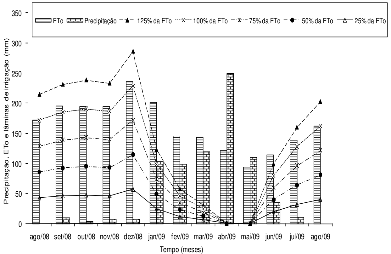
Figura 24. Balanço hídrico do cultivo do pinhão-mansão irrigado com água salina e adubado sob condições de campo
