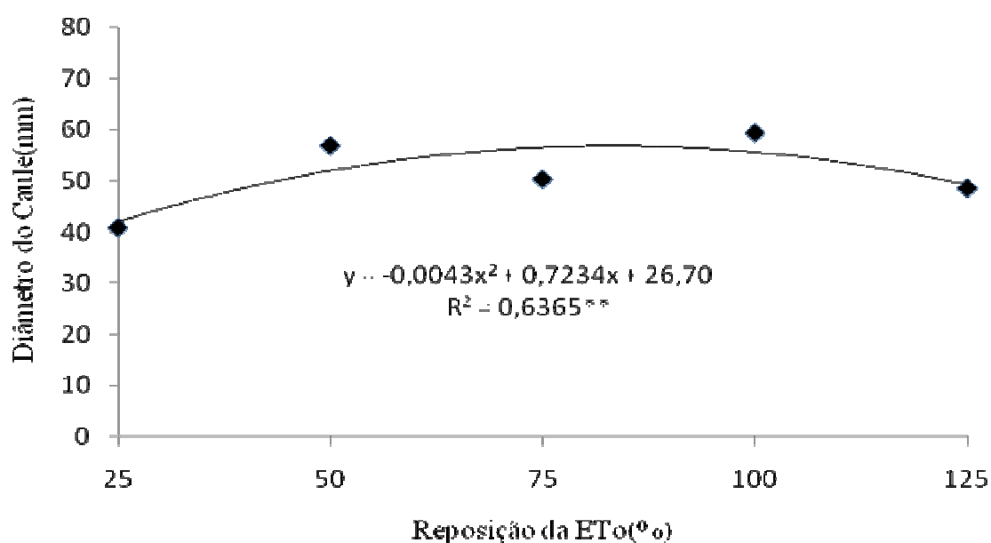
Figura 15. Análise do diâmetro do caule com adubação química em função da reposição da ETo, aos 210 DAT
