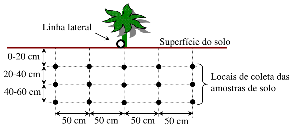
Figura 3. Esquema mostrando a localização de coleta das amostras de solo, para análise de salinidade
