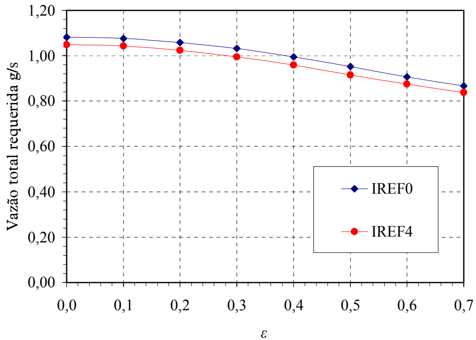
Figura 5.14 – Vazão mássica total em função da excentricidade adimensional, para o coeficiente de descarga Cd = \text{variável} .
