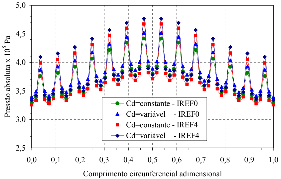
Figura 5.21 – Comparação das pressões absolutas nas posições dos orifícios de abastecimento, excêntrica adimensional \varepsilon = 0,1 .
