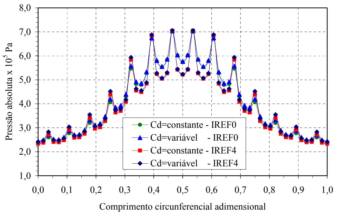
Figura 5.22 – Comparação das pressões absolutas nas posições dos orifícios de abastecimento, excêntrica adimensional \varepsilon = 0,7 .
