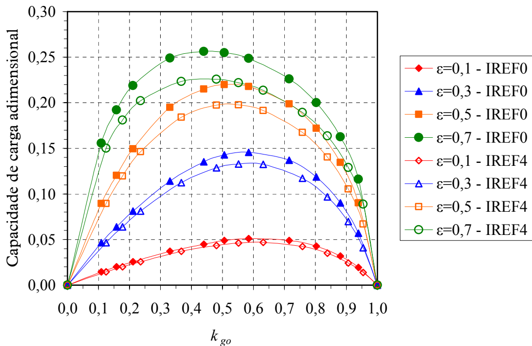
Figura 5.17 – Capacidades de carga adimensional versus k_{go} , comparação entre os resultados da malha de referência IREF0 e com índice de refinamento IREF4, Cd = variável.
