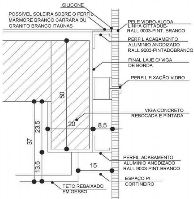
Figura 4.66. Corte do detalhe da fixação da pele de vidro
