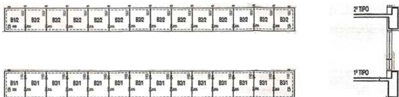
Figura 3.6 - Paginação com elevação e corte das placas pétreas aplicadas em fachadas. Cota
