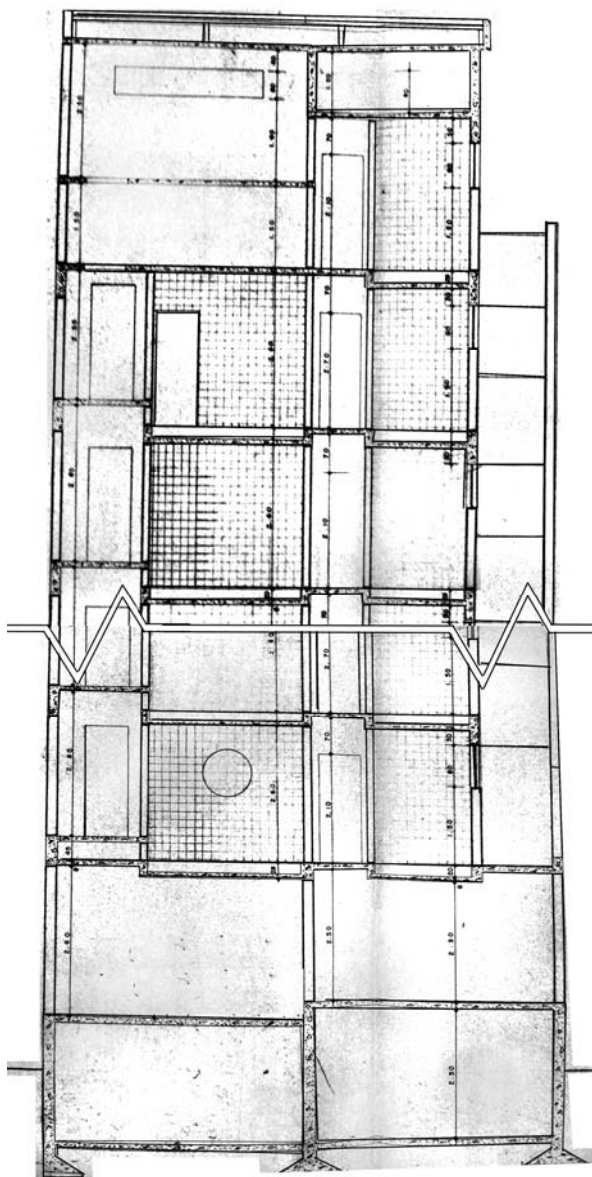
Figura 4.11. Corte transversal do edifício Aldebarã com doze pavimentos
