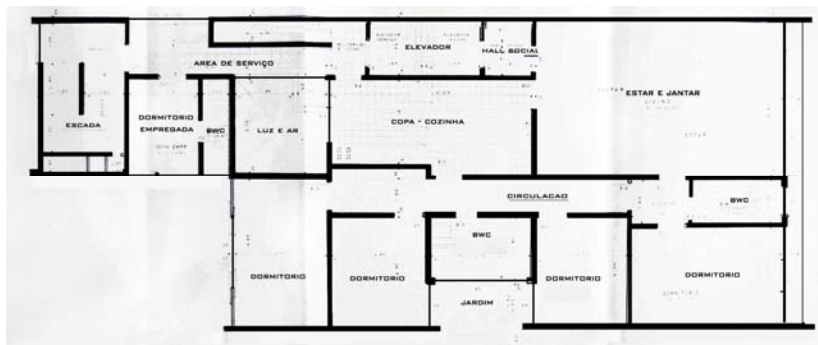
Figura 4.9. Planta baixa do pavimento tipo.
