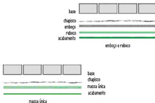
Figura 3.5 - Camadas argamassadas. Fonte: Baía e Sabattini (2000)
