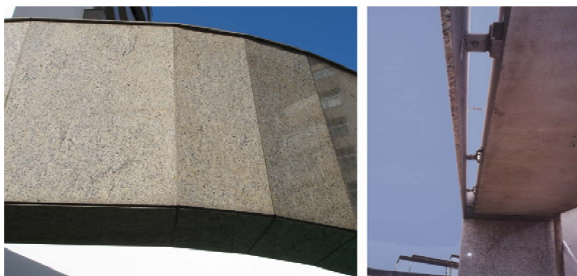
Figura 4.50 a- revestimento pétreo e b- fixação de insertes metálicos
