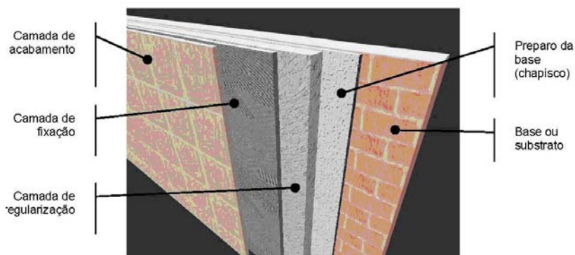
Figura 3.8 - Partes constituintes do revestimento cerâmico aderido. Fonte: Junginger (2003)
