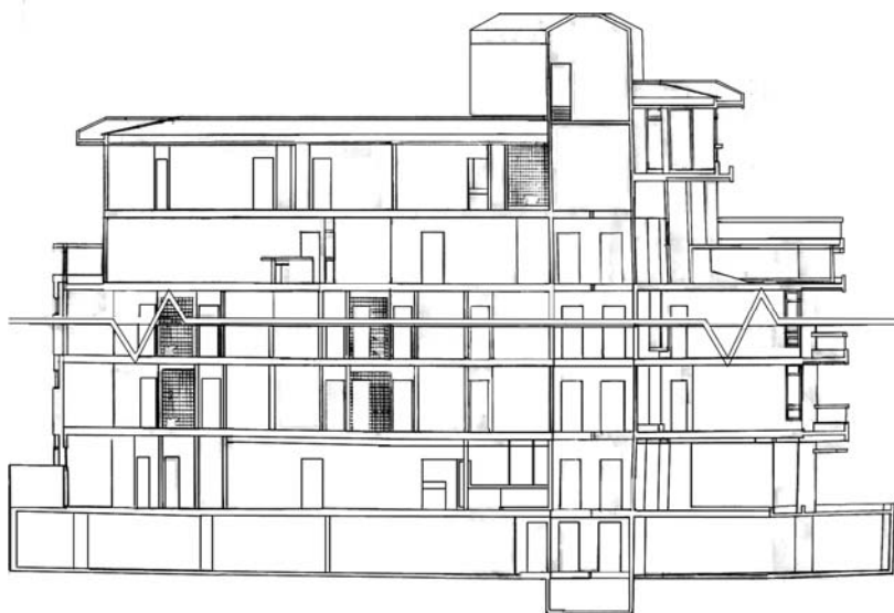
Figura 4.33. Corte longitudinal do edifício Guarazes com dez pavimentos.
