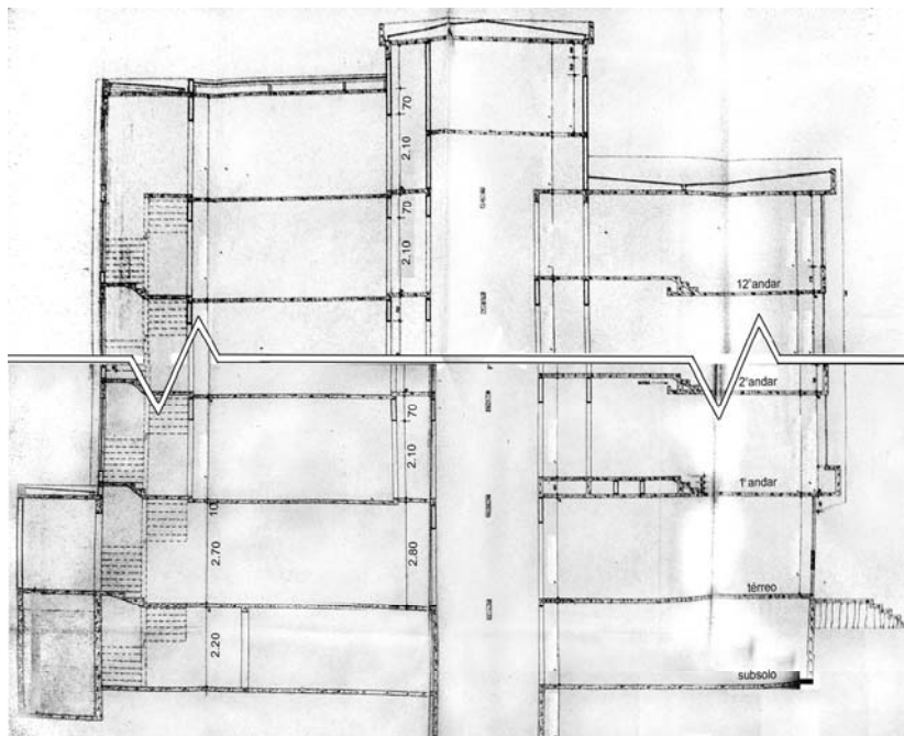
Figura 4.10. Corte longitudinal do edifício Aldebarã com doze pavimentos
