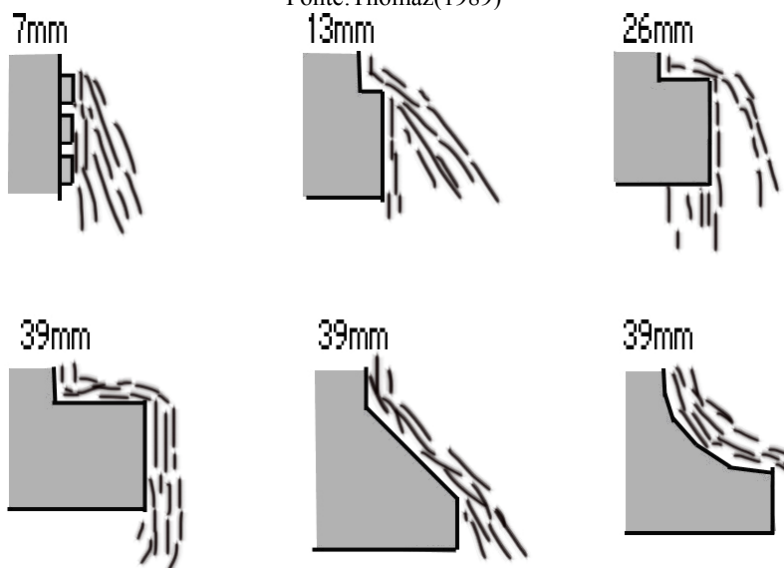
Figura 3.4 - Medidas e projeções nas superfícies das fachadas.
