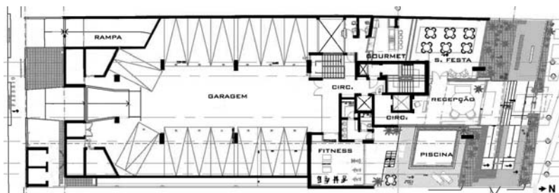
Figura 4.57. Planta de implantação do pavimento térreo.
