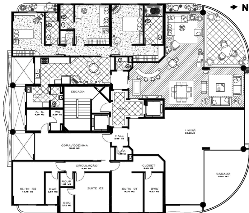
Figura 4.42. Planta baixa tipo padrão do pavimento tipo
