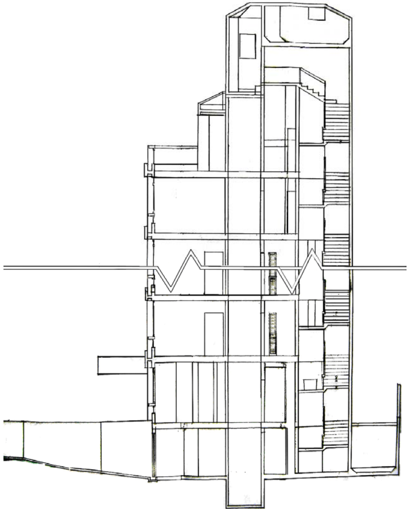
Figura 4.32. Corte transversal do edifício Guarazes com dez pavimentos.
