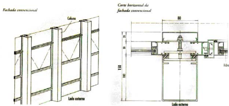
Figura 3.13 - Fachada cortina de vidro. Fonte: Corcuera (1999)
