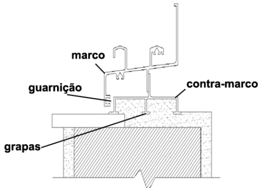
Figura 3.9 - Corte transversal esquemático de uma esquadria. Fonte: Stylo Alumínio (2008)
