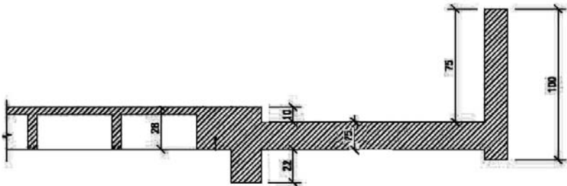
Figura 4.68. Corte da laje maciça da sacada e da laje nervurada dos apartamentos
