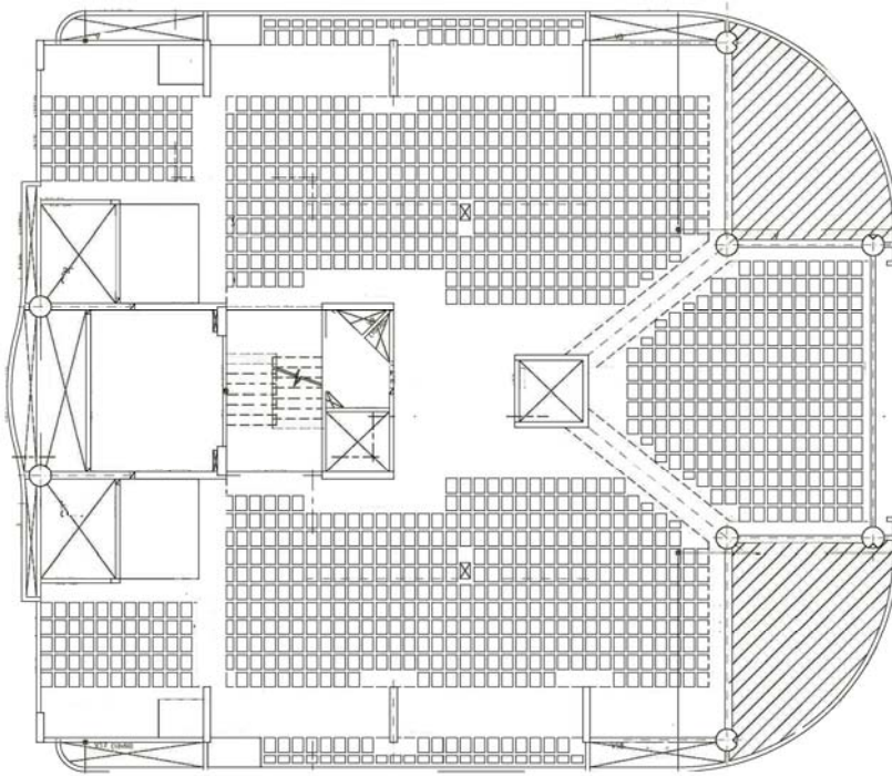
Figura 4.45. Planta estrutural do pavimento tipo.
