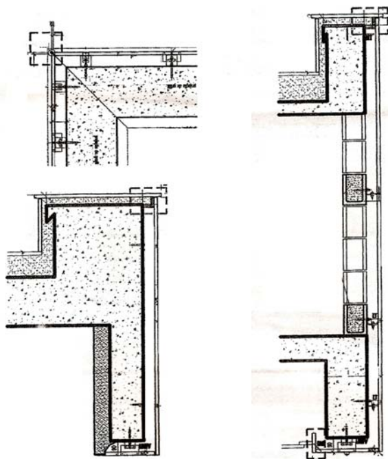
Figura 3.7 - Seção transversal e detalhe das fixações das placas de granito. Fonte: Cota
