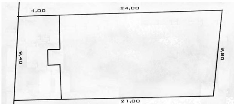
Figura 4.7. Planta de localização do edifício Aldebarã
