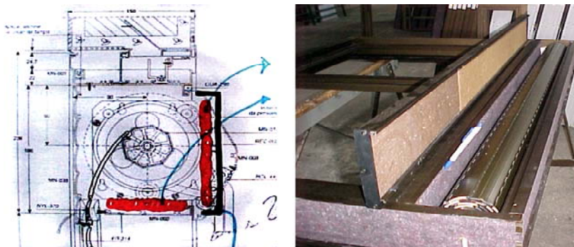
Figura 4.54 a- projeto de produção e b- esquadria com persiana embutida.
