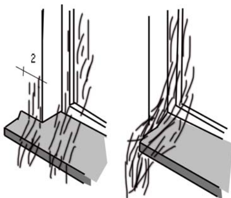
Figura 3.3 - Pingadeira com e sem proteção do fluxo de água da chuva.
