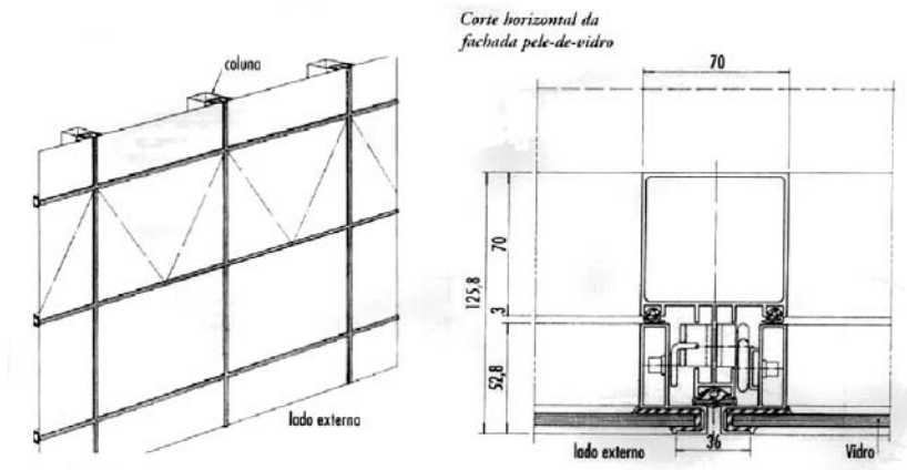
Figura 3.14 - Fachada pele de vidro. Fonte :Corcuera(1999)
