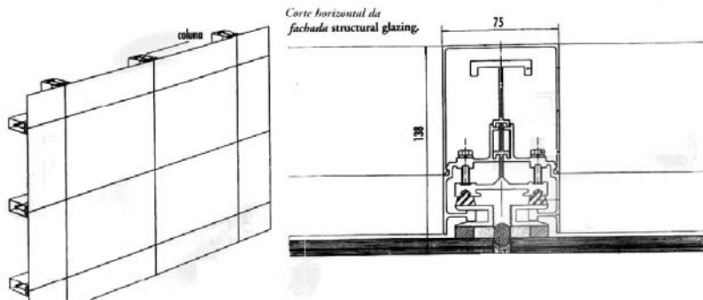
Figura 3.15 - Fachada tipo structural glazing. Fonte: Corcuera (1999)
