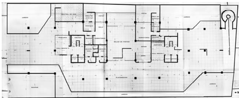
Figura 4.17. Planta de implantação do pavimento térreo.
