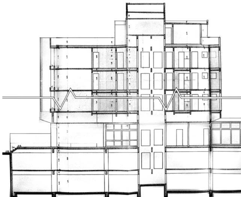
Figura 4.23. Corte longitudinal do edifício Gemini II com onze pavimentos
