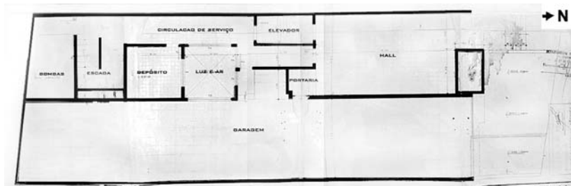
Figura 4.8. Planta de implantação do térreo.
