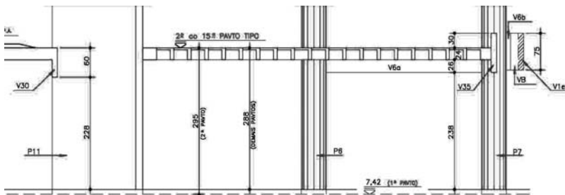
Figura 4.46. Corte do projeto estrutural do pavimento tipo.
