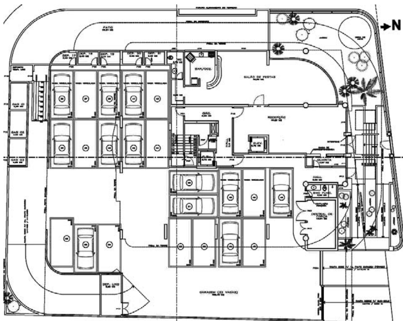
Figura 4.41. Planta de implantação do pavimento térreo.
