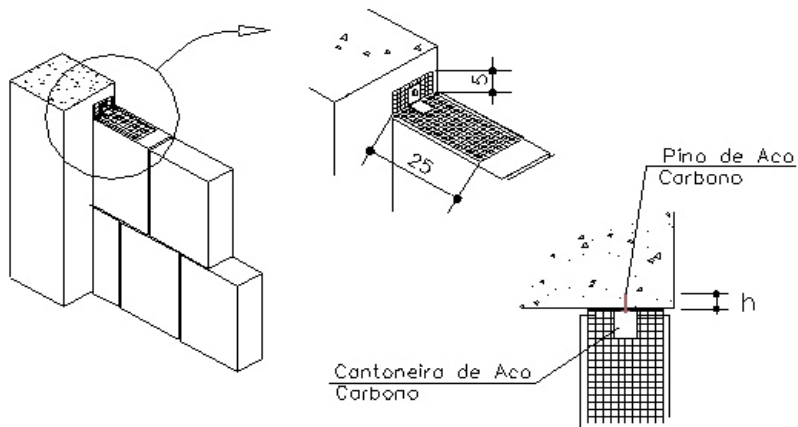
Figura 3.1 - Detalhe de ligação de reforço entre parede e estrutura. Fonte: Franco (1998).
