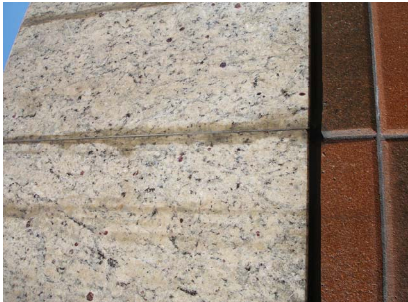
Figura 4.51 Aplicação de silicone no rejunte das placas de granito.
