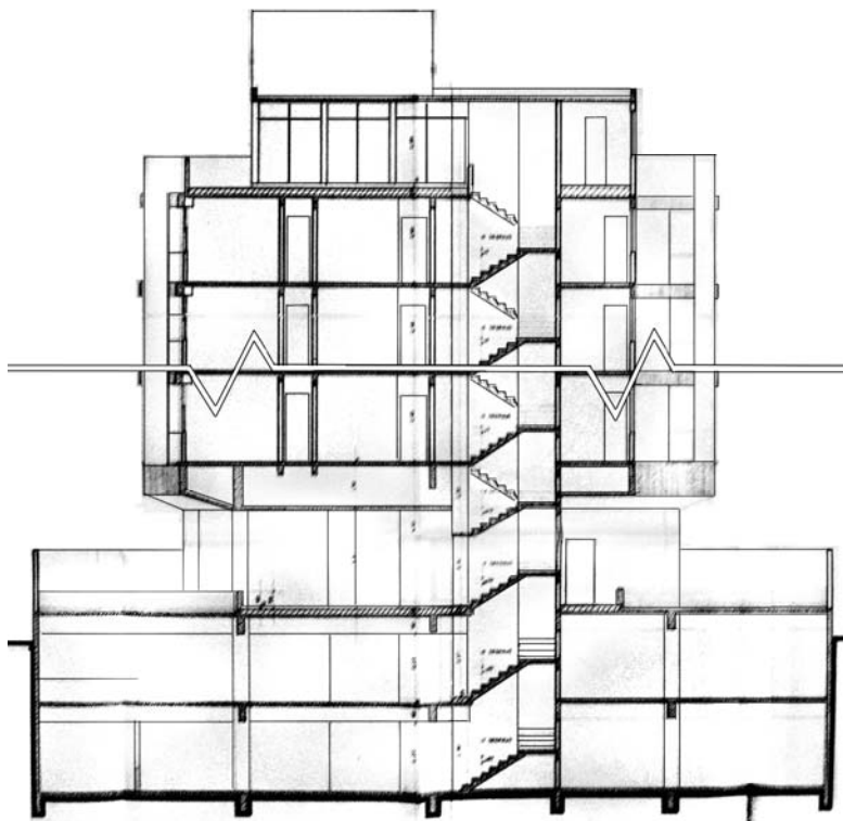
Figura 4.22. Corte transversal do edifício Gemini I com dez pavimentos
