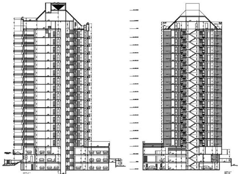
Figura 4.43 a- corte longitudinal e b- corte transversal.
