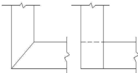
Figura 3.12 - Corte dos perfis em 45 e 90 graus. FONTE: Stylo Alumínio
