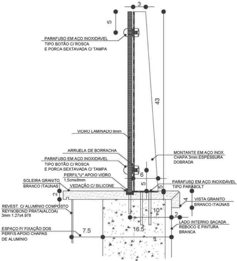
Figura 4.65. Corte longitudinal do guarda-corpo
