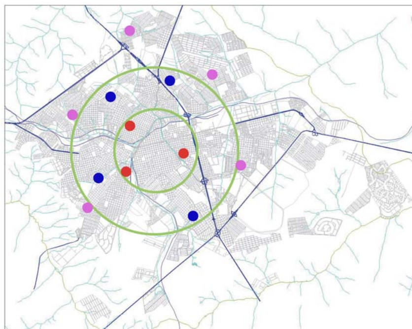
Figura 9: Mapa da cidade de Bauru, divisão dos três setores pelos círculos de cor verde e representação das doze escolas estaduais que fizeram parte do estudo de Ferraz (2006).
