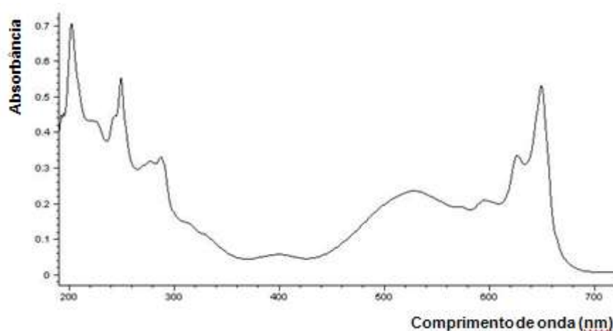
Figura 12: Espectro de U.V do composto 30a
