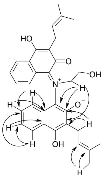
Figura 10: Principais correlações do espectro de COLOC ( J^{\beta} e J^{\alpha} ) de 30a
