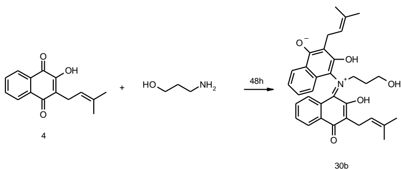
Esquema 14: Acoplamento do 3-amino-1-propanol com o lapachol
