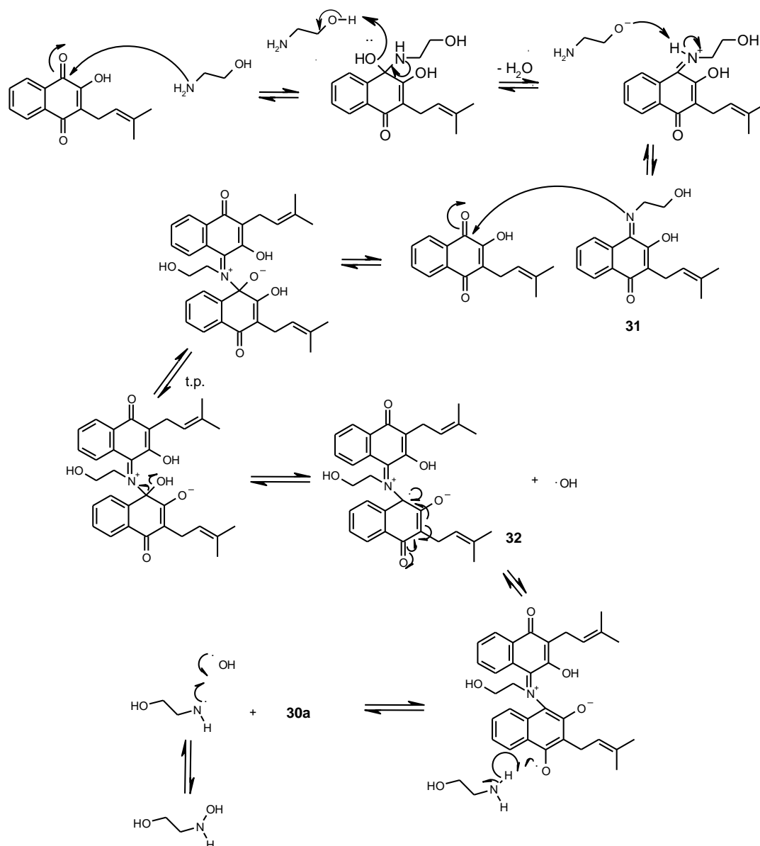
Esquema 12: Proposta mecânica para a formação de 30a
