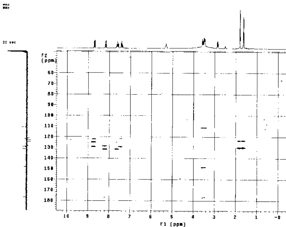
Figura 10: Principais correlações do espectro de COLOC ( J^{\beta} e J^{\alpha} ) de 30a
