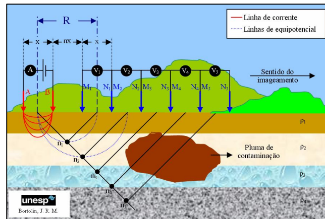
Figura 2.11: Arranjo Dipolo-Dipolo.
