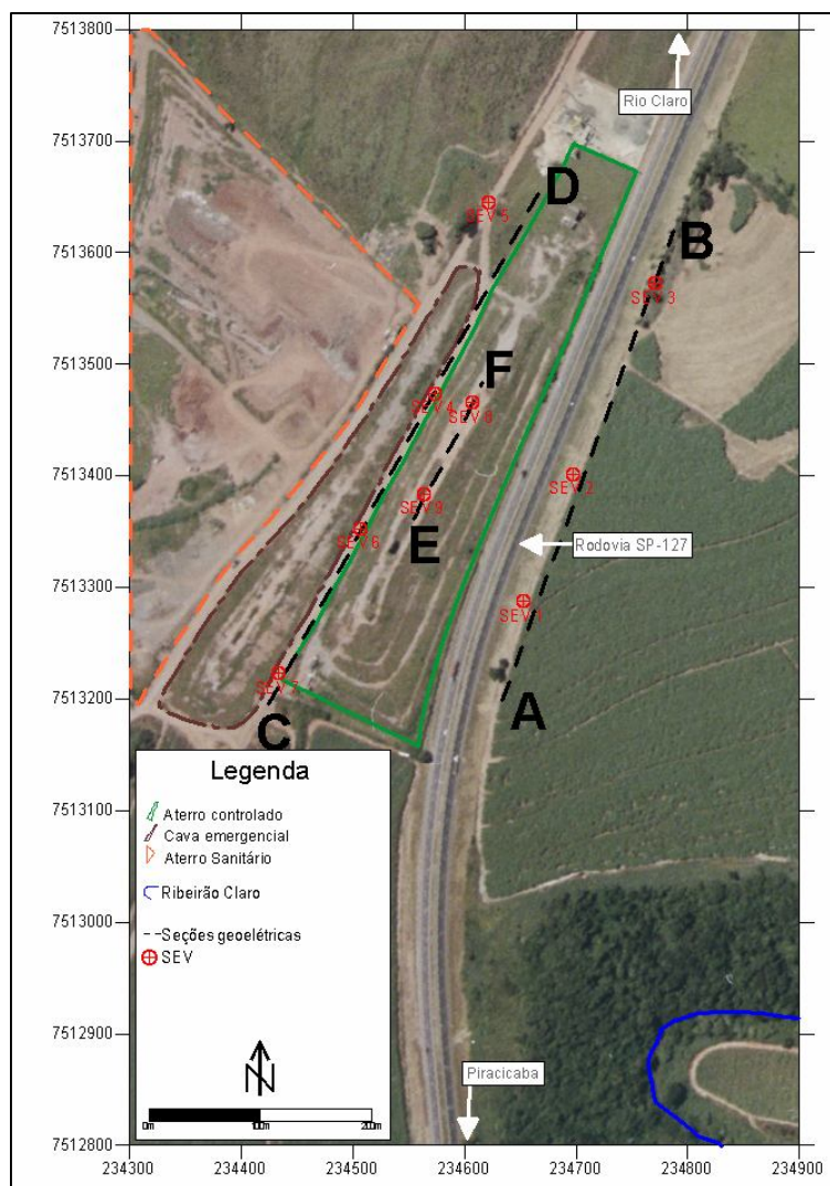
Figura 5.7: Mapa de localização das seções geoeletricas gradadas com base nos dados das SEV.
