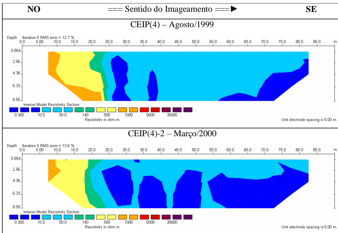
Figura 5.24: Acima: Seção de resistividade aparente do ensaio CEIP(4), realizado no período de estiagem, em Agosto de 1999. Abaixo: Seção de resistividade aparente do ensaio CEIP(4)-2, realizado no período de chuvas, em Março de 2000.
