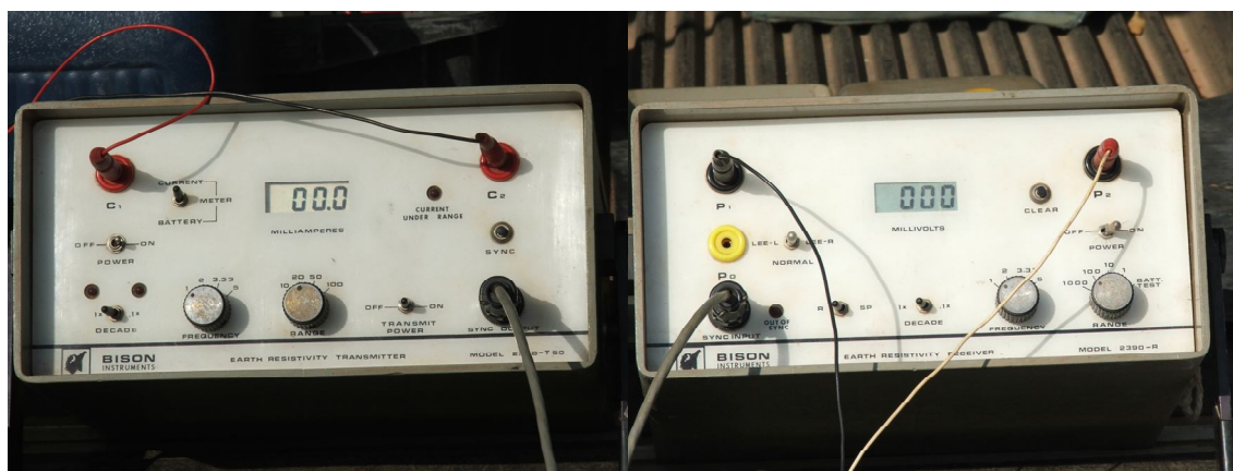
Figura 4.3: Módulo de emissão de corrente BISON 2390 – T 50 (à esquerda) e módulo de medição do potencial BISON 2390 – R (à direita).
