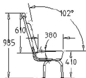
DETALHE POLTRONA ESTOFADA ENCOSTO ALTO
