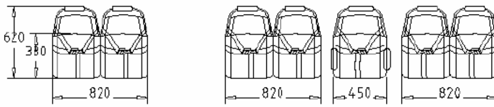
DETALHE DIMENSÕES BANCO TRASEIRO
