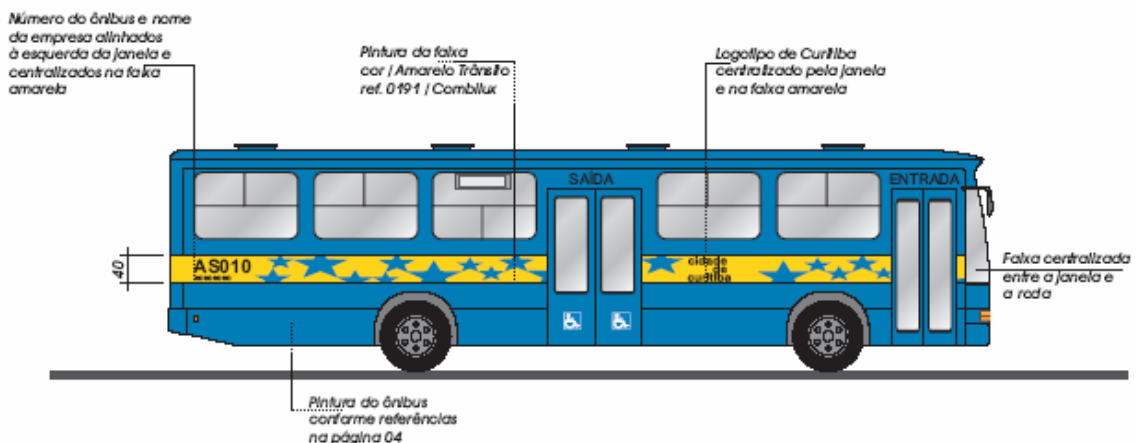
FIGURA 09 – VISTA LATERAL DO ÔNIBUS
