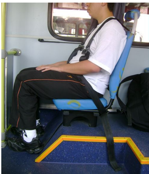
FIGURA 26 - DISTÂNCIA ENTRE ASSENTOS FONTE: FOTO FEITA PELO AUTOR
