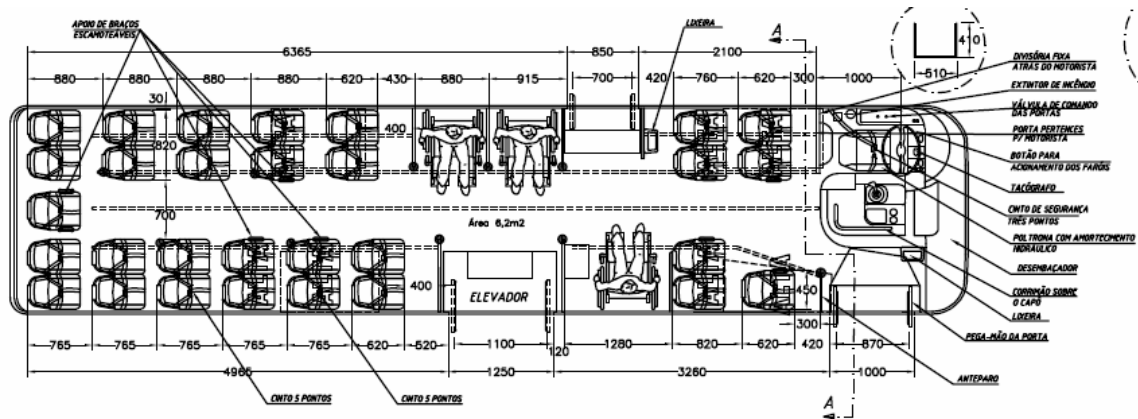
FIGURA 11 – LAY-OUT INTERNO DO ÔNIBUS
