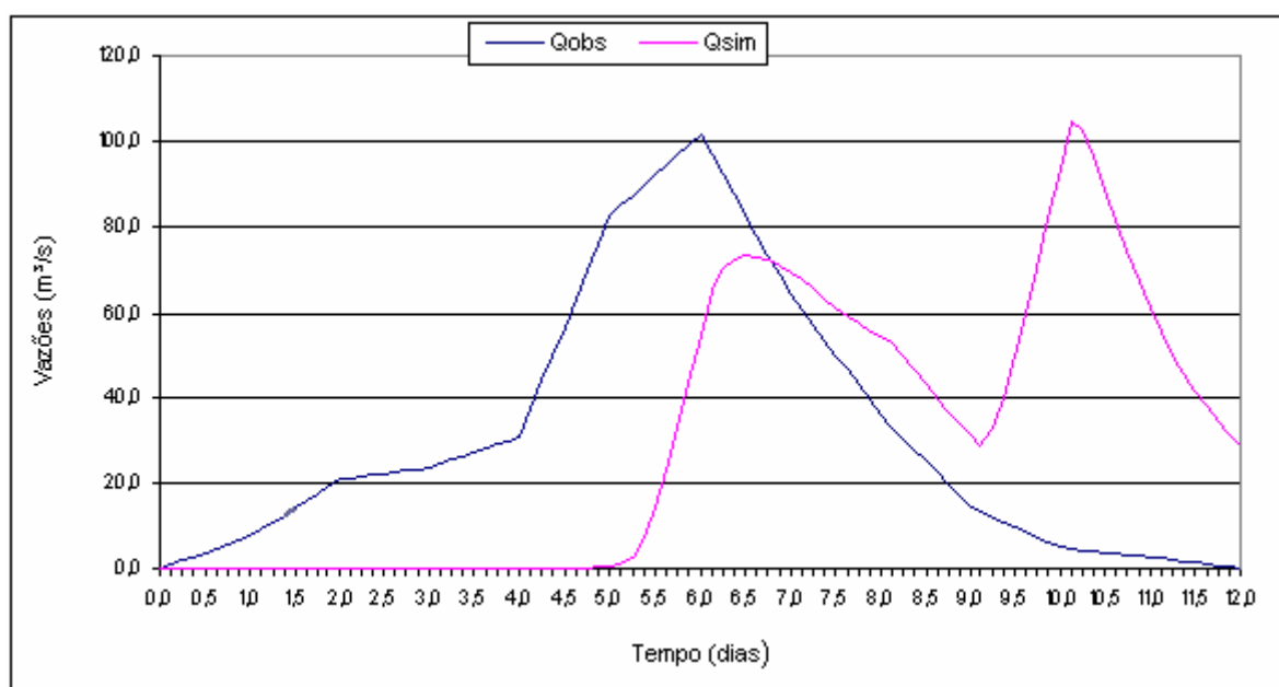
FIGURA D.12 – Simulação para o Evento 2 com uso de todas as funções .
