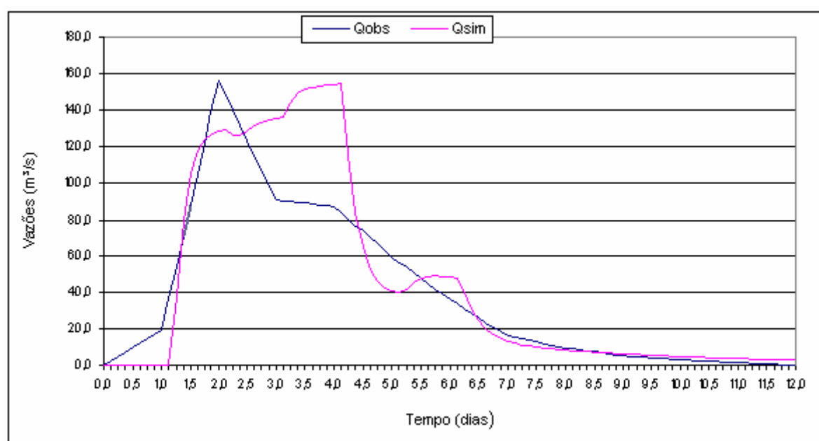
FIGURA D.13 – Simulação para o Evento 3 com uso de todas as funções .
