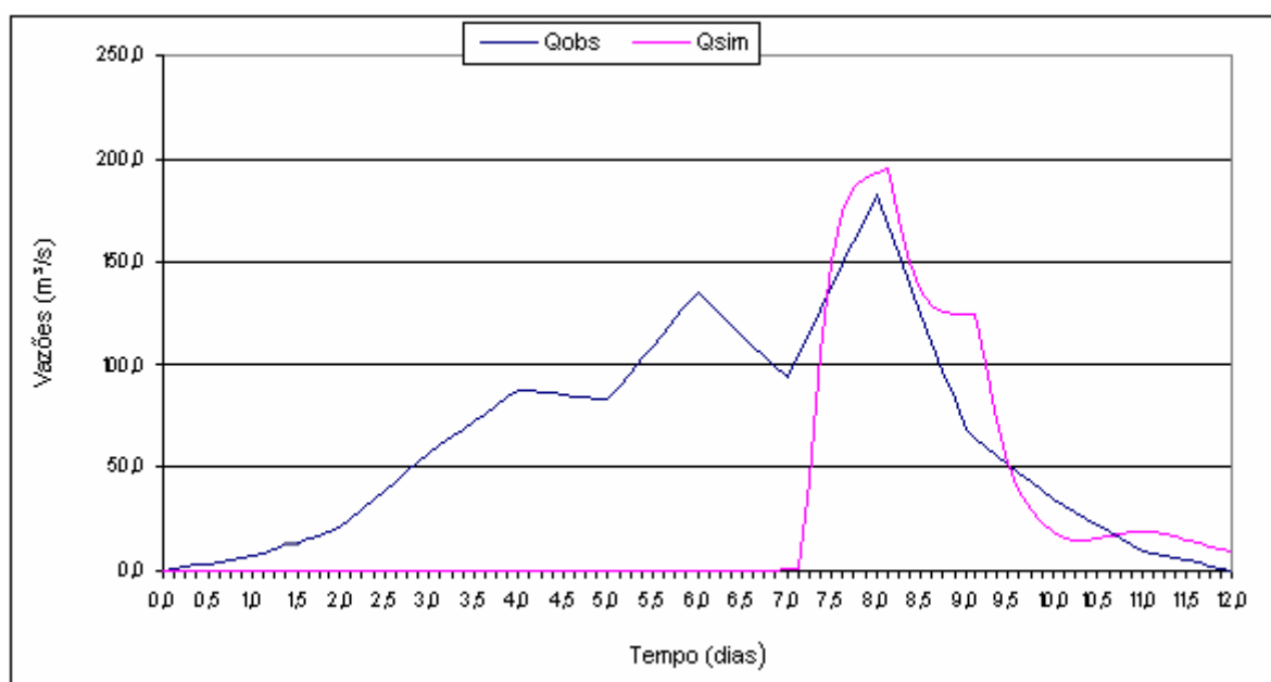
FIGURA D.14 – Simulação para o Evento 4 com uso de todas as funções .
