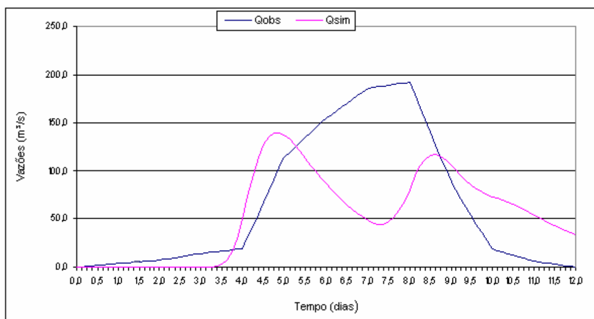
FIGURA D.11 – Simulação para o Evento 1 com uso de todas as funções .
