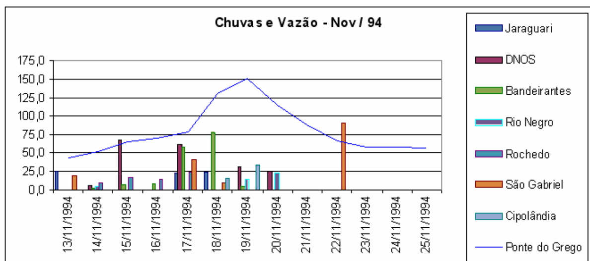
FIGURA B.2 - Dados de chuva e vazão relativos ao Evento 2.
