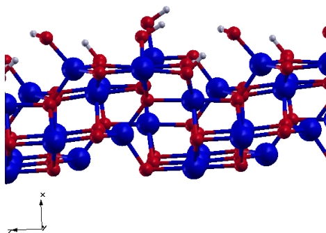
Figura 4.7: Superfície (110) hidratada (8,9
