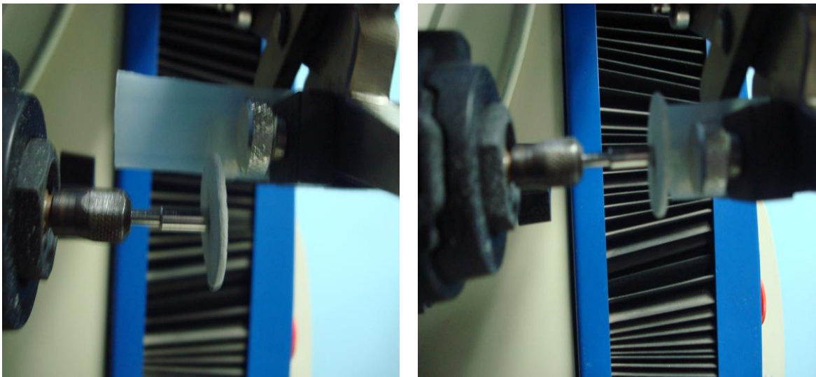
Figura 4.12 – Ensaio de corte de materiais poliméricos com disco cerâmico.
