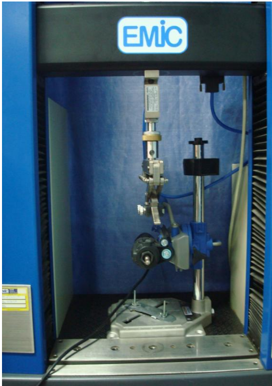
Figura 4.5—Máquina Universal de ensaios mecânicos com o dispositivo adicionado.
