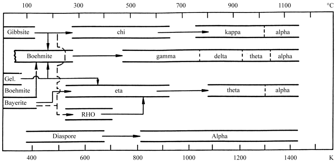
Figura 2.3 – Sequência da transformação térmica dos hidróxidos de alumínio
