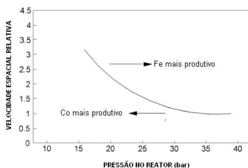
Figura 2.14 - Comparação cinética entre os catalisadores de ferro e cobalto (Espinosa et al. , 1999).
