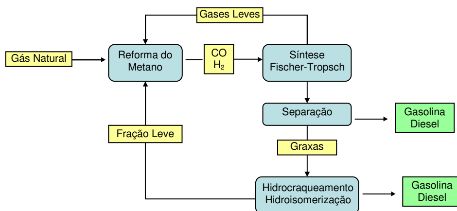
Figura 2.1 - Etapas do Processo de Fischer-Tropsch.
