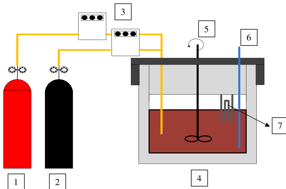
Figura 3.2 - Representação do aparato experimental utilizado na Síntese de Fischer-Tropsch. 1 - Cilindro contendo monóxido de carbono; 2 - Cilindro contendo hidrogênio; 3 - Controladores de fluxo mássico; 4 - Reator de alta pressão; 5 - Sistema de agitação magnética; 6 - Termopar; 7 - Serpentina de refrigeração interna.
