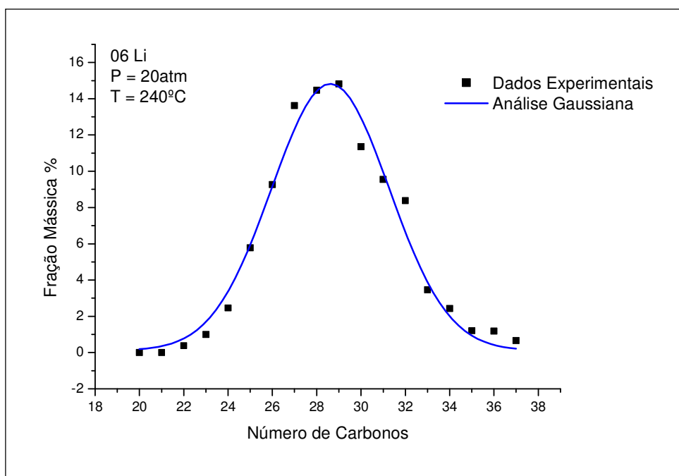
Figura 4.4 - Distribuição dos hidrocarbonetos gerados para o Catalisador 06 Li nas condições operacionais de 20atm e 240°C.
