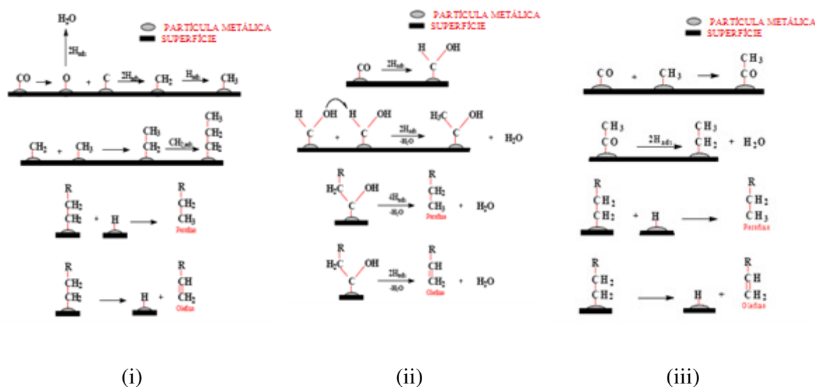
Figura 2.4 - Representação esquemática de três mecanismos básicos de reação de Fischer-Tropsch: (i) mecanismo de carbeno, (ii) mecanismo de hidroxicarbeno e (iii) mecanismo de inserção de CO (Furtado, 2009).
