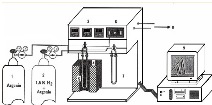
Figura 3.1 - Diagrama esquemático do equipamento utilizado para análises de RTP (Farias, 2007). 1 e 2 - Cilindros de gases; 3 - Controladores de temperatura do forno, das linhas aquecidas e do bloco do TCD; 4 - Forno; 5 - Reator de quartzo contendo a amostra; 6 - TCD; 7 - Saturador com sílica; 8 - Saída dos gases; 9 - Computador para coleta dos dados.
