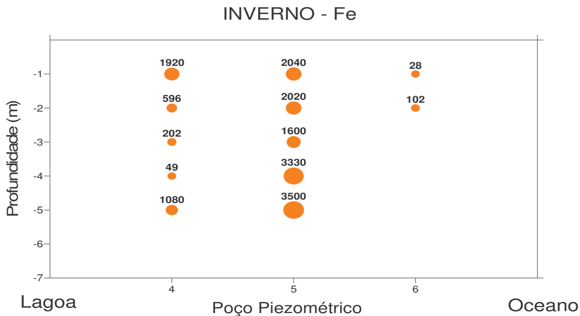
FIGURA 3.18 – Distribuição do ferro ao longo do transecto central da barreira IV para os poços 4, 5 e 6 da Figura 3.9.a.
