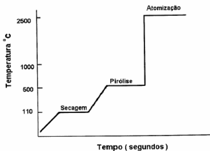
FIGURA 1.3 – Estágios gerais do programa de temperatura (Ficarís, 2004)
