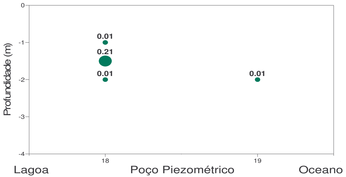
VERÃO - Cu (ppb)
