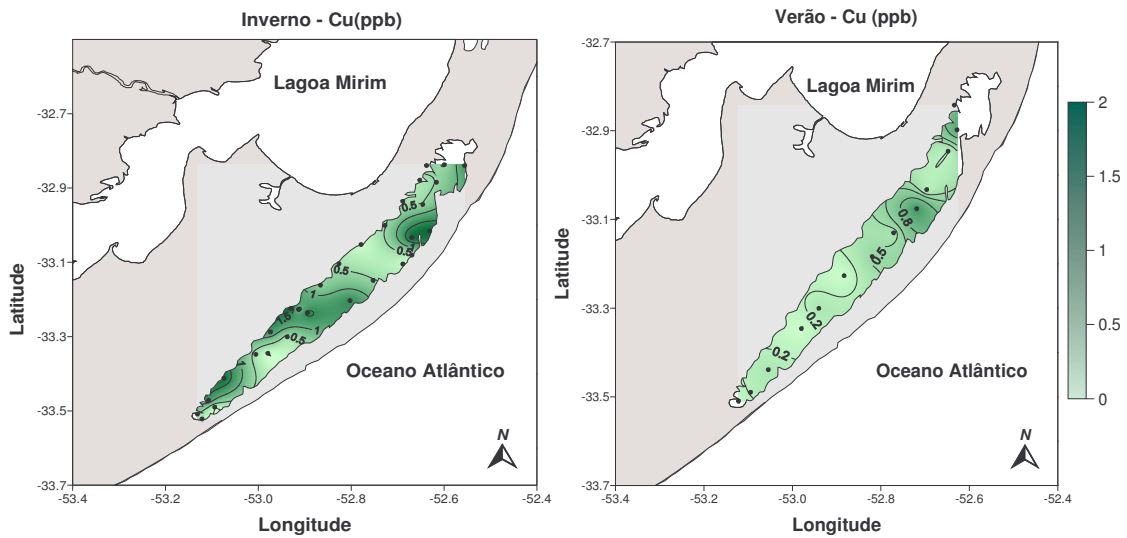
FIGURA 3.30 – Teores de cobre para a Lagoa Mangueira
