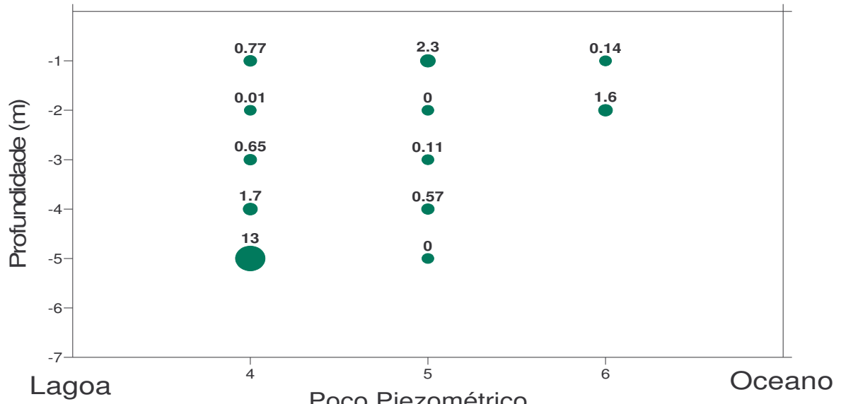
VERÃO - Cu (ppb)
