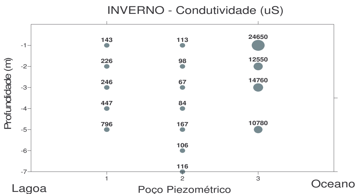
FIGURA 3.16 – Distribuição da condutividade na parte sul para o inverno de 2006 para os poços 1, 2 e 3 da Figura 3.9.a.
