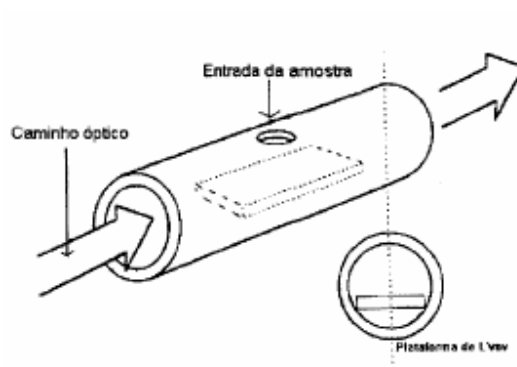
FIGURA 1.2 – Esquema do forno de grafite. Fonte:Ficaris, 2004
