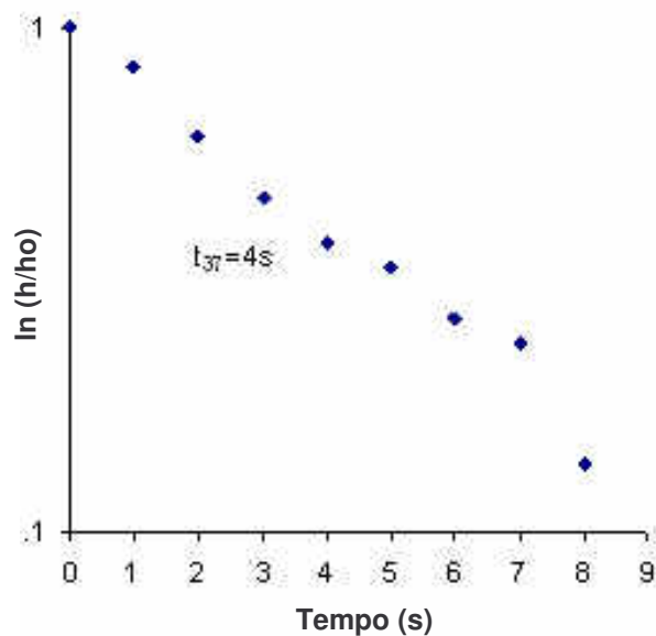
FIGURA 3.38 – Razão entre o nível freático no tempo t sobre o nível freático no tempo 0 (h/ho) em escala logarítmica para o poço permanente
