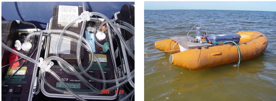
FIGURA 3.12 – Sistema RAD-7 acoplado à embarcação
