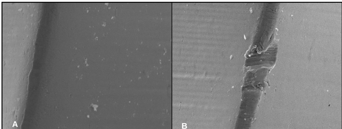
Figuras 10A e 10B – Fotomicrografia da região a 3mm da ponta de uma lima EndoSequence® com aumento de 1000X. (A) antes do uso; (B) após instrumentação
