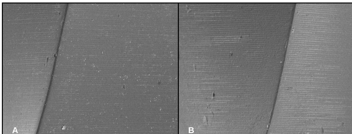
Figuras 14A e 14B – Fotomicrografia da região a 15mm da ponta de uma EndoSequence® com aumento de 190X. A) antes do uso; (B) após instrumentação
