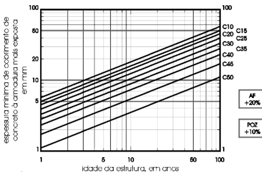
Figura 3.1 – Ábaco para representação da durabilidade em relação aos cobrimentos dos concretos (de C10 a C50) expostos a carbonatação.
