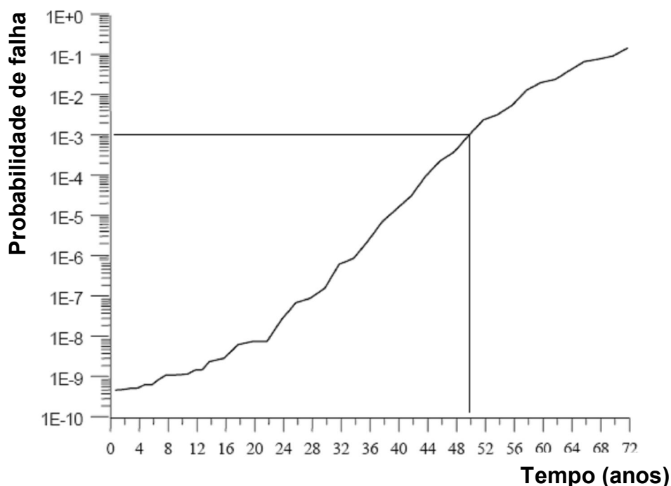
Figura 5.4 – Gráfico de probabilidade de falha em função do tempo.
