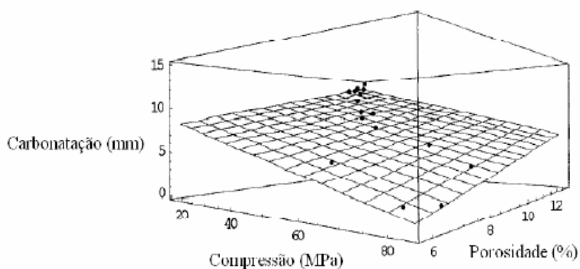
Figura 2.7 – Gráfico tridimensional da relação entre profundidade de carbonatação, resistência mecânica e porosidade.
