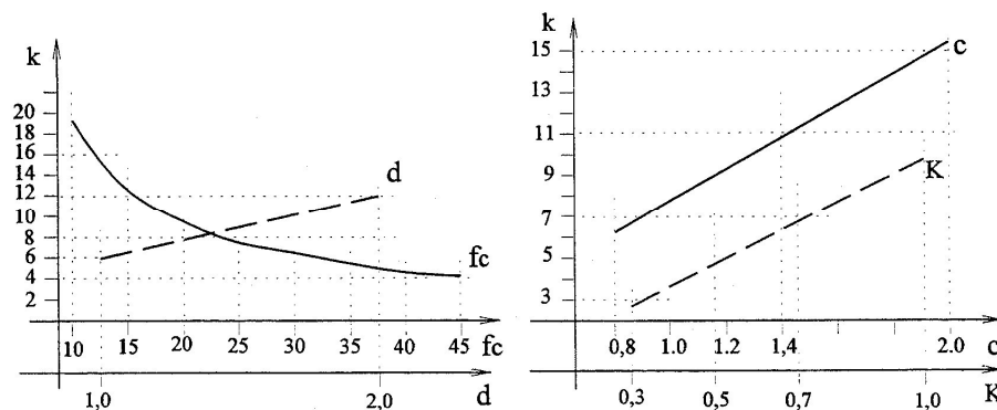
Figura 7.2 – Influência das variáveis na carbonatação no modelo de Bob e Bob.
