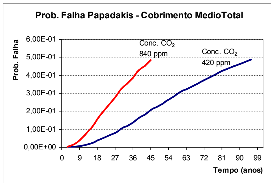
Figura 7.4 – Probabilidade de falha pelo modelo de Papadakis (1992).
