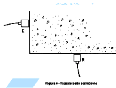
Figura 4.5 – Transmissão semi-direta.
