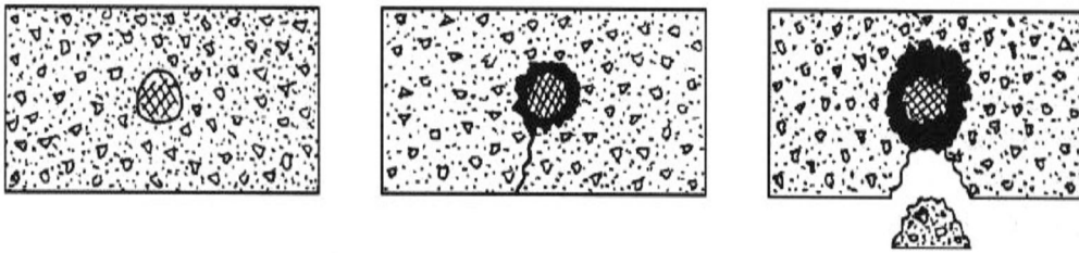
Figura 2.1 – Esquema ilustrativo do processo de deterioração do concreto armado. Fonte: (GENTIL, 2007)
