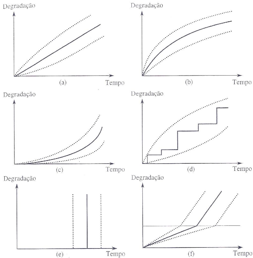
Figura 3.3 – Modelos genéricos de processos de degradação.
