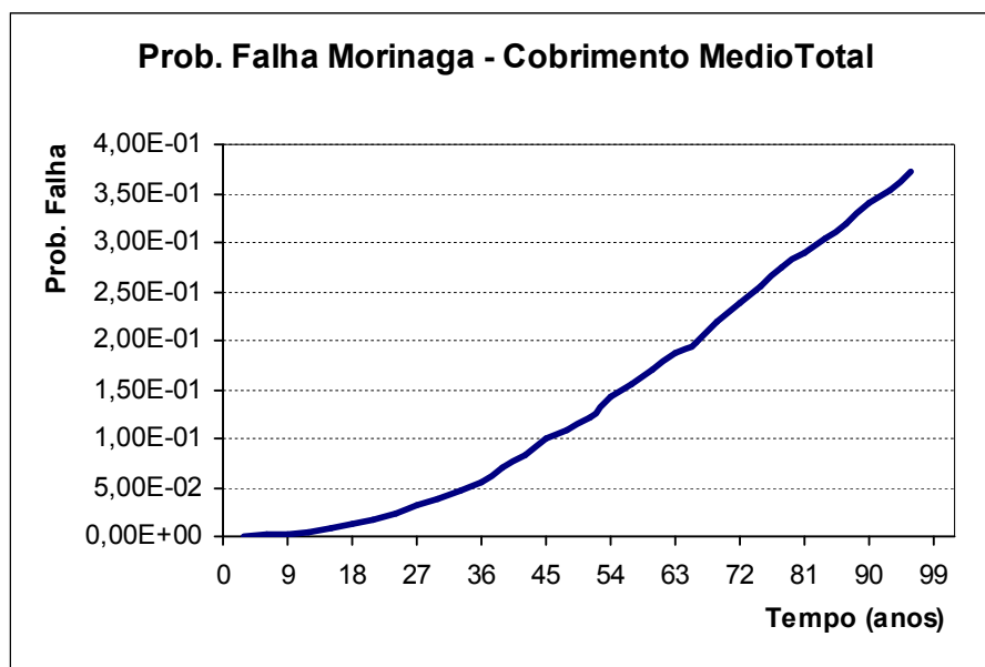
Figura 7.5 – Probabilidade de falha pelo modelo de Morinaga (1990).
