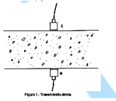
Figura 4.4 – Transmissão direta.
