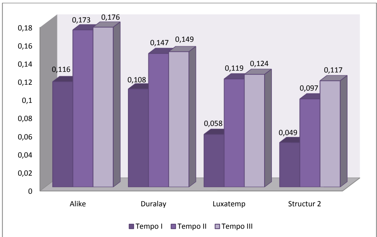
Figura 36 – Valores médios de rugosidade de superfície (Ra) das resinas (µm)
