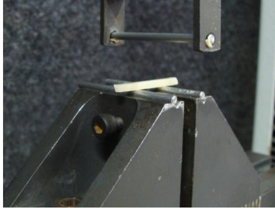
Figura 18 – Corpos-de-prova colocados sobre os suportes metálicos CP sobre os apoios
