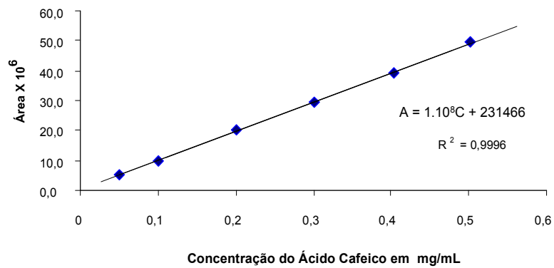
Figura 23. Gráfico da curva de calibração para o padrão de ácido cafeíco.
