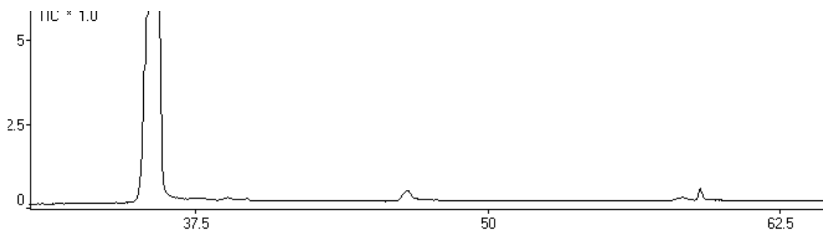
Figura 35. Cromatograma em diclorometano de CG/EM do extrato da borra de café ( Coffea arabica ) do cerrado mineiro.
