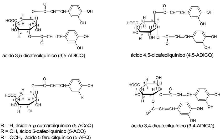
Figura 4. Estrutura dos ácidos clorogênicos
