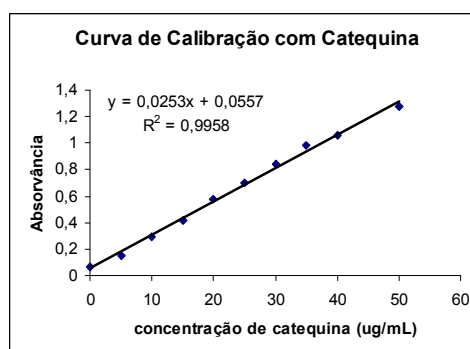
Figura 15. Gráfico da curva de calibração com Catequina.
