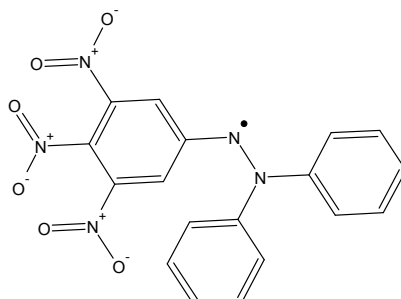
Figura 6. Estrutura do radical estável DPPH •
