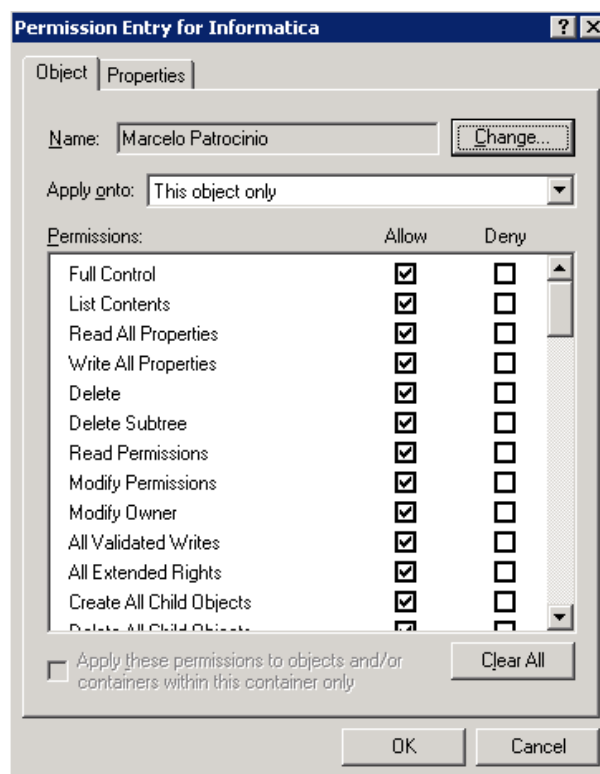
Figura 5: Aplicação de permissões no serviço de diretório. Fonte: Microsoft Active Directory.
