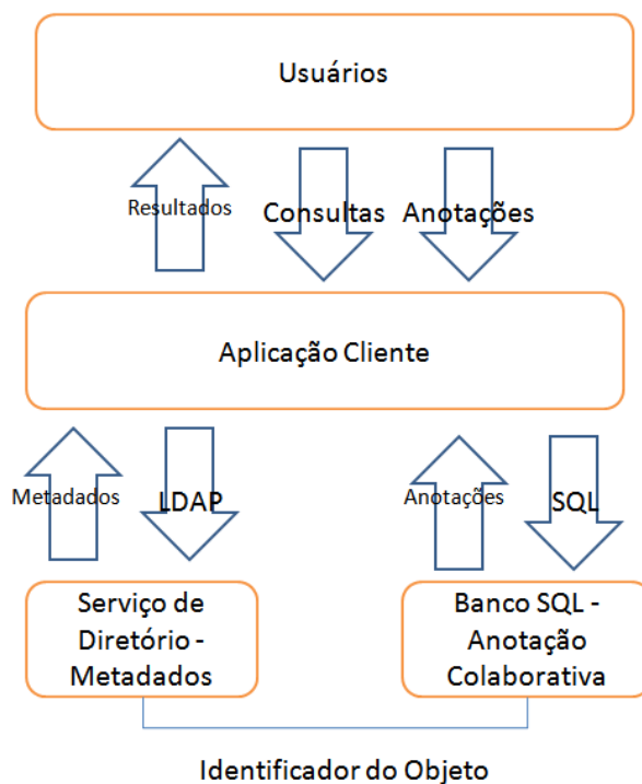
Figura 9: Inclusão de usuário no serviço de diretório.
