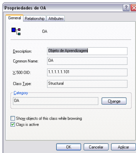
(b) Criação da Classe OA
