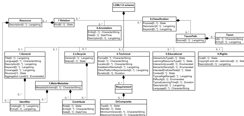
Figura 2: Diagrama da estrutura de classes, relacionamentos e propriedades base do LOM.
