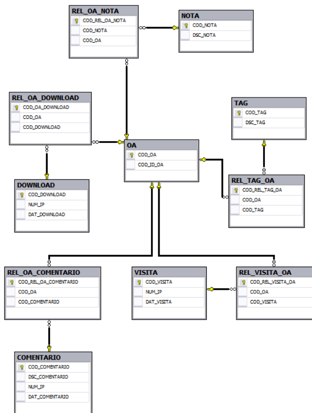
Figura 14: Diagrama do Banco de Dados SQL Utilizado para Anotações. Fonte: Do autor.
