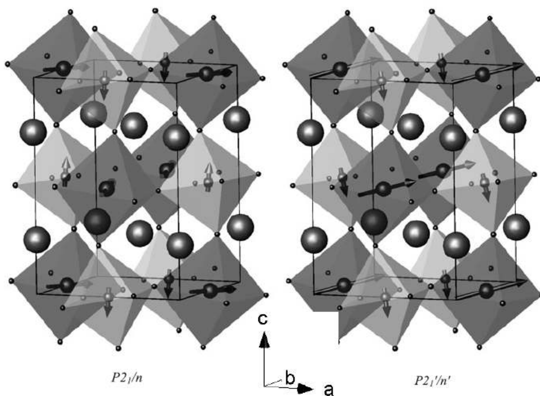
Figura 4.13 - Arranjo dos spins do \text{Mn}^{+2} e do \text{Re}^{+6} no \text{Sr}_2\text{MnReO}_6 de acordo com os dois modelos propostos por Popov et al . Os octaedros mais escuros contêm Mn, que tem momento magnético maior.
