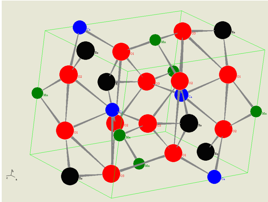
Figura 4.3 - Estrutura cristalina da perovskita gerada pelo PowderCell.
