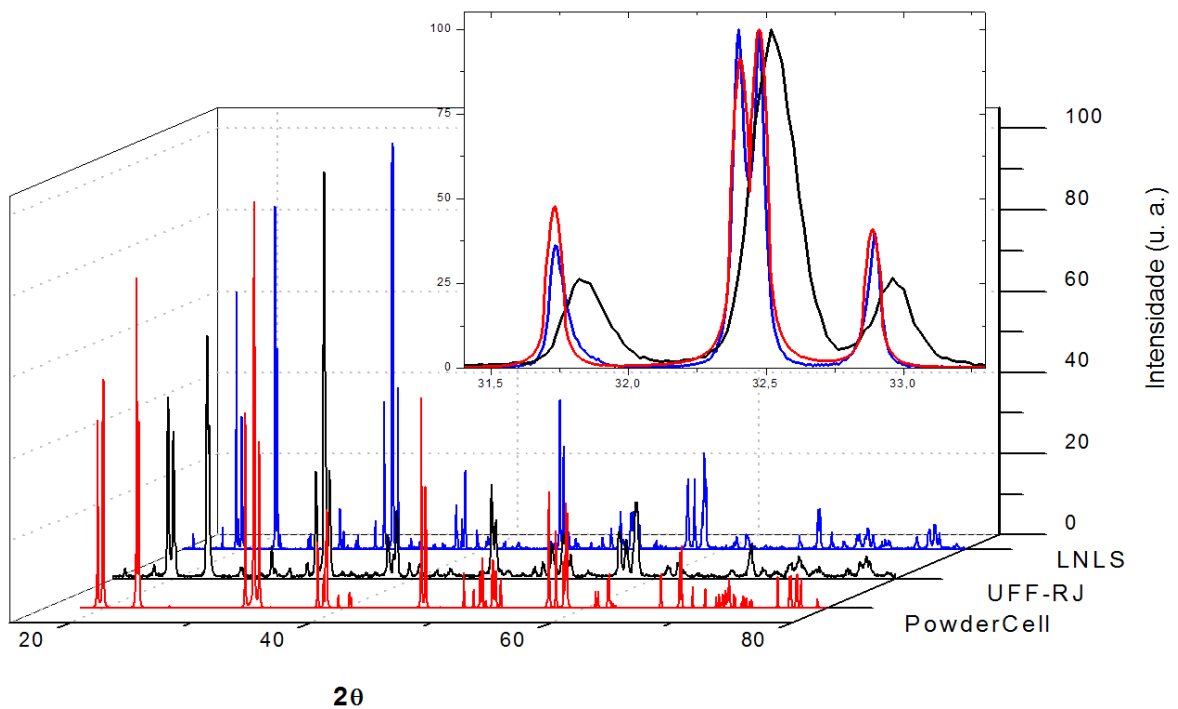
Figura 4.4 - Padrão de difração calculado e medido para a dupla perovskita. No “inset” nota-se a maior resolução e alinhamento do padrão feito no LNLS.
