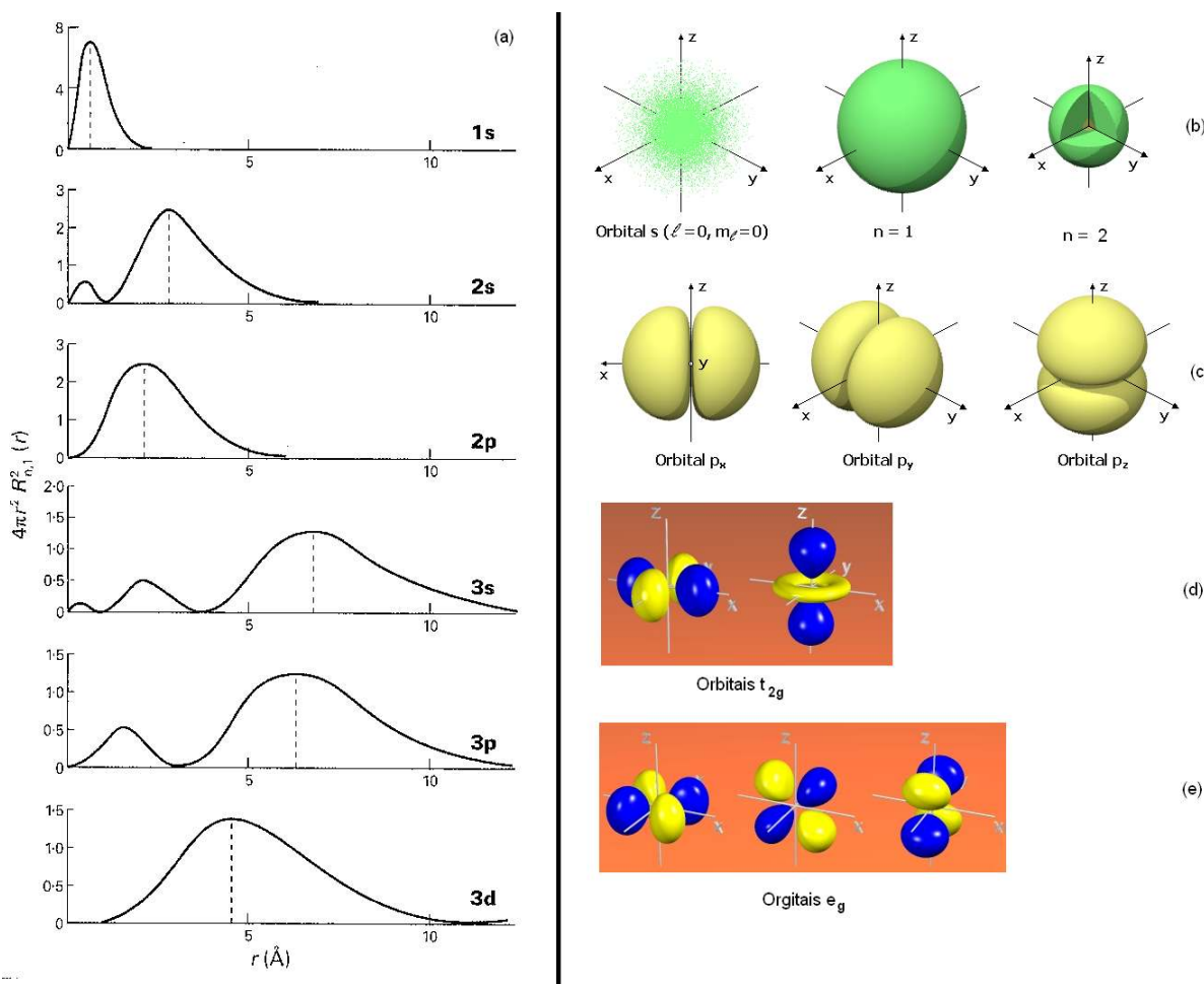
Figura 2.2 - (a) Funções de onda radiais [25]. Orbitais atômicos: (b) orbital s, para n=1 e n=2 ; (c) orbitais p [27]; (d) orbitais 3d_{x^2-y^2} à esquerda e 3d_{z^2} à direita; (e) orbitais 3d_{xy} , 3d_{xz} e 3d_{yz} , respectivamente [28].
