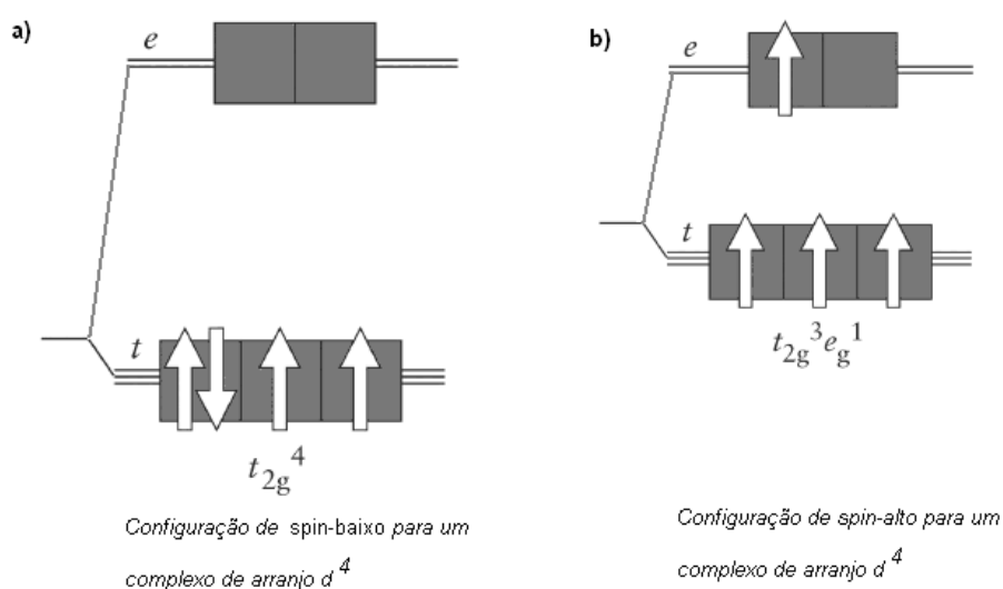
Figura 2.8 - Complexos de spin alto e spin baixo. a) arranjo d^4 de spin alto (campo ligante fraco); b) arranjo d^4 de spin baixo (campo ligante forte).
