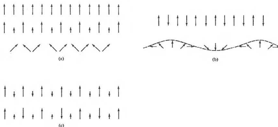
Figura 3.2 - Arranjos ordenados dos spins dos elétrons, (a) ferromagnético; mostrando o tipo canted como caso particular de ferromagnetismo, (b) antiferromagnético; mostrando o tipo helicoidal como caso particular do antiferromagnetismo e (c) ferrimagnético [80].
