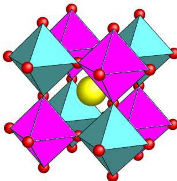
Figura 2.9 - Estrutura cristalina da dupla perovskita mostrando os octaedros compartilhados [9].
