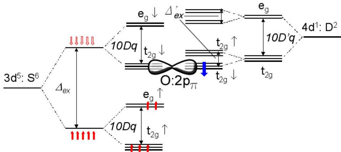
Figura 2.11 - Diagrama esquemático dos níveis de energia de \text{Sr}_2\text{FeMoO}_6 . O nível de Fermi está na banda formada exclusivamente pelas sub-bandas Fe ( t_{2g} \downarrow ) – O ( 2p ) – Mo ( t_{2g} \downarrow ) [39]. O símbolo \Delta_{\text{ex}} representa a energia de troca (emparelhamento de elétrons).
