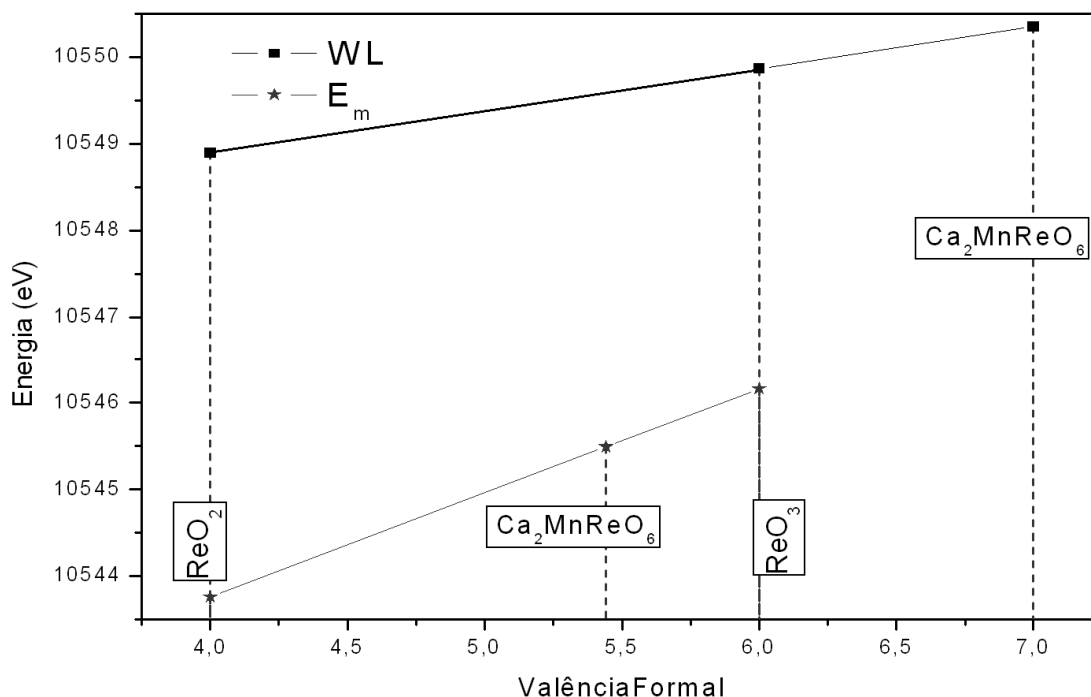
Figura 4.9 - Valores dos primeiros momentos ( E_m ) calculados e posições das WL para os compostos envolvidos na XAS.
