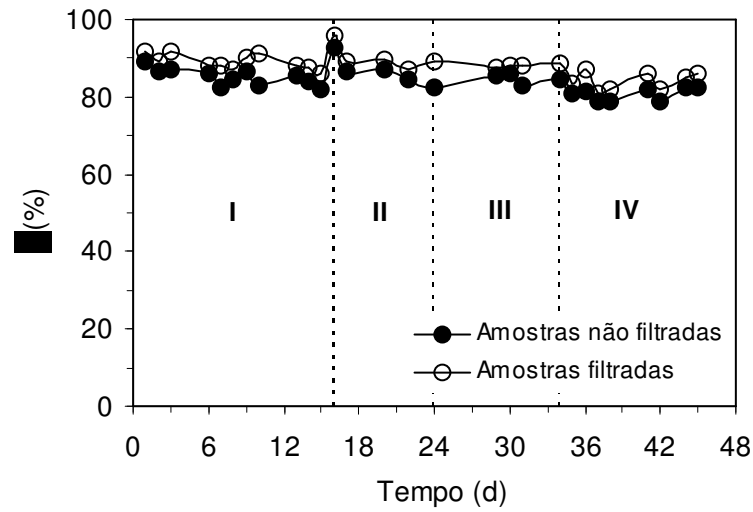
Figura 4. 11 – Eficiência de remoção de matéria orgânica na operação com 1000 mgDQO/L (I: 0,5 g NaHCO 3 /L; II: 0,8 g NaHCO 3 /L; III: 1,0 g NaHCO 3 /L; IV: 1,5 gNaHCO 3 /L)
