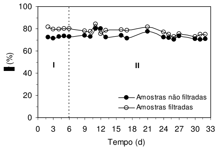
Figura 4. 58 – Eficiência de remoção de matéria orgânica na operação com 2000 mgDQO/L: alimentação em batelada (I) e alimentação em batelada alimentada durante 4 horas (II)
