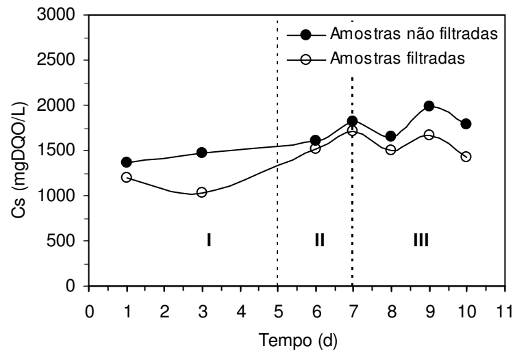
Figura 4. 30 – Concentração de matéria orgânica na operação com 3000 mgDQO/L (I: 4,5 g NaHCO 3 /L; II: 6,0 g NaHCO 3 /L; III: 8,0 g NaHCO 3 /L)
