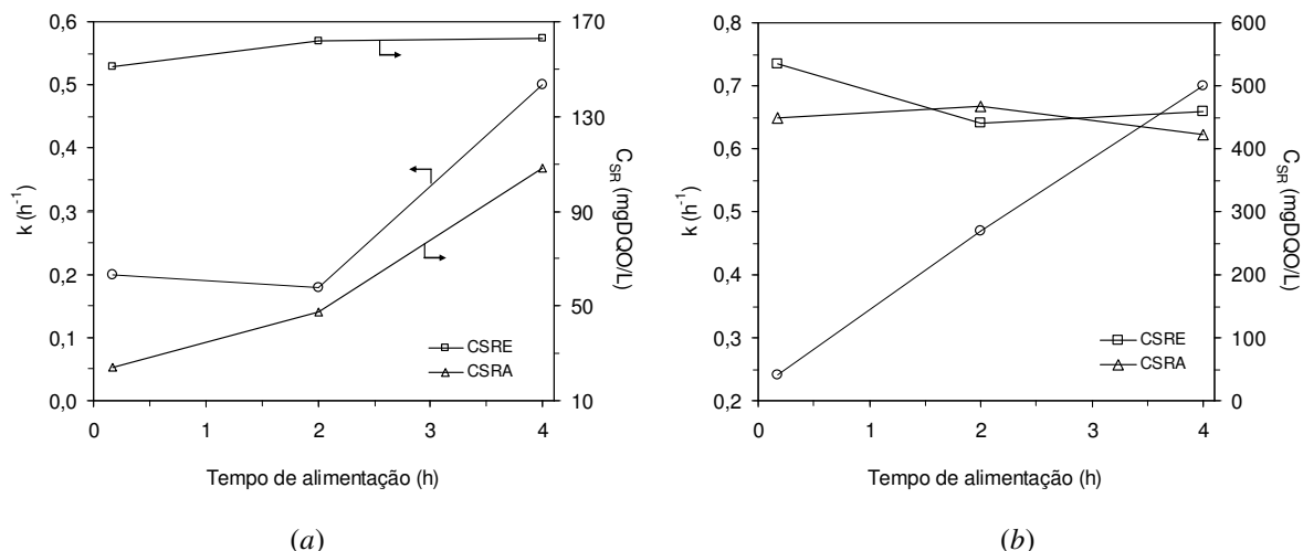
Figura 4.74 – Parâmetro cinético de primeira ordem e concentração residual ( C_{SRE} experimental e C_{SRA} ajustada) de matéria orgânica em função do tempo de alimentação de 10 minutos, 2 e 4 horas para as condições com (a) 1000 mgDQO/L e (b) 2000 mgDQO/L
