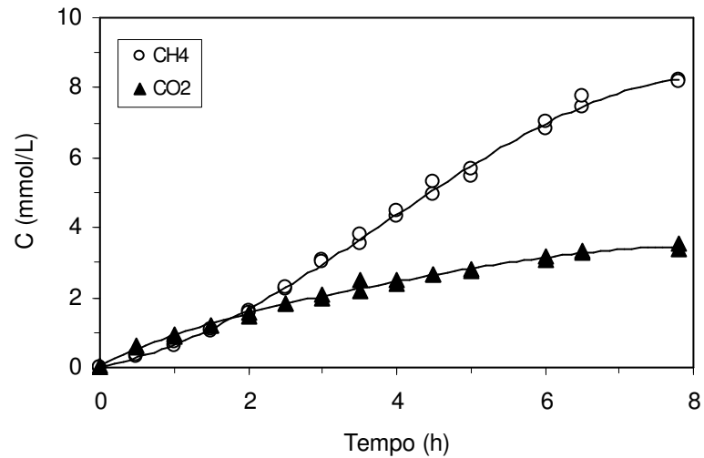
Figura 4. 39 – Perfis de concentração de metano e de gás carbônico na operação com 1000 mgDQO/L: alimentação em batelada alimentada durante 2 horas
