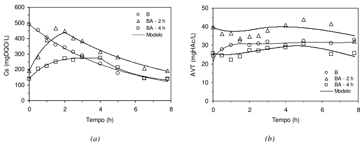
Figura 4.75 – Perfis de C_s (a) e de AVT (b) para as condições com 1000 mgDQO/L e alimentação em batelada (B), em batelada alimentada durante: 2 h (BA – 2 h) e 4 h (BA – 4 h)
