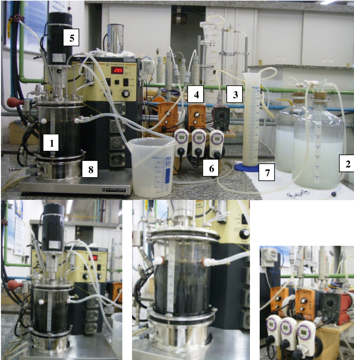
Figura 3. 2 – Fotografia do aparato experimental
