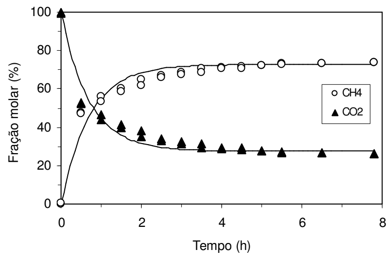
Figura 4. 20 – Perfis de fração molar de metano e de gás carbônico na operação com 1000 mgDQO/L
