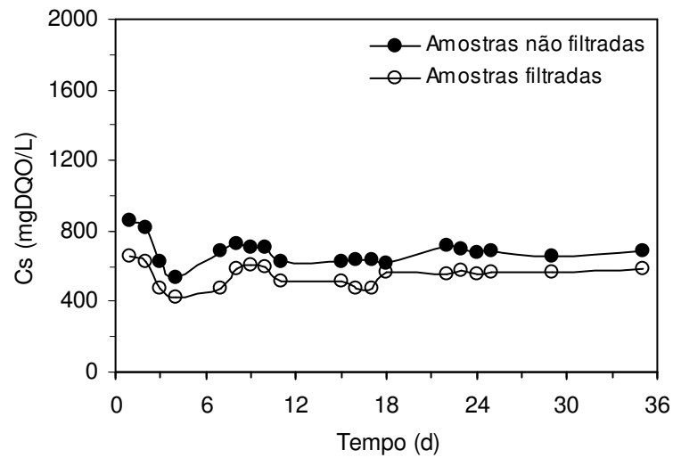
Figura 4.21 – Concentração de matéria orgânica na operação com 2000 mgDQO/L
