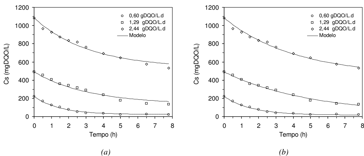
Figura 4. 65 – Perfis de concentração de matéria orgânica nas operações com 500 a 2000 mgDQO/L com alimentação em batelada ajuste: (a) Modelo I e (b) Modelo II
