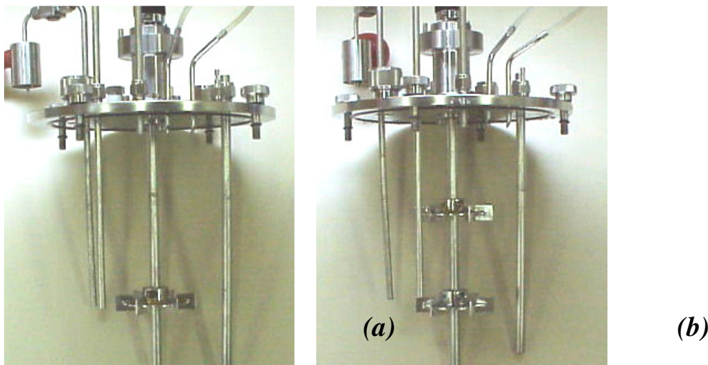
Figura 3.3 – Fotografias das configurações de impelidores tipo turbina no reator operado com agitação em batelada seqüencial (a) um impelidor e (b) dois impelidores
