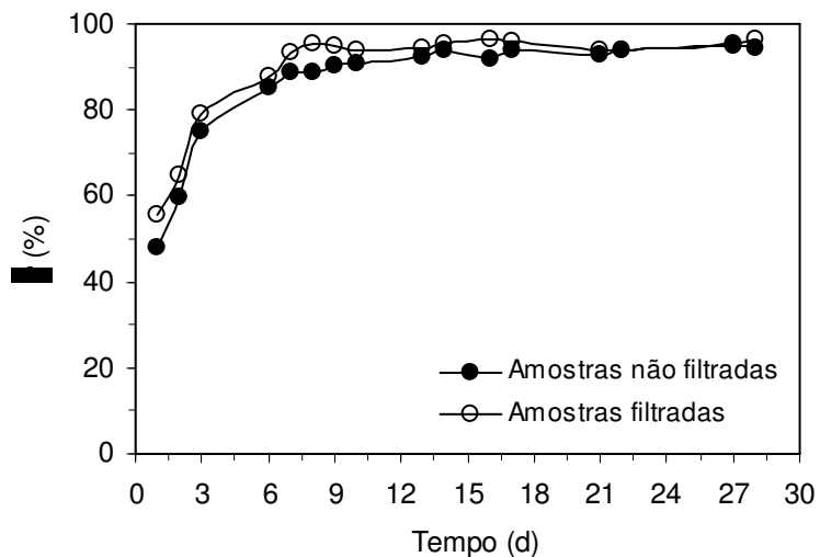
Figura 4. 2 – Eficiência de remoção de matéria orgânica na operação com 500 mgDQO/L
