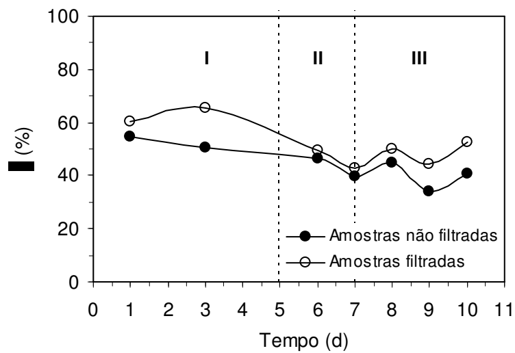
Figura 4. 31 – Eficiência de remoção de matéria orgânica na operação com 3000 mgDQO/L (I: 4,5 g NaHCO 3 /L; II: 6,0 g NaHCO 3 /L; III: 8,0 g NaHCO 3 /L)
