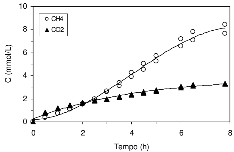
Figura 4. 47 – Perfis de concentração de metano e de gás carbônico na operação com 1000 mgDQO/L: alimentação em batelada alimentada durante 4 horas
