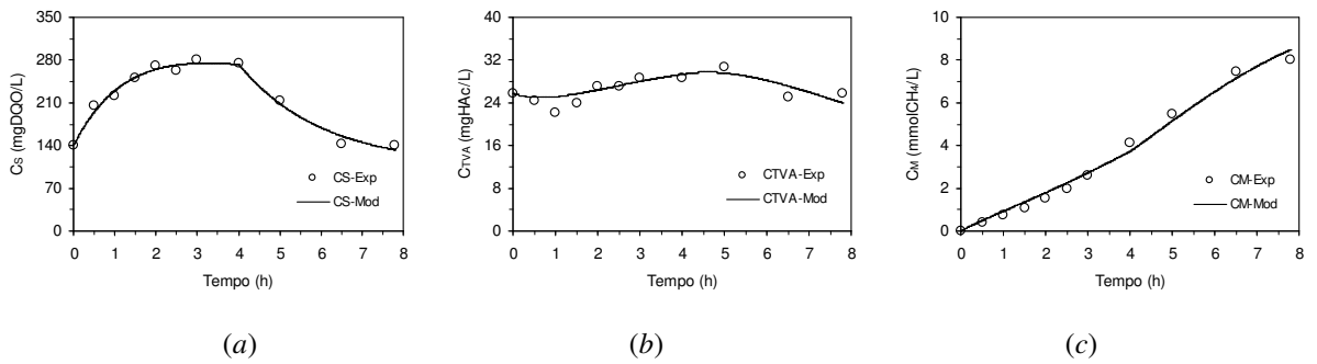
Figura 4. 71 – Perfil de (a) C_S , (b) C_{AVT} e (c) C_M na operação com 1000 mgDQO/L e alimentação em batelada alimentada durante 4 horas – Modelo III
