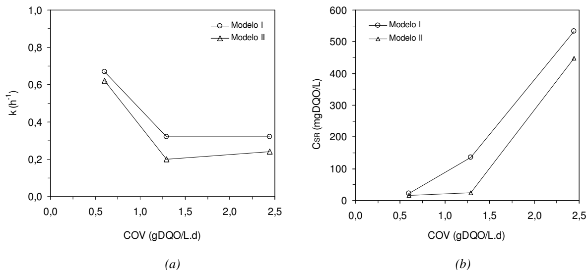
Figura 4.66 – Parâmetro cinético de primeira ordem (a) e concentração residual de matéria orgânica (b) em função da COV para o Modelo I e Modelo II
