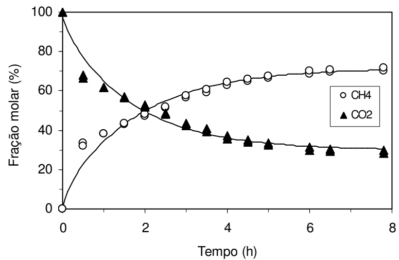
Figura 4. 48 – Perfis de fração molar de metano e de gás carbônico na operação com 1000 mgDQO/L: alimentação em batelada alimentada durante 4 horas
