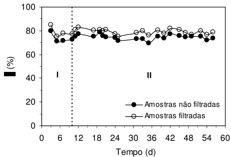
Figura 4. 50 – Eficiência de remoção de matéria orgânica na operação com 2000 mgDQO/L: alimentação em batelada (I) e alimentação em batelada alimentada durante 2 horas (II)
