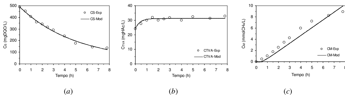
Figura 4. 68 – Perfil de (a) C_S , (b) C_{AVT} e (c) C_M na operação com 1000 mgDQO/L e alimentação em batelada – Modelo III
