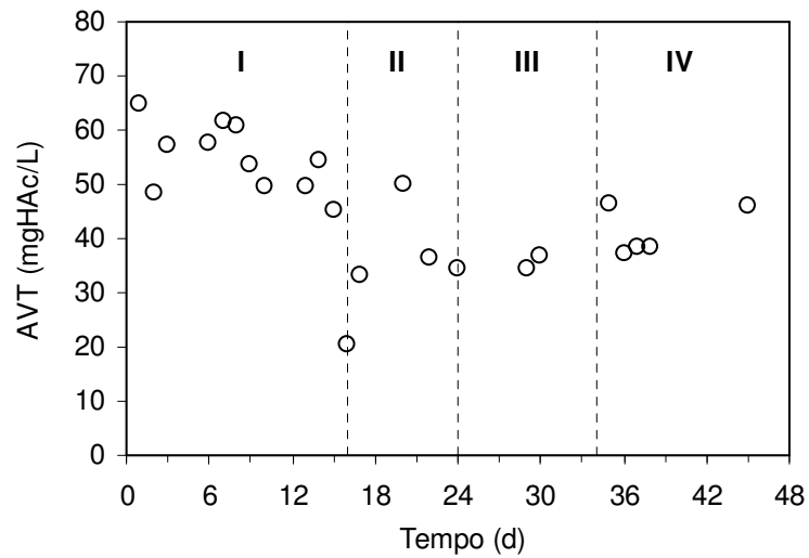
Figura 4. 12 – Ácidos voláteis totais (AVT) no efluente na operação com 1000 mgDQO/L (I: 0,5 g NaHCO 3 /L; II: 0,8 g NaHCO 3 /L; III: 1,0 g NaHCO 3 /L; IV: 1,5 gNaHCO 3 /L)
