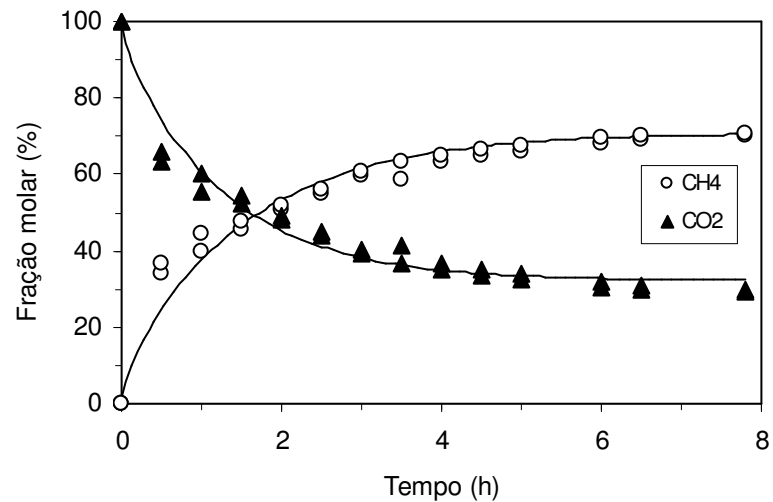
Figura 4. 40 – Perfis de fração molar de metano e de gás carbônico na operação com 1000 mgDQO/L: alimentação em batelada alimentada durante 2 horas
