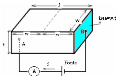
Figura 5.1 – Esquema de um material condutor de dimensões w (largura), l (comprimento), t (espessura)
