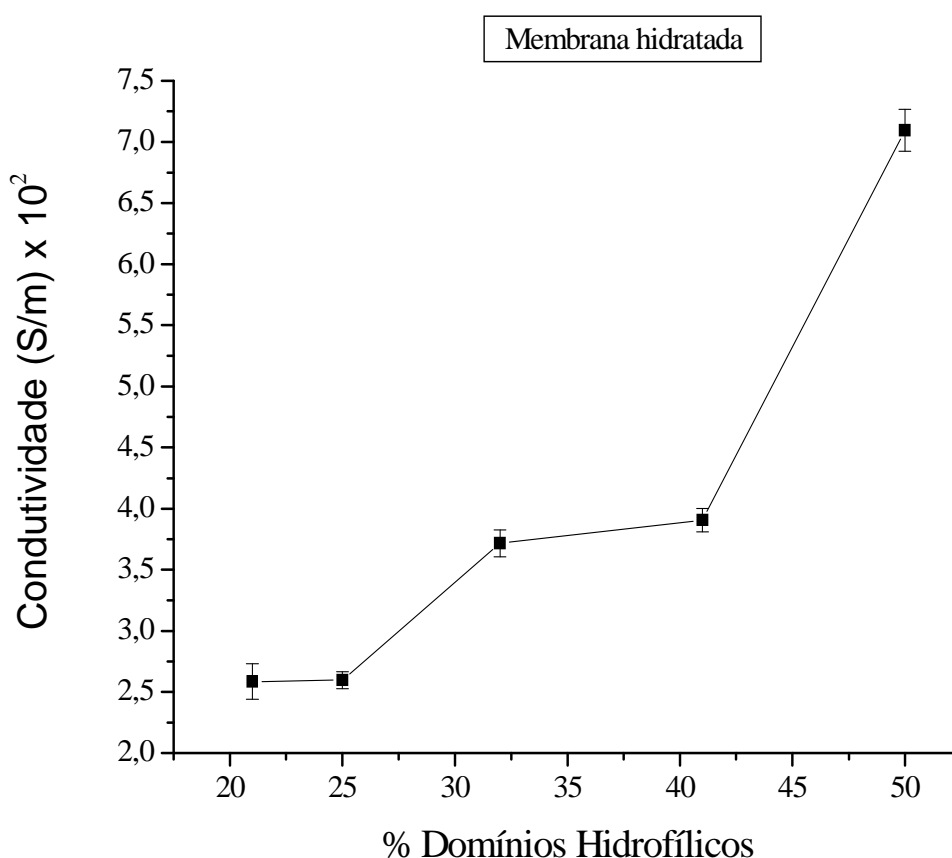
Figura 7.12 – Influência do percentual de domínios hidrofílicos na condutividade dos filmes obtidos no método de dois pontos com a membrana hidratada
