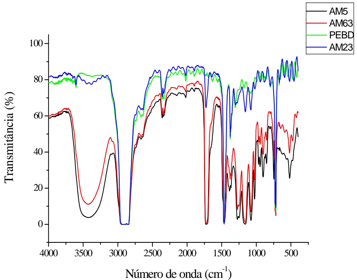
Figura 7.6 – Espectros vibracionais das membranas com 0%, 2%, 25% e 50% de domínios hidrofílicos
