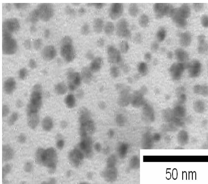
Figura 7.10 - Microscopia eletrônica de transmissão (TEM) dos domínios hidrofílicos na matriz orgânica após coloração com tetróxido de ósmio ( \text{OsO}_4 ).
