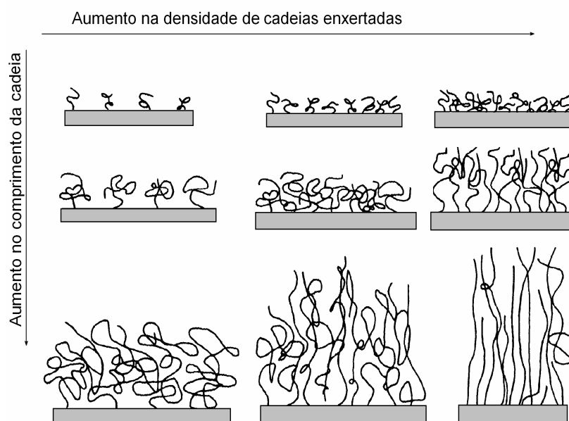
Figura 7.1 - Influência da densidade e comprimento de cadeias enxertadas na estrutura macromolecular do poli(HEMA).
