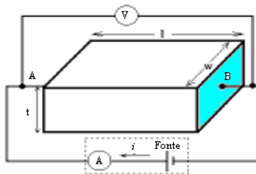
Figura 5.2 – Arranjo experimental para medida elétrica de dois pontos
