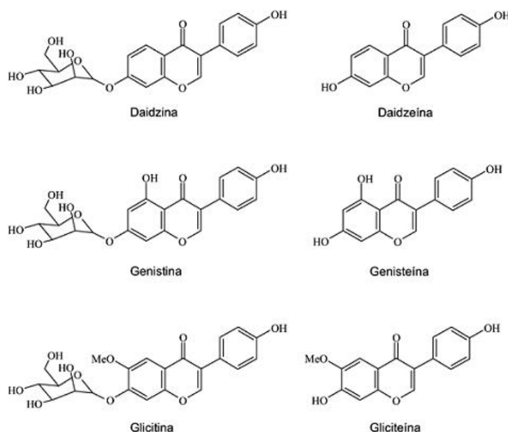
FIGURA 3 – ESTRUTURA QUÍMICA DOS GLICOSÍDEOS E AGLICONAS PRESENTES EM EXTRATOS DE SOJA.
