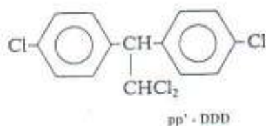
Figura 7: Estrutura química do p,p' - DDD.
