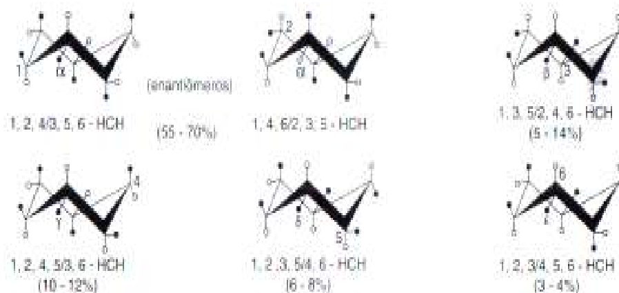
Figura 2: Isômeros do Hexaclorocicloexano.
