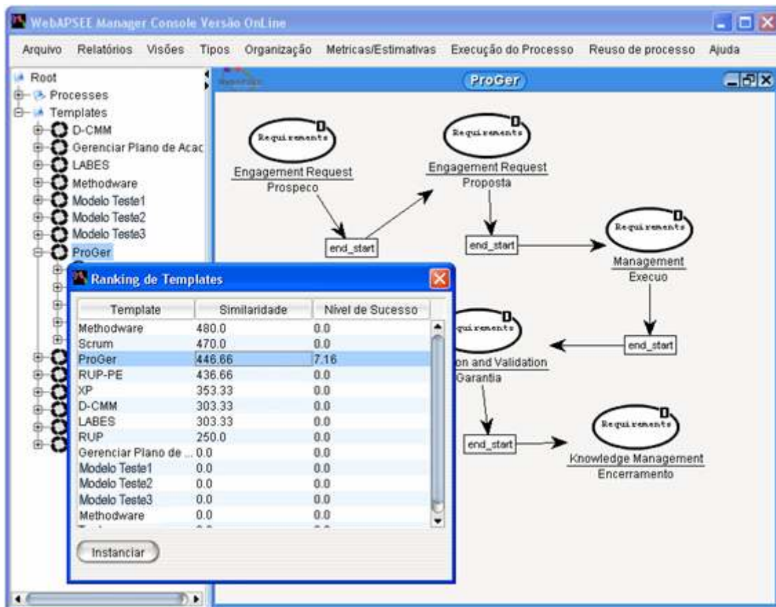
Figura 30 – Tela que exibe o resultado da recuperação de templates e visualização do template selecionado.
