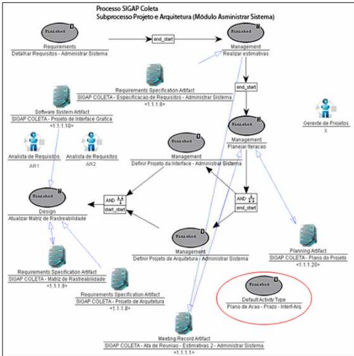
Figura 73 – Inclusão da atividade decomposta para ajuste de prazo no subprocesso Projeto e Arquitetura do módulo Administrar Sistema.
