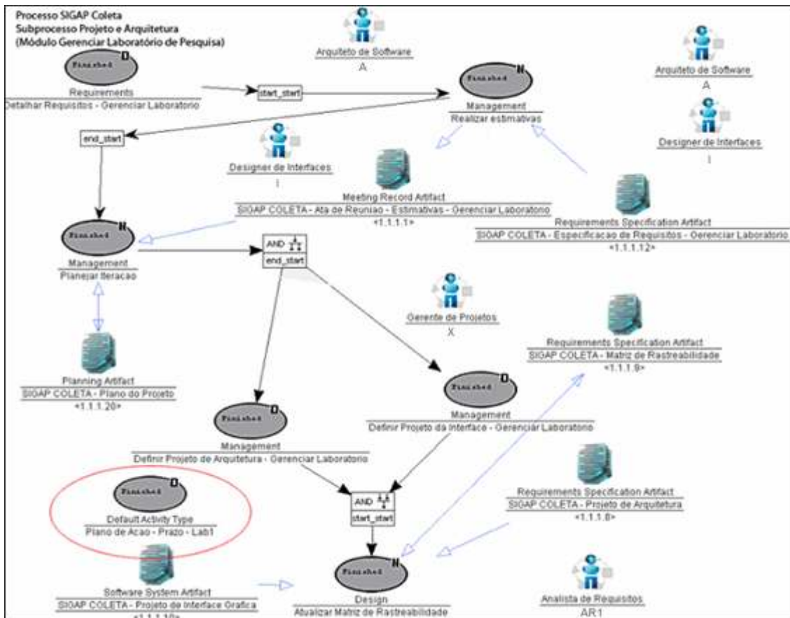
Figura 74 – Inclusão da atividade decomposta para ajuste de prazo no subprocesso Projeto e Arquitetura do módulo Gerenciar Laboratório de Pesquisa.
