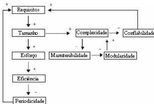
Figura 37 - Diagrama de causas e efeitos para a modelagem de um processo de software.
