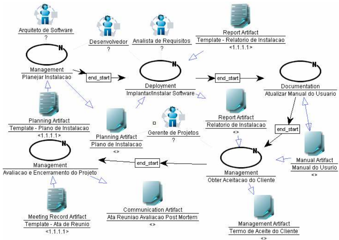
Figura 43 – Subprocesso Implantação e Encerramento do Projeto do Template LABES-UFPA .
