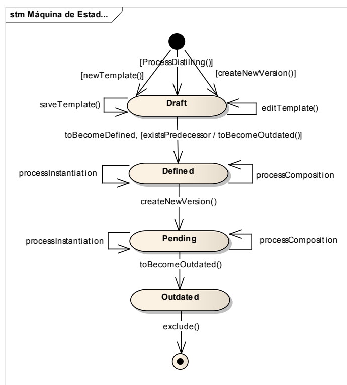
Figura 21 – Máquina de estados de um template .
