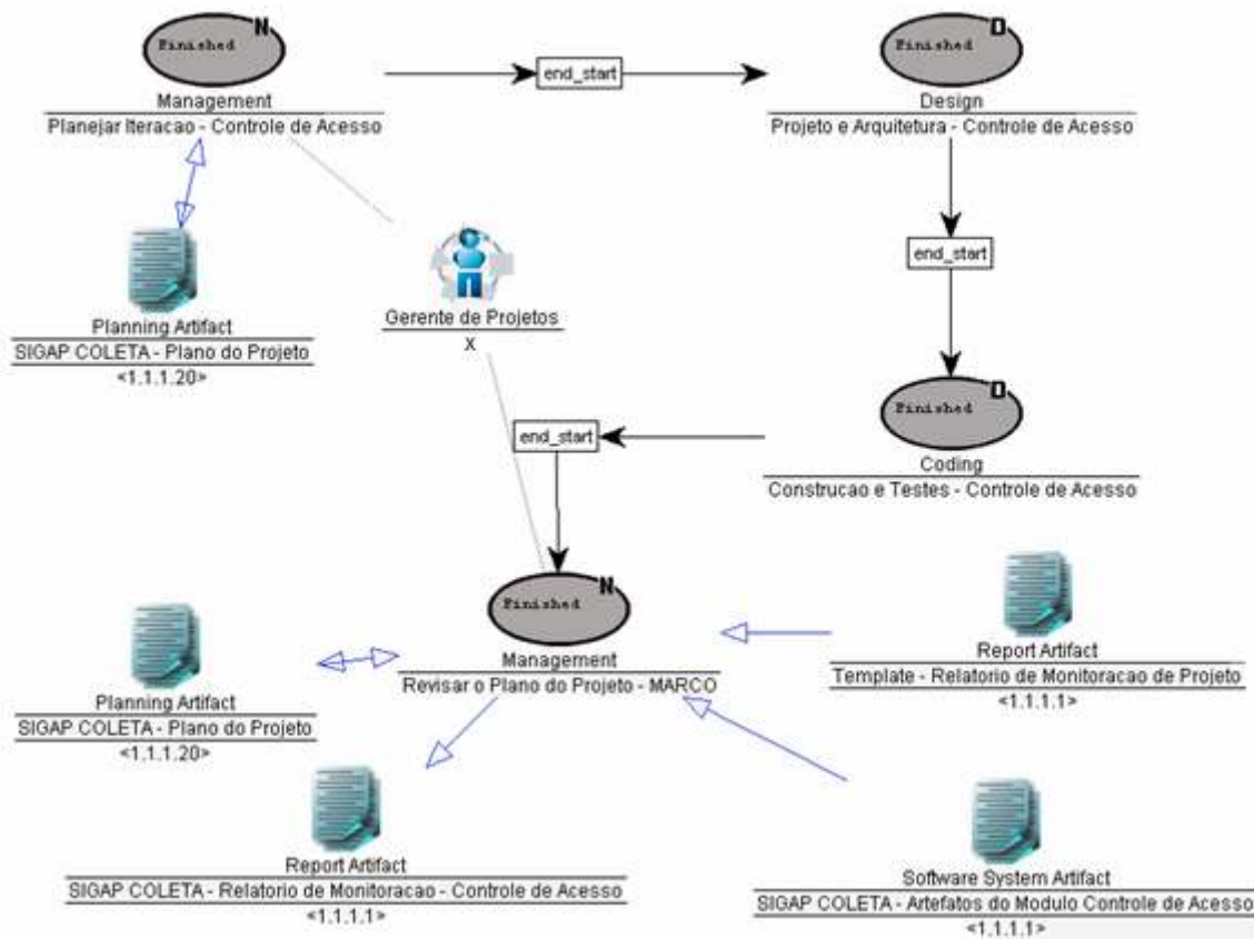
Figura 64 – Subprocesso Módulo Controle de Acesso do processo SIGAP Coleta.
