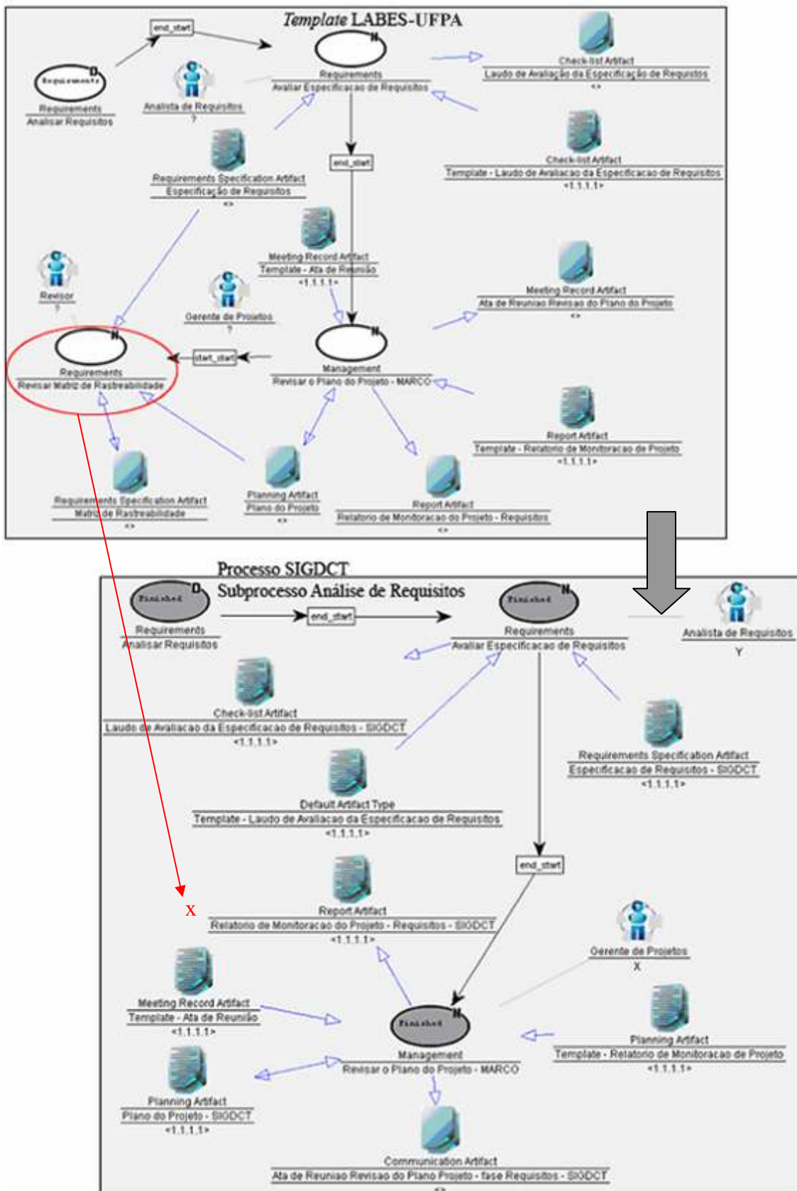
Figura 50 – Remoção da atividade Revisar matriz de rastreabilidade do subprocesso Análise de Requisitos .
