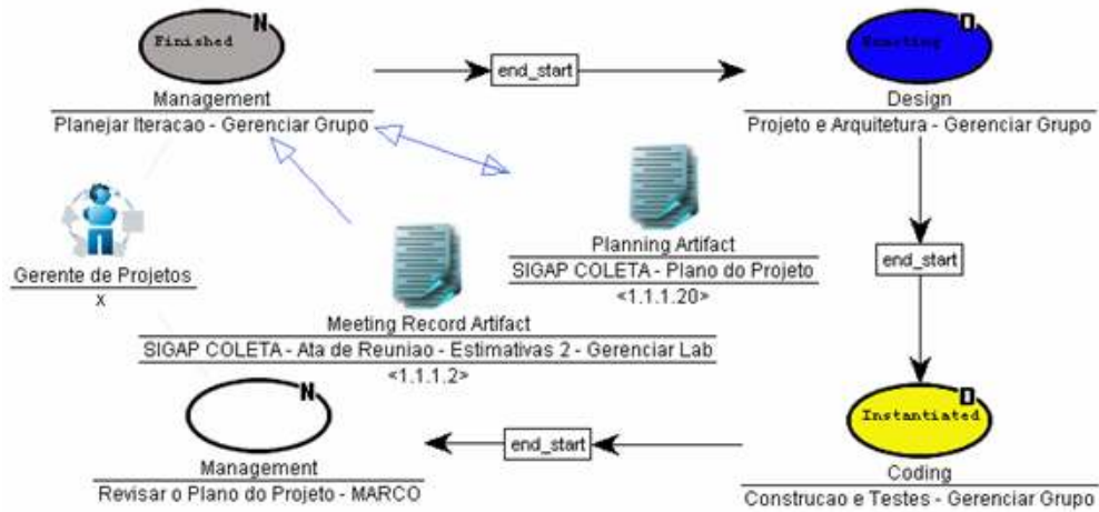
Figura 67 – Subprocesso Módulo Gerenciar Grupo de Pesquisa do processo SIGAP Coleta.
