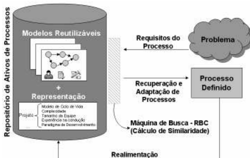
Figura 9 – Abordagem para gerenciamento de ativos de processos de software.
