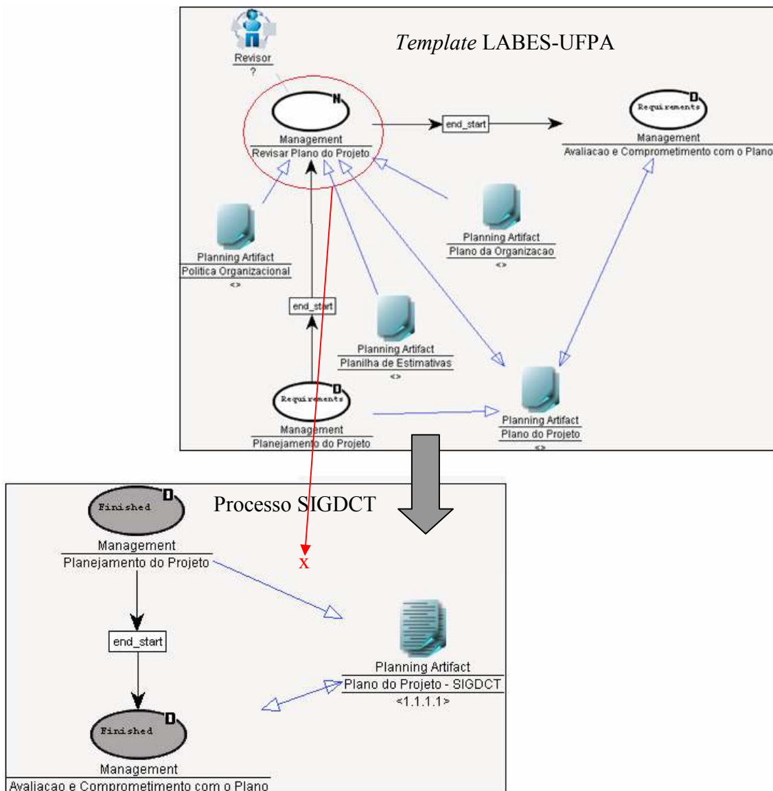
Figura 49 – Remoção da atividade Revisar Plano de Projeto do subprocesso Planejamento .
