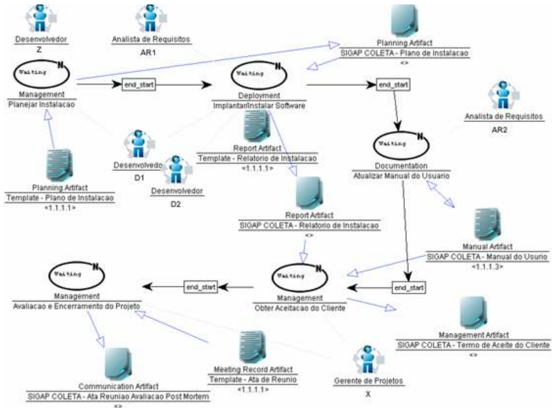
Figura 70 – Subprocesso Implantação e Encerramento do processo SIGAP Coleta.
