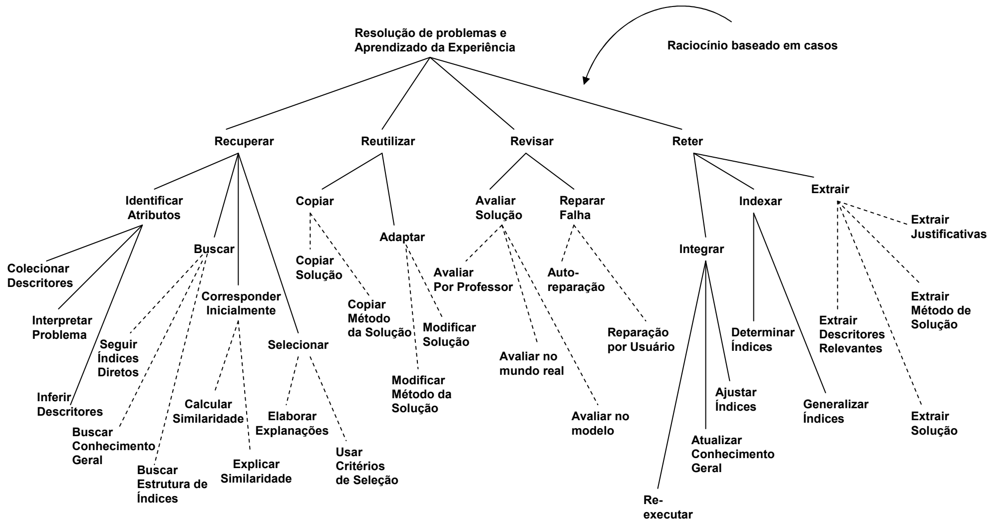
Figura 8 – Modelo de decomposição do método de tarefa de RBC [Aamodt e Plaza, 1994].
