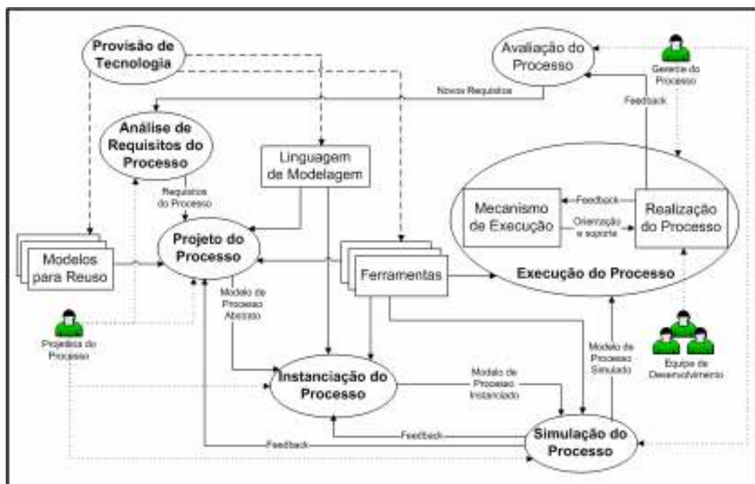
Figura 1 – Ciclo de Vida do Processo de Software.
