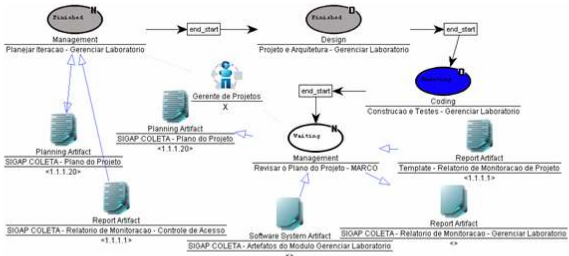
Figura 66 – Subprocesso Módulo Gerenciar Laboratório de Pesquisa do processo SIGAP Coleta.
