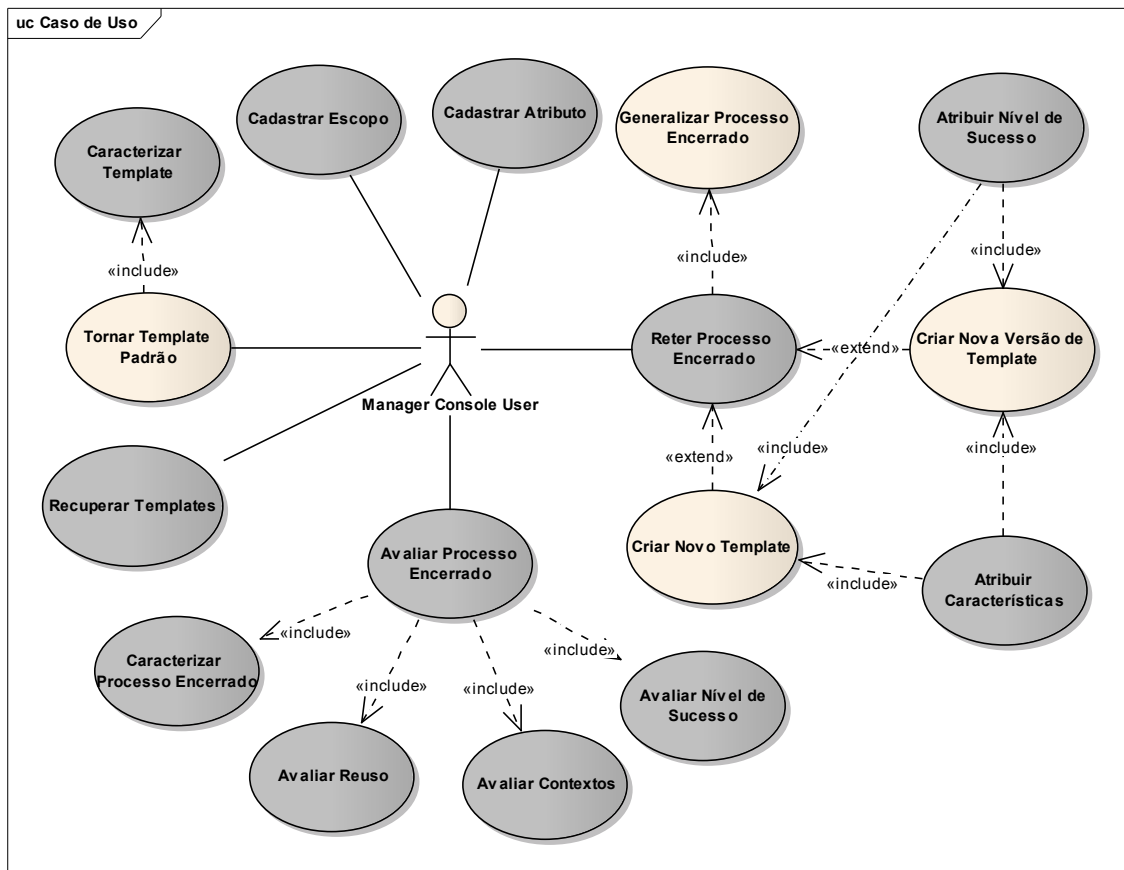
Figura 19 – Diagrama de casos de uso destacando as funcionalidades deste trabalho e sua relação com as funcionalidades pré-existentes no ambiente WebAPSEE-Pro.
