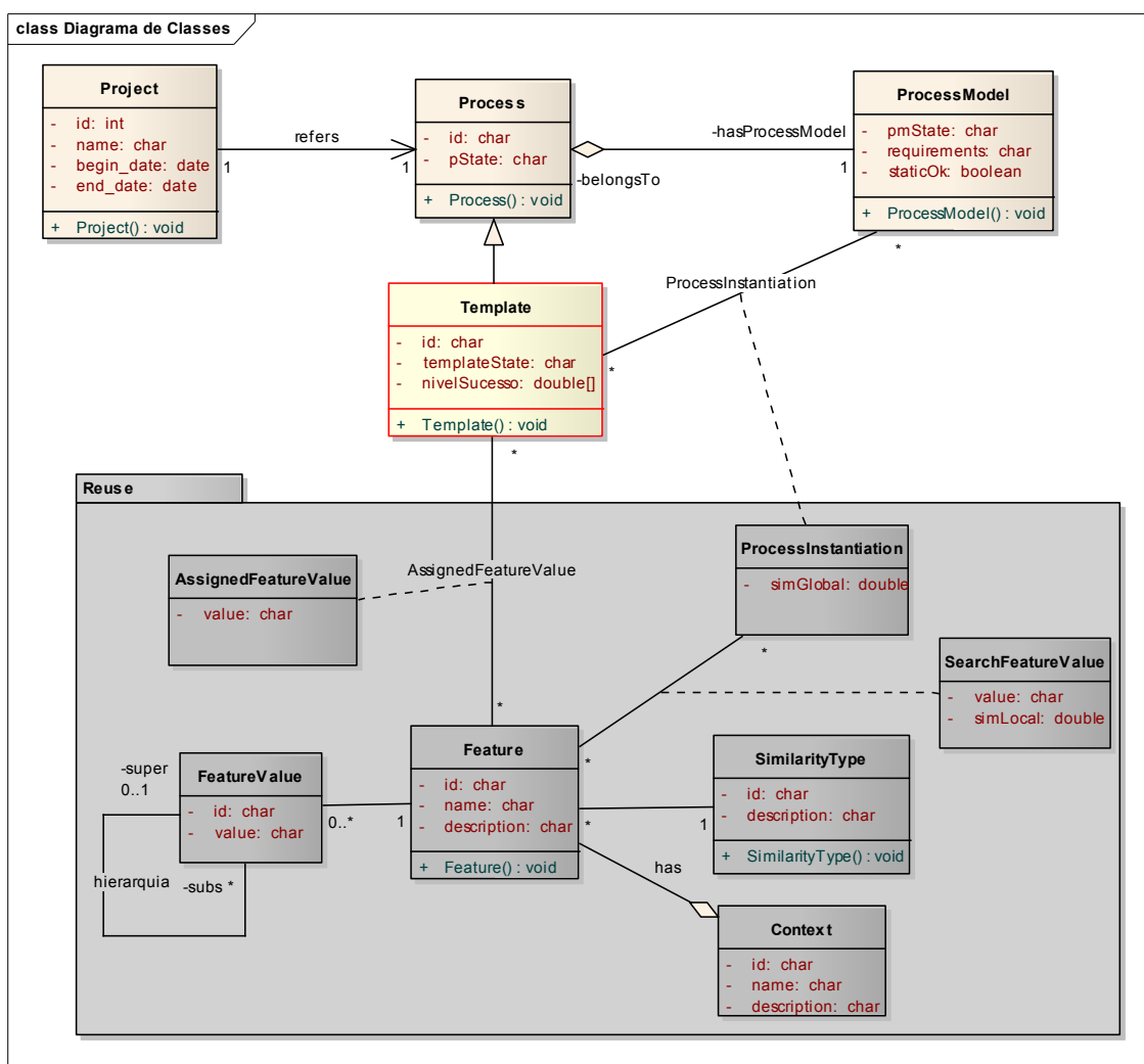
Figura 20 – Diagrama de classes apresentando as classes criadas e sua relação com as classes do modelo WebAPSEE-Pro.
