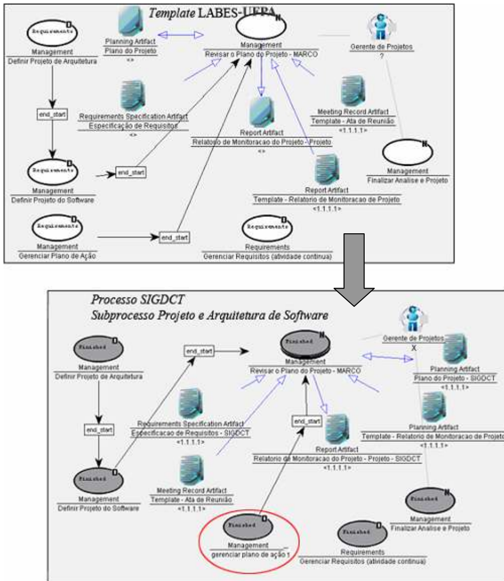
Figura 52 - Inclusão de subprocesso chamado “Gerenciar Plano de Ação 1” na fase de Projeto e Arquitetura do Software.
