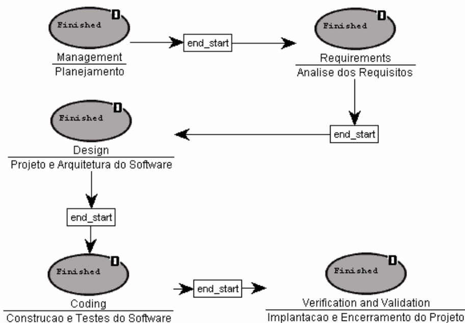
Figura 54 – Atividades decompostas do processo SIGDCT no estado finished .
