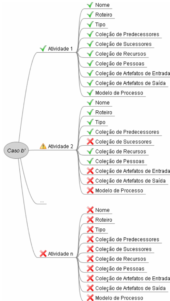
Figura 18 – Mapeamento dos componentes reutilizados e não reutilizados do caso a no caso b' .
