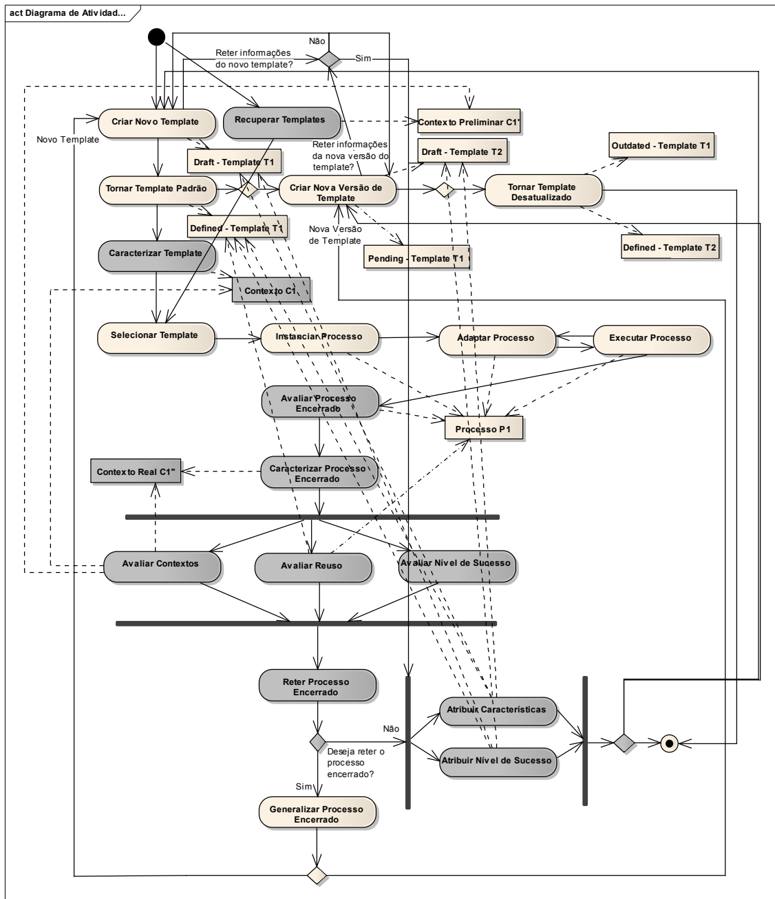
Figura 22 – Diagrama de atividades destacando as funcionalidades deste trabalho.
