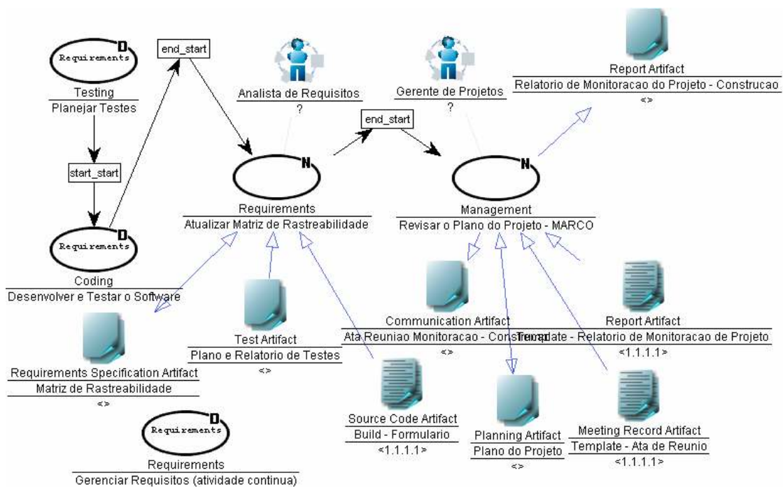
Figura 42 – Subprocesso Construção e Testes do Software do template LABES-UFPA.
