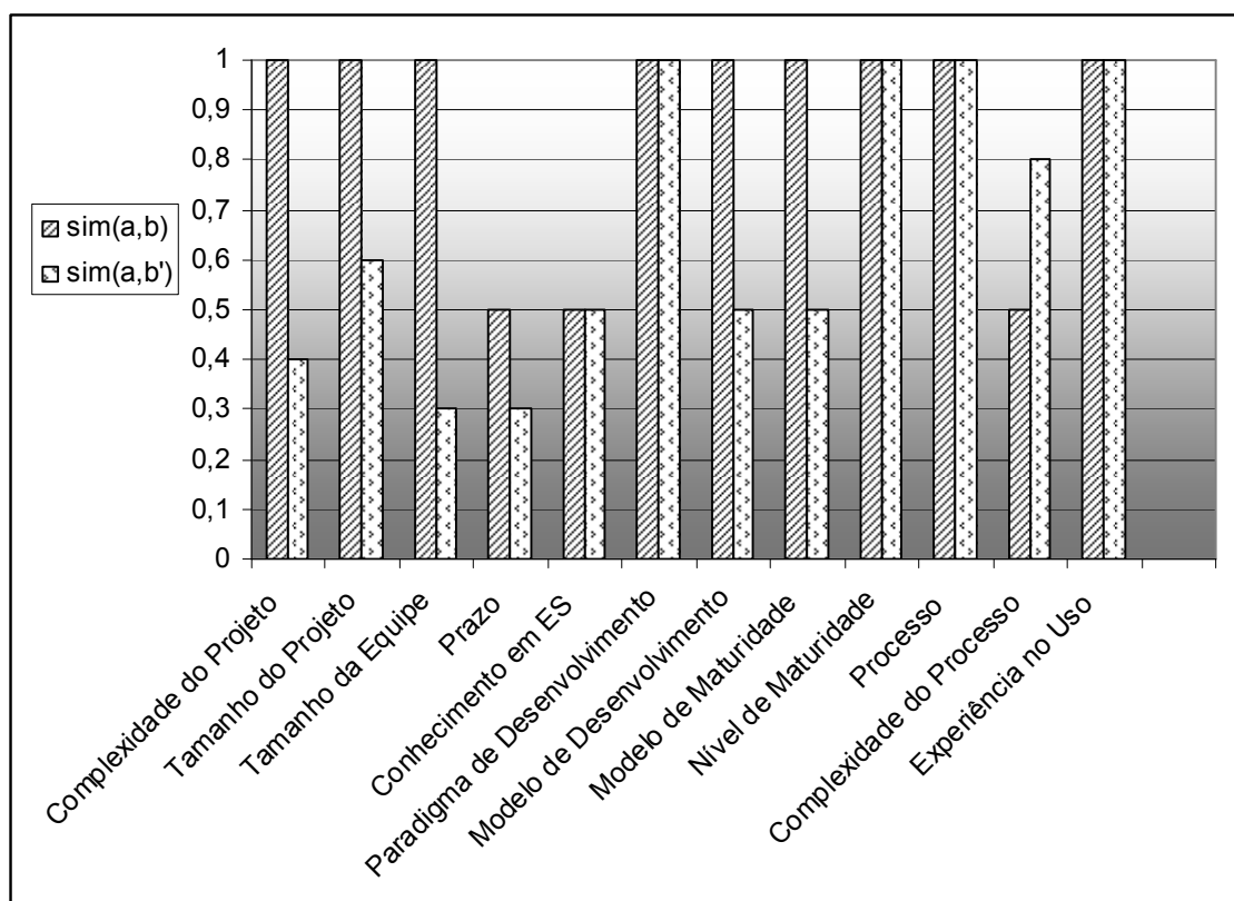
Figura 17 – Exemplo de um gráfico de variação das similaridades locais dos atributos nos contextos preliminar e real.
