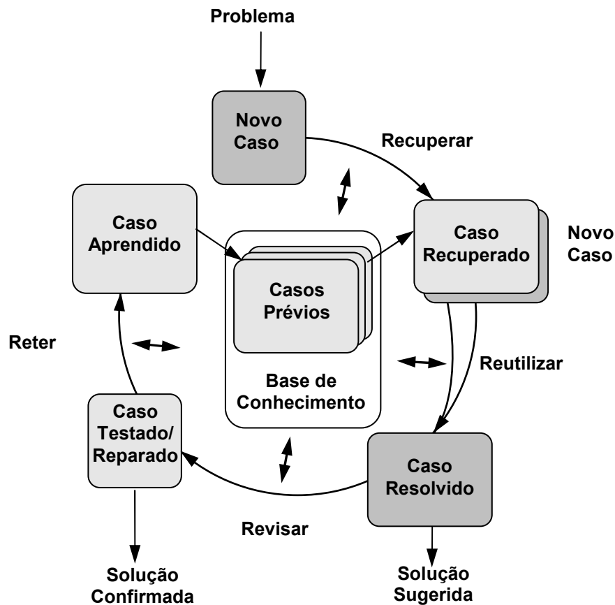
Figura 7 – Ciclo de vida do RBC [Aamodt e Plaza, 1994].
