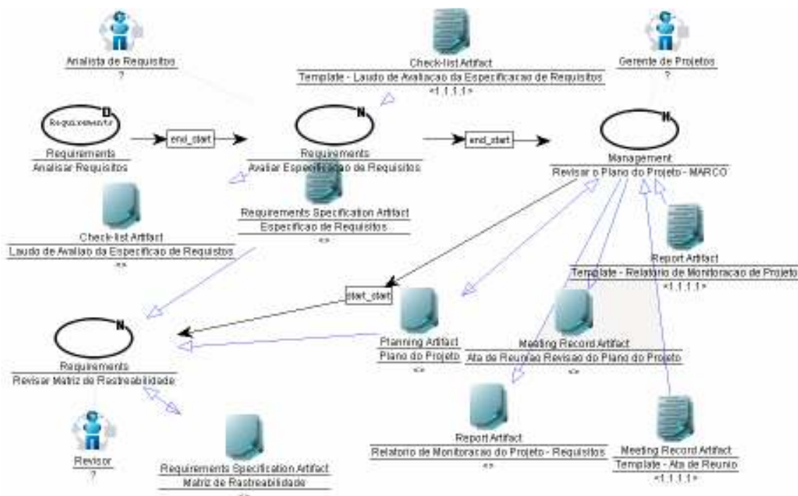
Figura 40 – Subprocesso Análise dos Requisitos do template LABES-UFPA.
