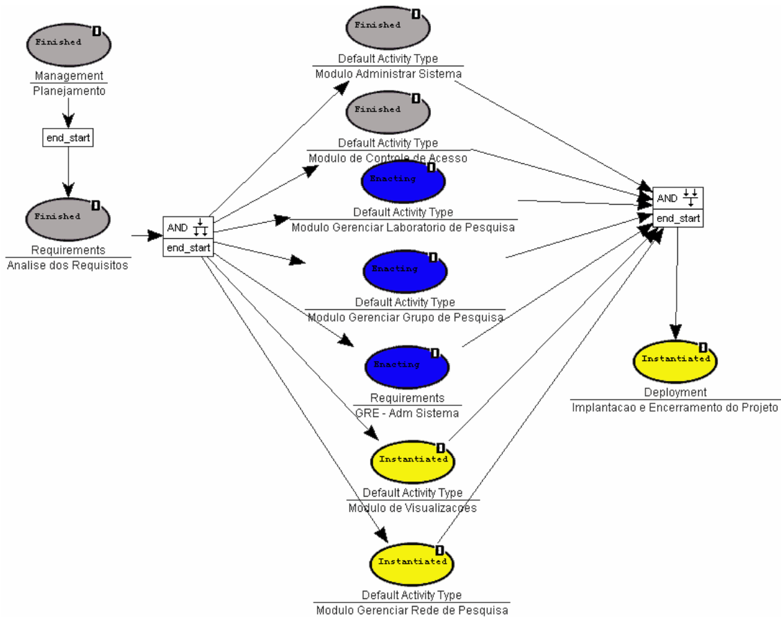
Figura 61 – Processo SIGAP Coleta em andamento [Lemos et al., 2009].
