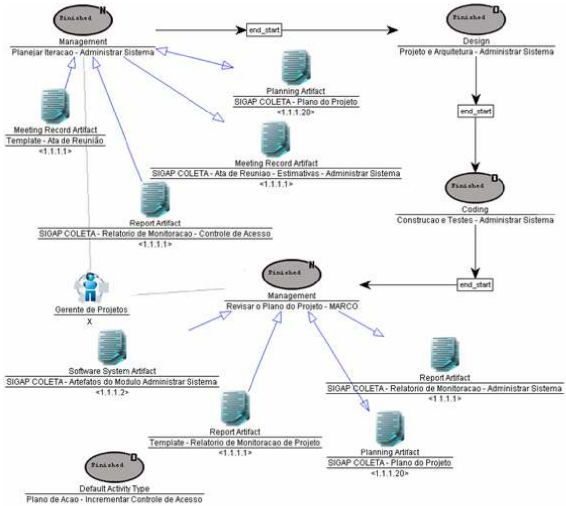
Figura 65 – Subprocesso Módulo Administrar Sistema do processo SIGAP Coleta.
