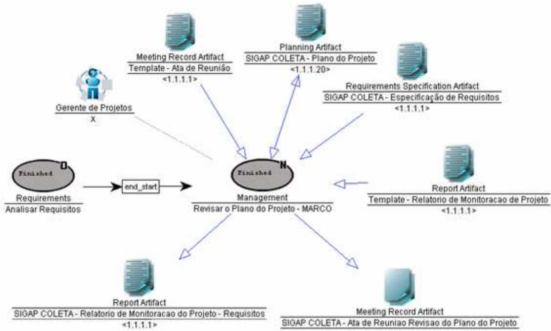
Figura 63 – Subprocesso Análise dos Requisitos do processo SIGAP Coleta.
