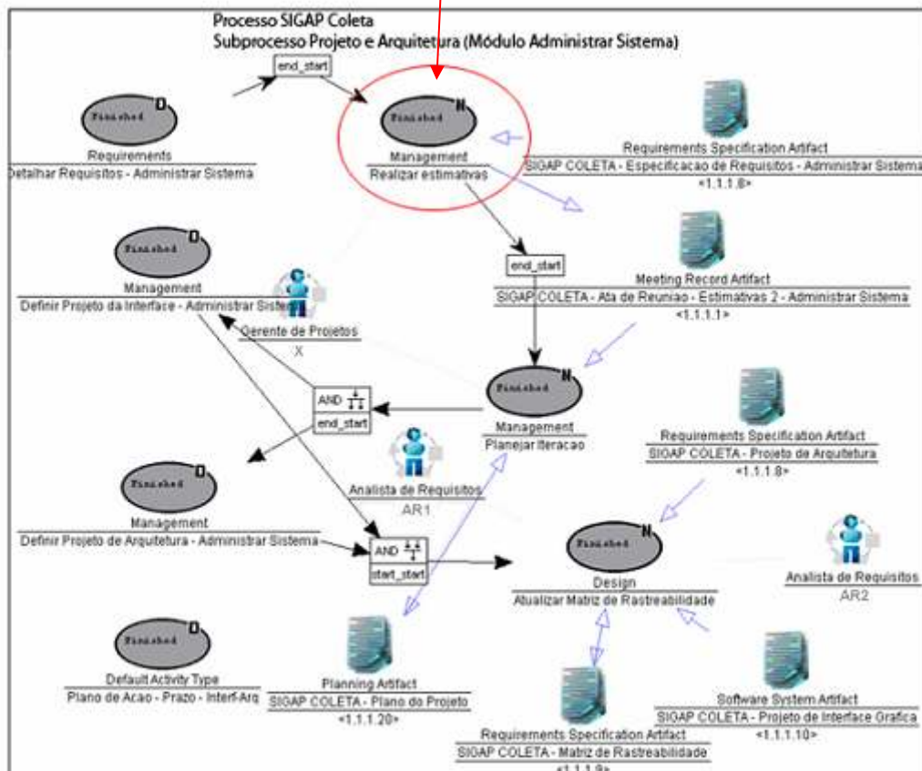
Figura 72 – Inclusão da atividade Realizar Estimativas após o detalhamento dos requisitos.
