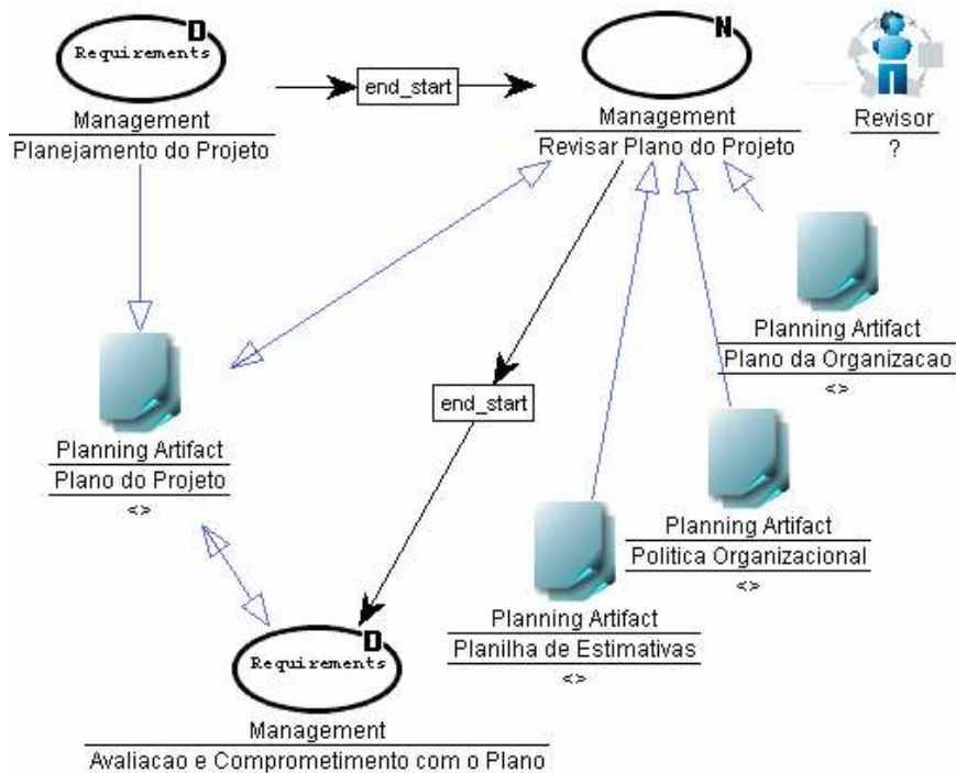
Figura 39 – Subprocesso Planejamento do template LABES-UFPA.
