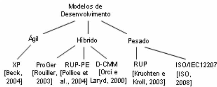
Figura 13 - Taxonomia para o atributo Modelo de Desenvolvimento (Processo).
