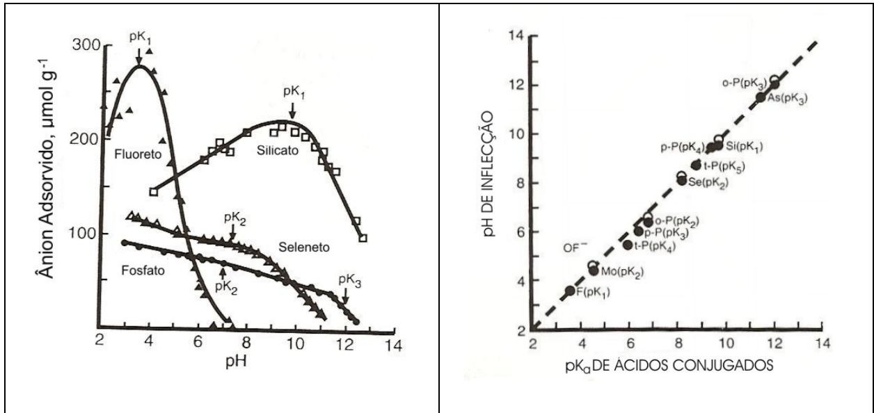
Figura 10: Adsorção de ânions em goethita. Modificado de Hingston et al. (1972).
