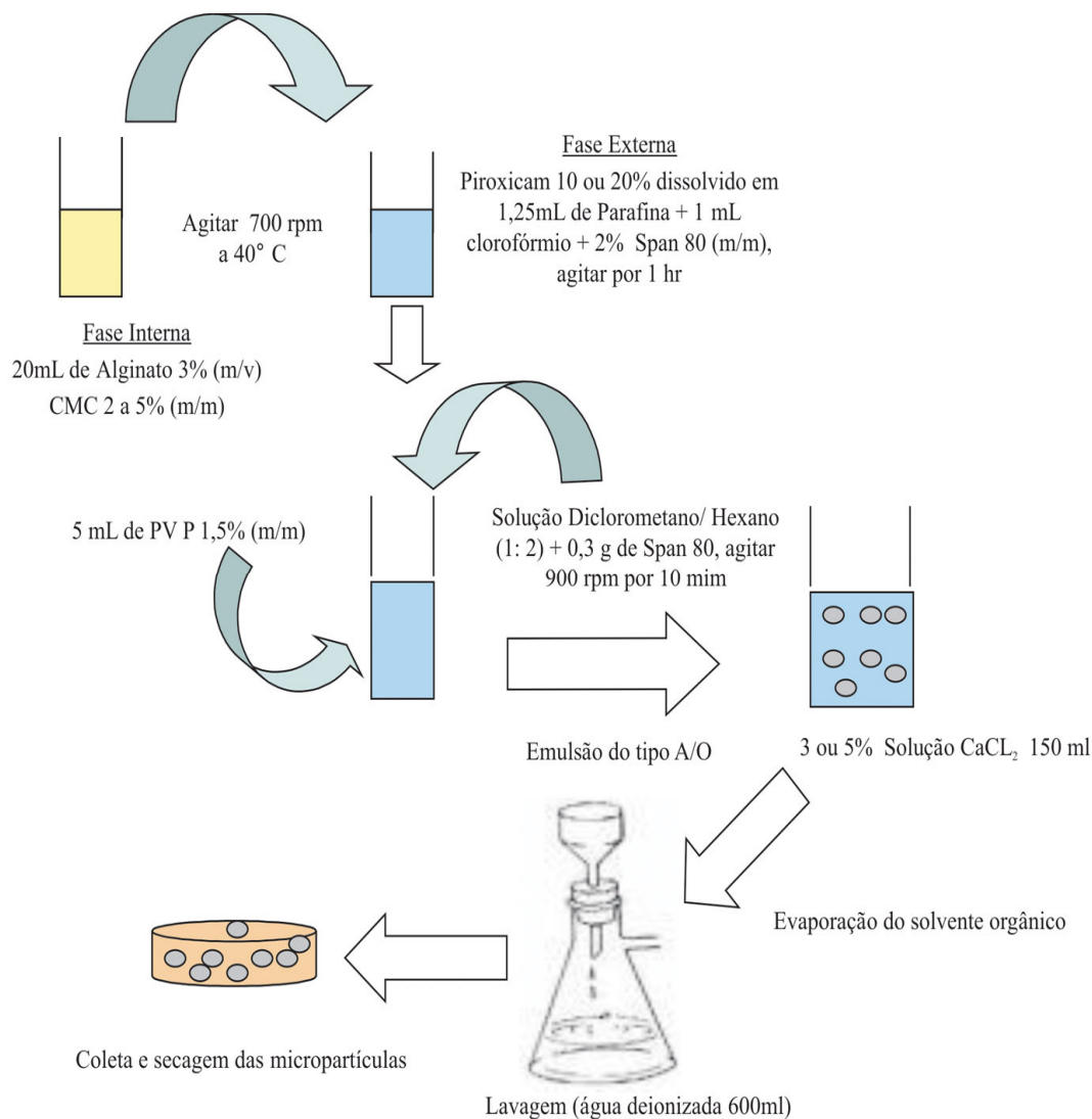
Figura 10 - Esquema de obtenção das micropartículas Alg/CMC pelo método de emulsão-reticulação.
