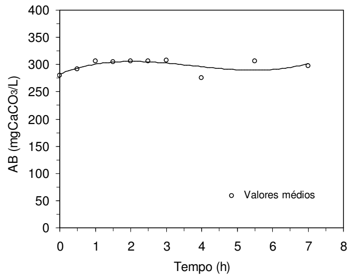
Figura 4.17 – Perfil de alcalinidade a bicarbonato (AB) na operação com 1000 mgDQO/L
