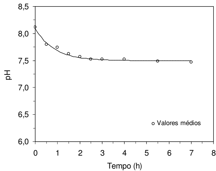
Figura 4.18 – Perfil da variação de pH na operação com 1000 mgDQO/L
