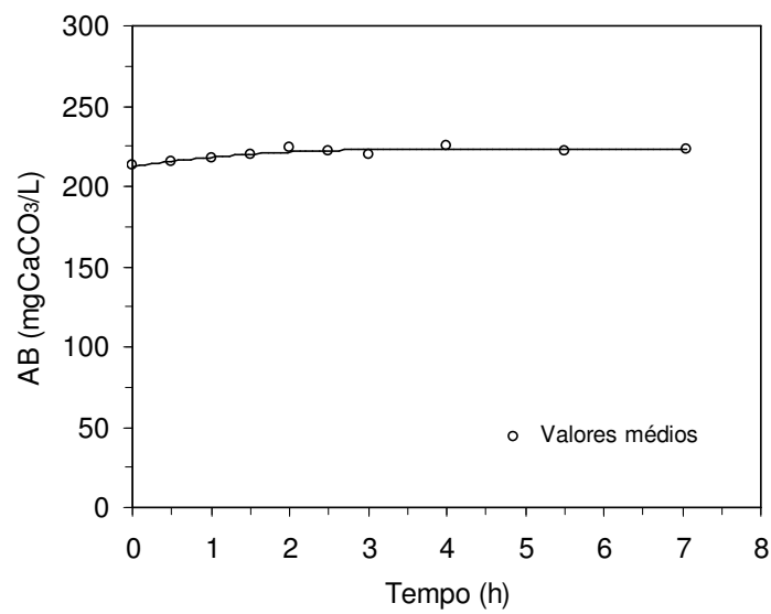
Figura 4.5 – Perfil de alcalinidade a bicarbonato (AB) na operação com 500 mgDQO/L
