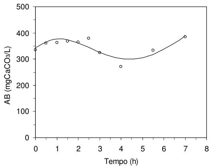
Figura 4.35 – Perfil de alcalinidade a bicarbonato (AB) na operação com 2000 mgDQO/L ao longo do ciclo seguinte à aplicação de carga de choque com 4000 mgDQO/L
