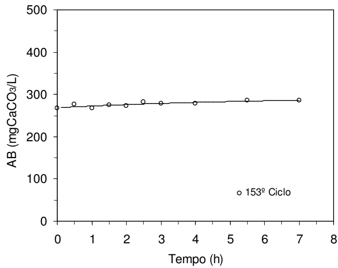
Figura 4.49 – Perfil de alcalinidade a bicarbonato (AB) na operação com 2000 mgDQO/L e alimentação em batelada seguida de batelada alimentada durante 4 horas ao longo do ciclo seguinte à aplicação de carga de choque com 4000 mgDQO/L
