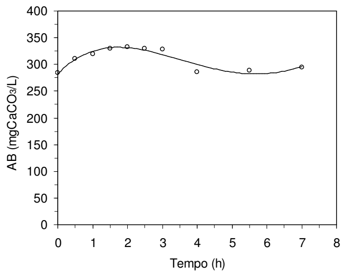
Figura 4.23 – Perfil de alcalinidade a bicarbonato (AB) na operação com 1000 mgDQO/L ao longo do ciclo seguinte à aplicação de carga de choque com 2000 mgDQO/L
