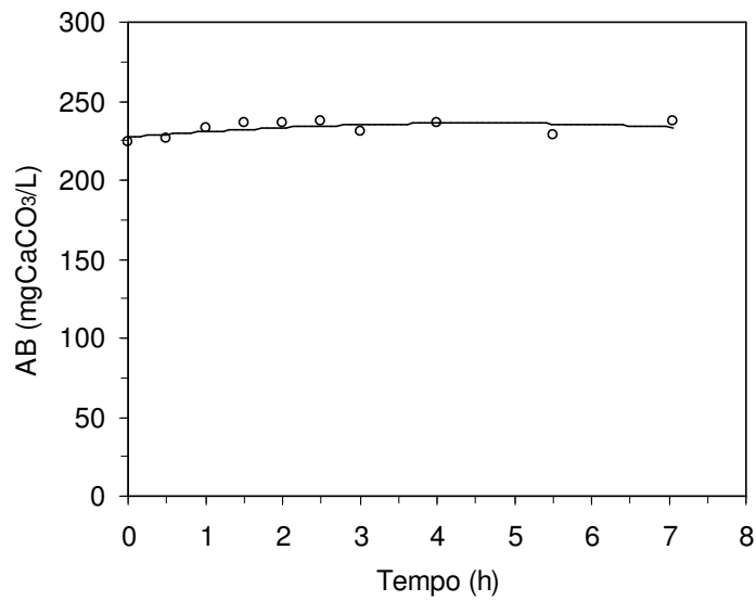
Figura 4.11 – Perfil de alcalinidade a bicarbonato (AB) na operação com 500 mgDQO/L ao longo do ciclo seguinte à aplicação de carga de choque com 1000 mgDQO/L
