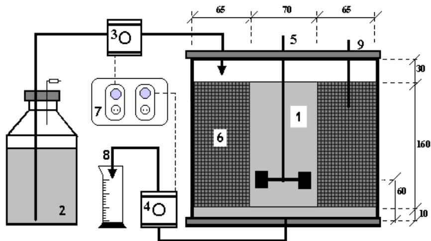
Figura 3.1 – Esquema do reator anaeróbio operado em batelada seqüencial contendo biomassa imobilizada AnSBBR [(Dimensões em milímetros): (1) Tanque de reação, (2) Água residuária, (3) Bomba de alimentação, (4) Bomba de descarga, (5) Agitador mecânico, (6) Cesto contendo espumas e biomassa imobilizada, (7) Temporizadores, (8) Efluente tratado e (9) Termômetro]
